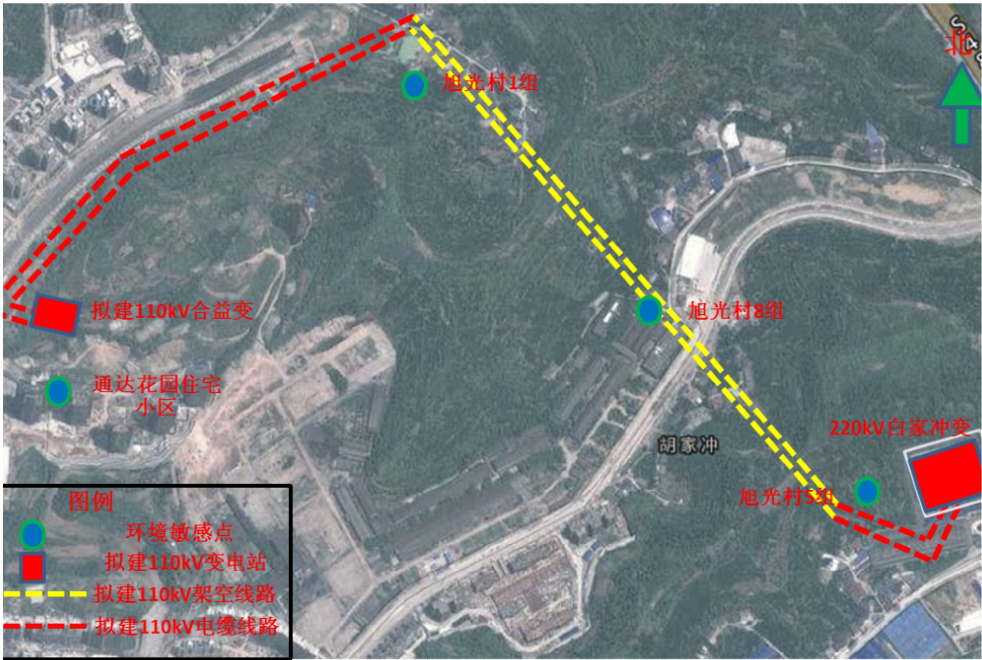
附图3 宜昌合益110kV输变电工程路径走向示意图
