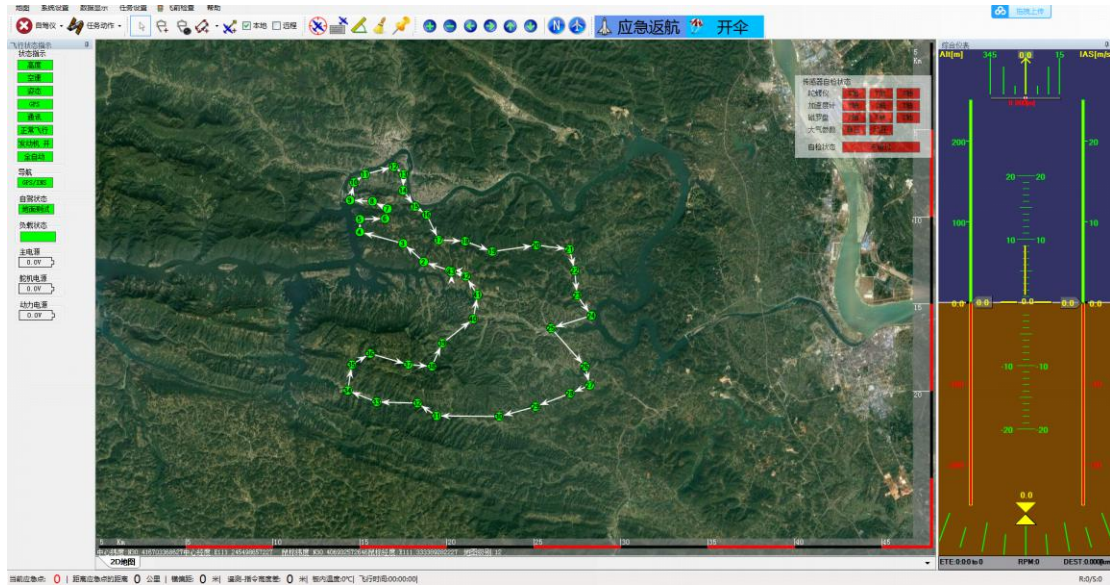
图 2：飞行航线图
