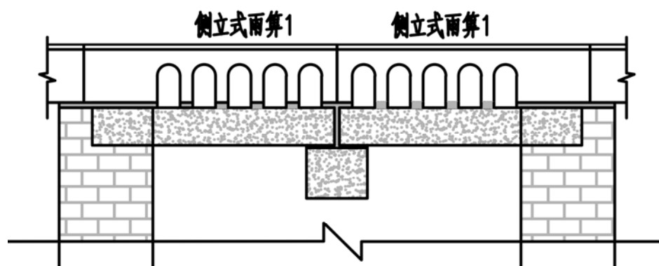
侧立式双篦雨水口安装示例
