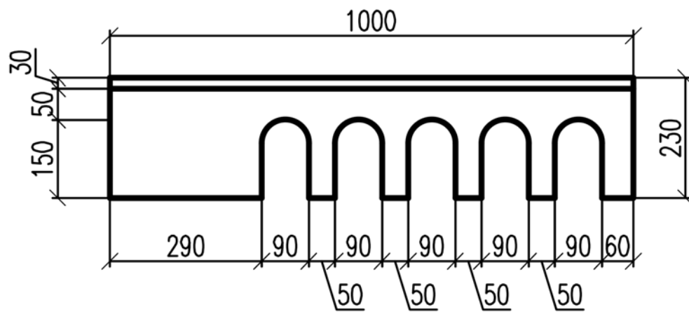
侧立式雨篦 1 大样图
