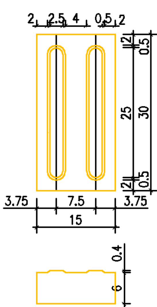
行进块盲道砖尺寸图
