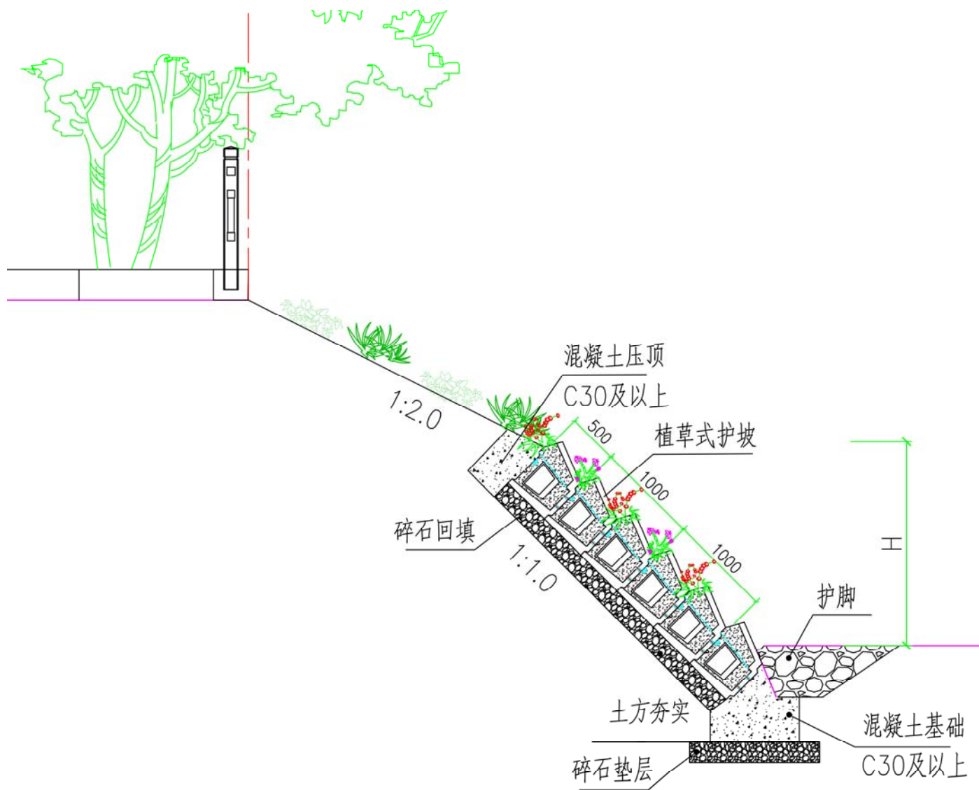
植草式生态护坡砌块安装剖面图
