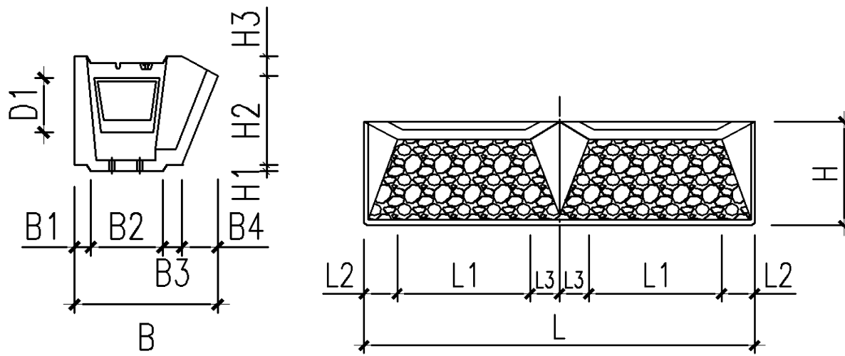
植草式生态护坡砌块尺寸图
