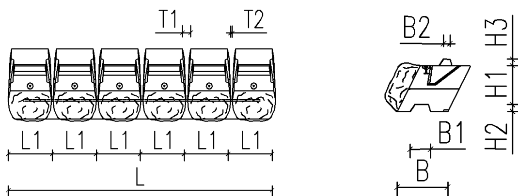
生态石挡土墙护坡砌块尺寸图
