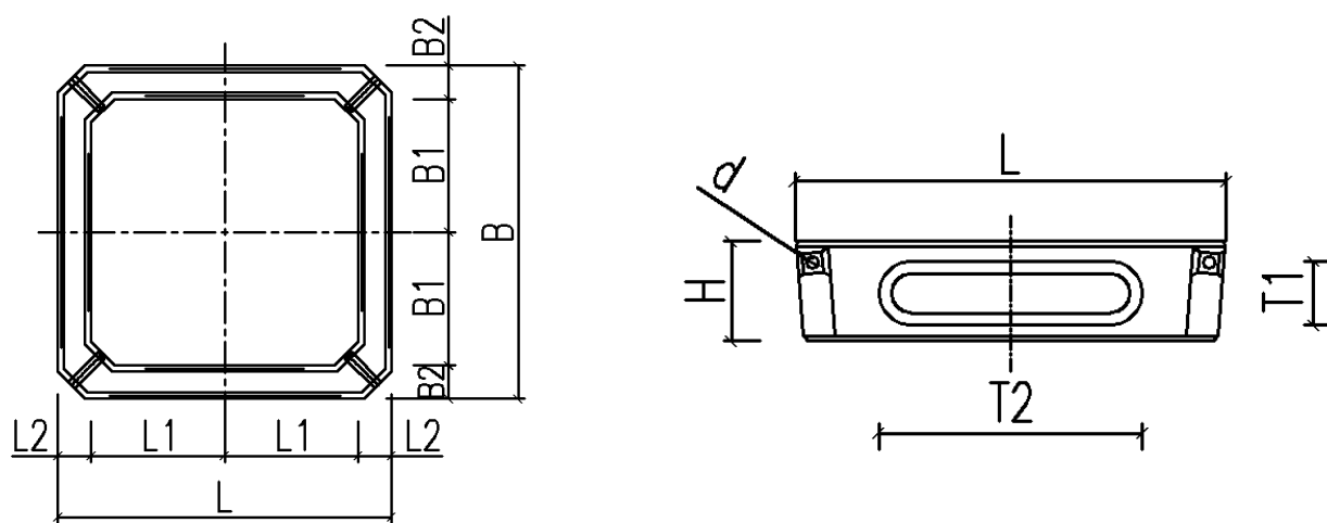
平铺式生态护坡砌块尺寸图
