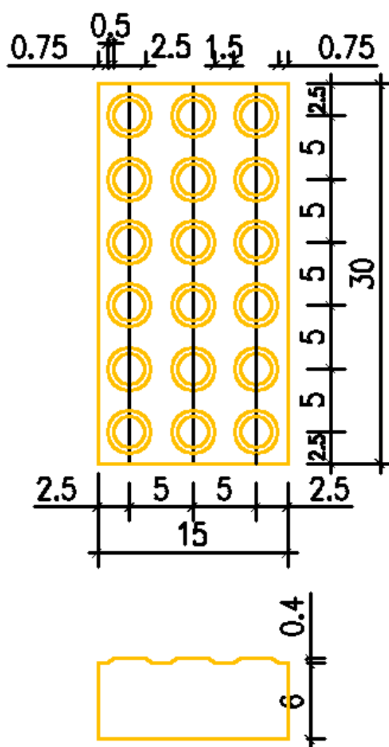
提示块盲道砖尺寸图
