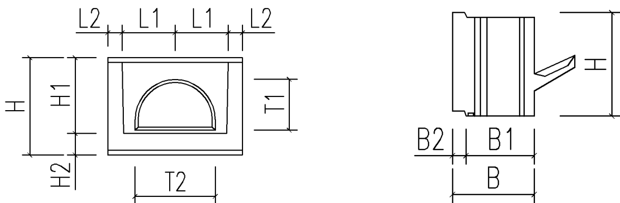
格构式挡土墙护坡砌块尺寸图
