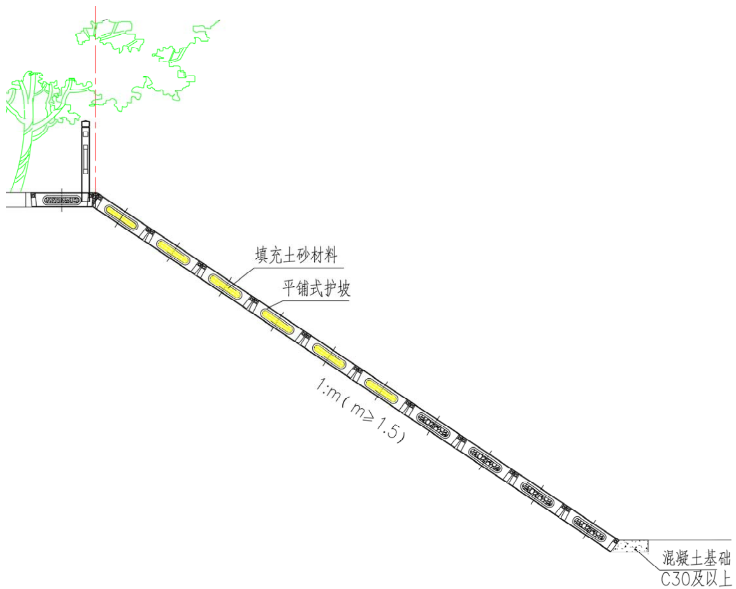
平铺式生态护坡砌块安装剖面图
