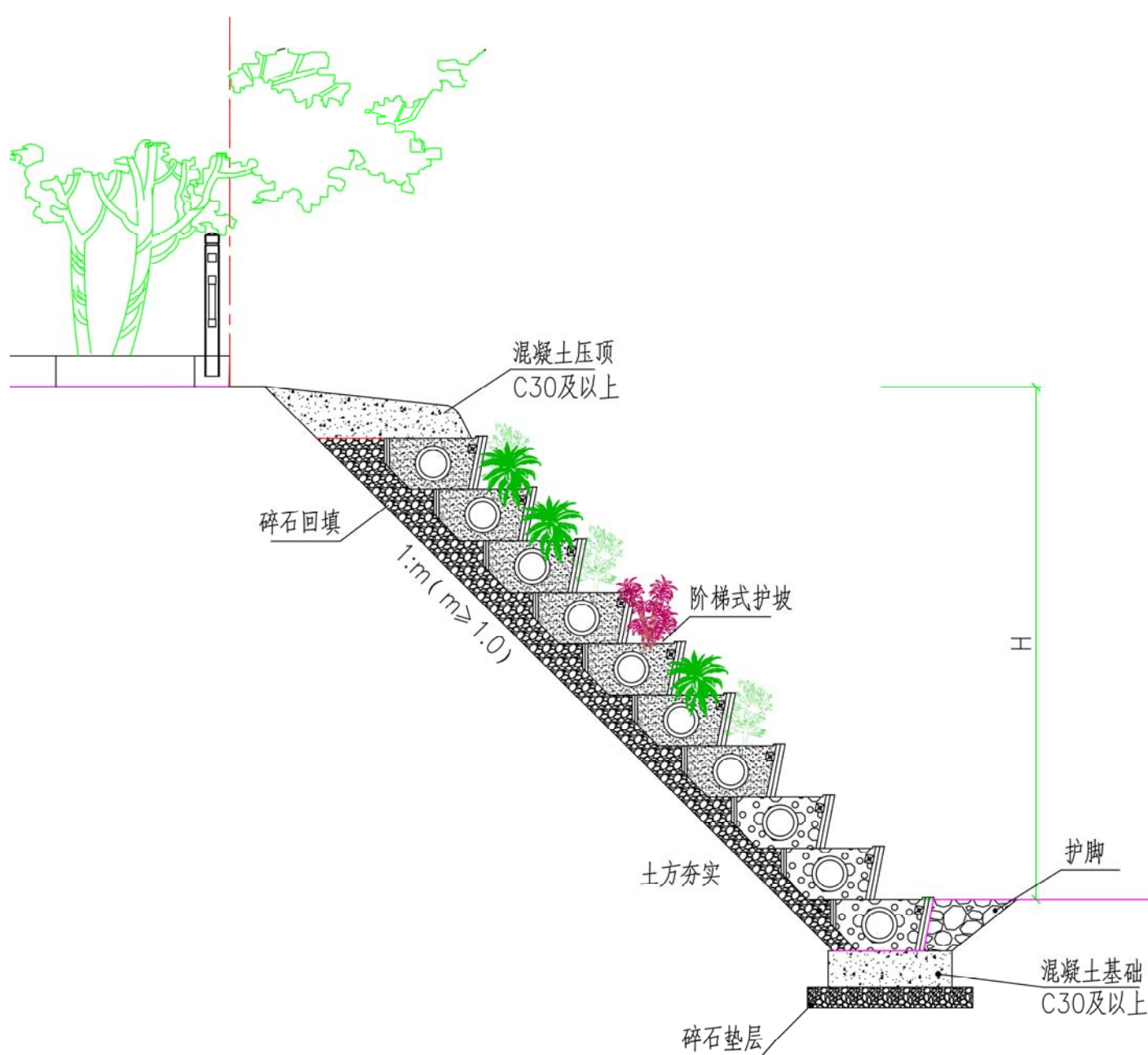
阶梯式生态护坡砌块安装剖面图
