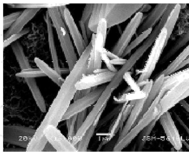
钙矾石晶体
