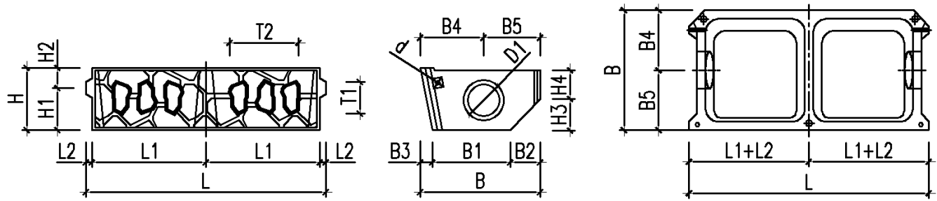
阶梯式生态护坡砌块砌块尺寸图
