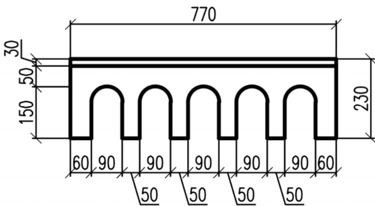
侧立式雨篦 2 大样图
