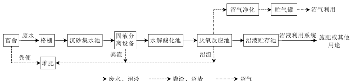
图 7.2-1 模式 II 处理工艺基本流程
