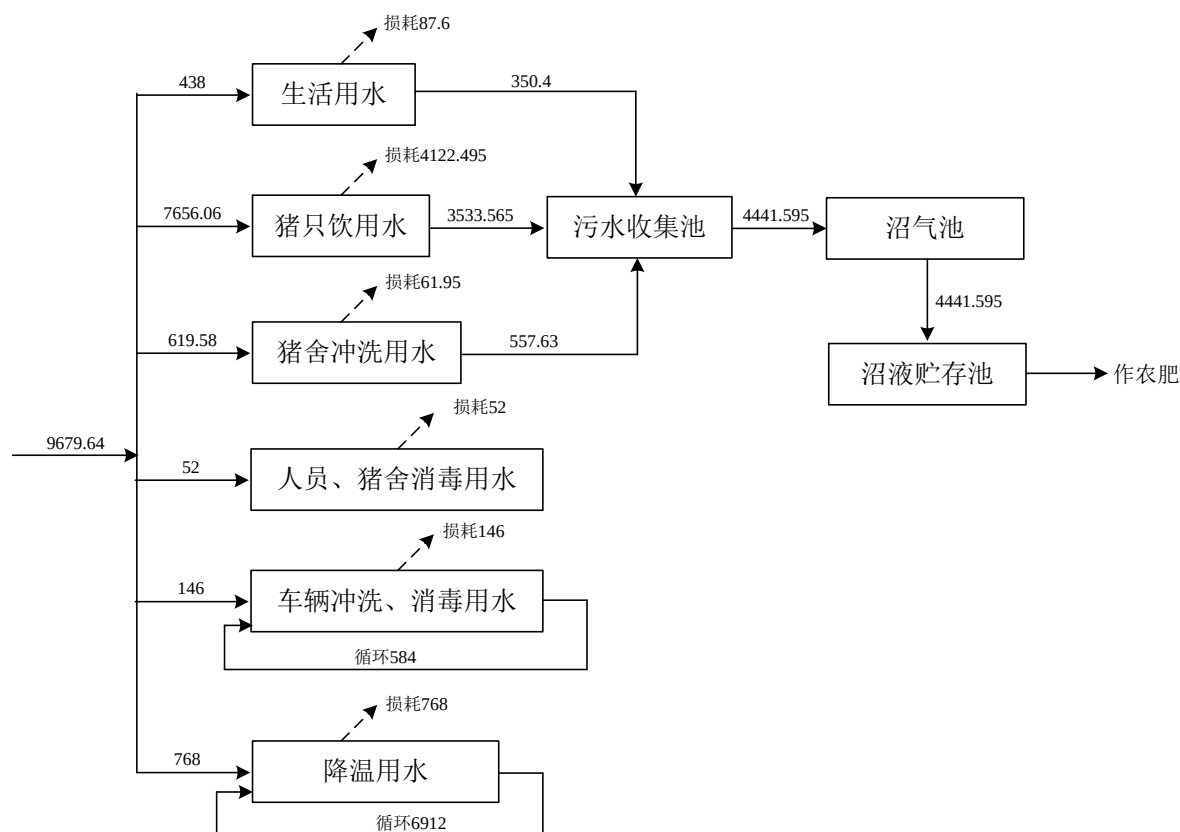
图 3.2-4 项目水平衡分析 ( \text{m}^3/\text{a} )
