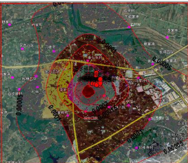
图 6.2-14 NH 3 年均浓度贡献值等值线图
