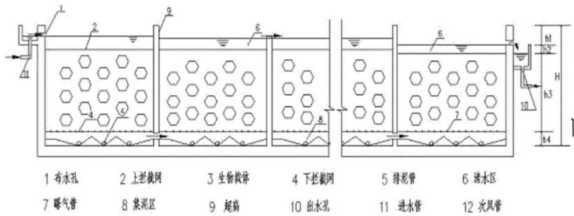
图 8.2-2 曝气生物流化池构造示意图
