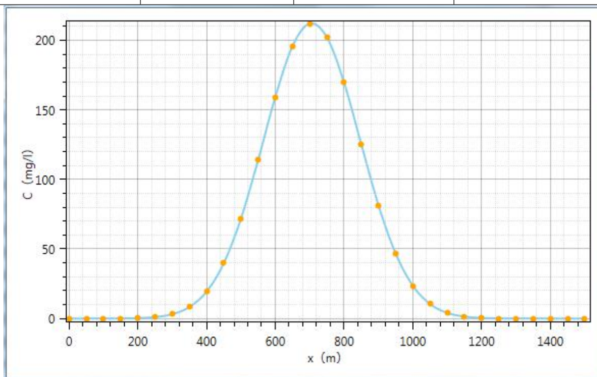
图 6.2-16 1000 天 \text{NH}_3\text{-N} 迁移距离曲线图
