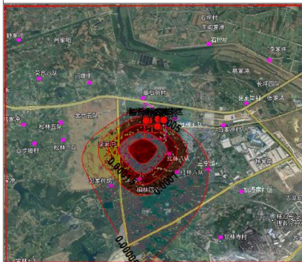
图 6.2-11 HCl 日均浓度贡献值等值线图
