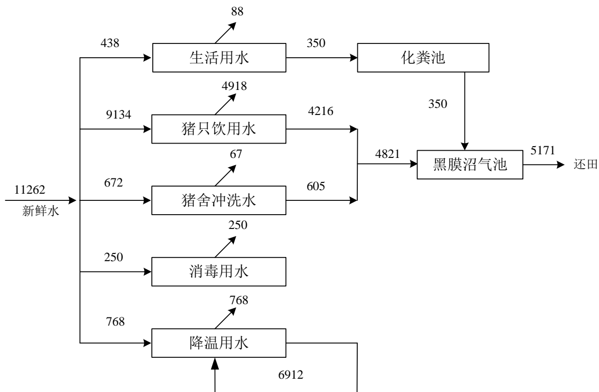
图 3.2-4 项目水平衡分析 (m³/a)
