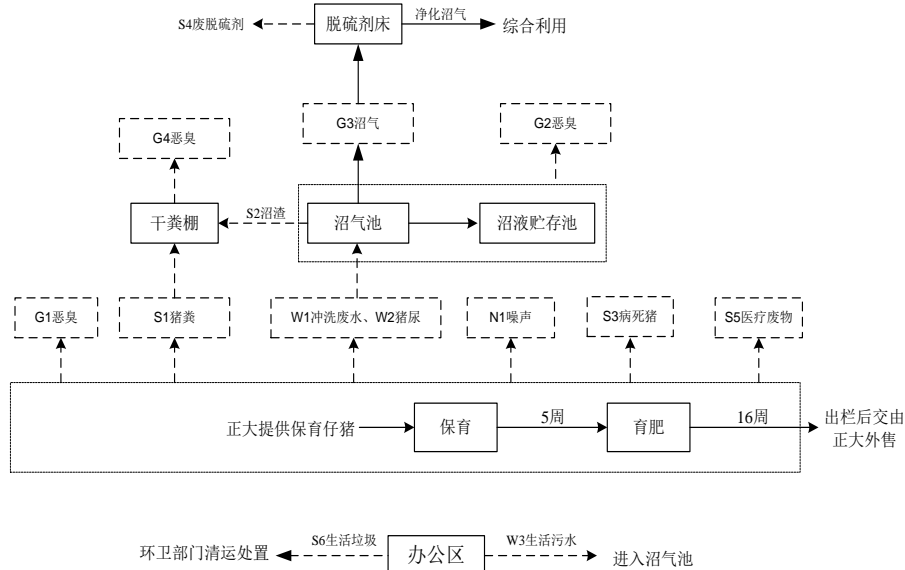
图 3.2-3 项目产污环节示意图
