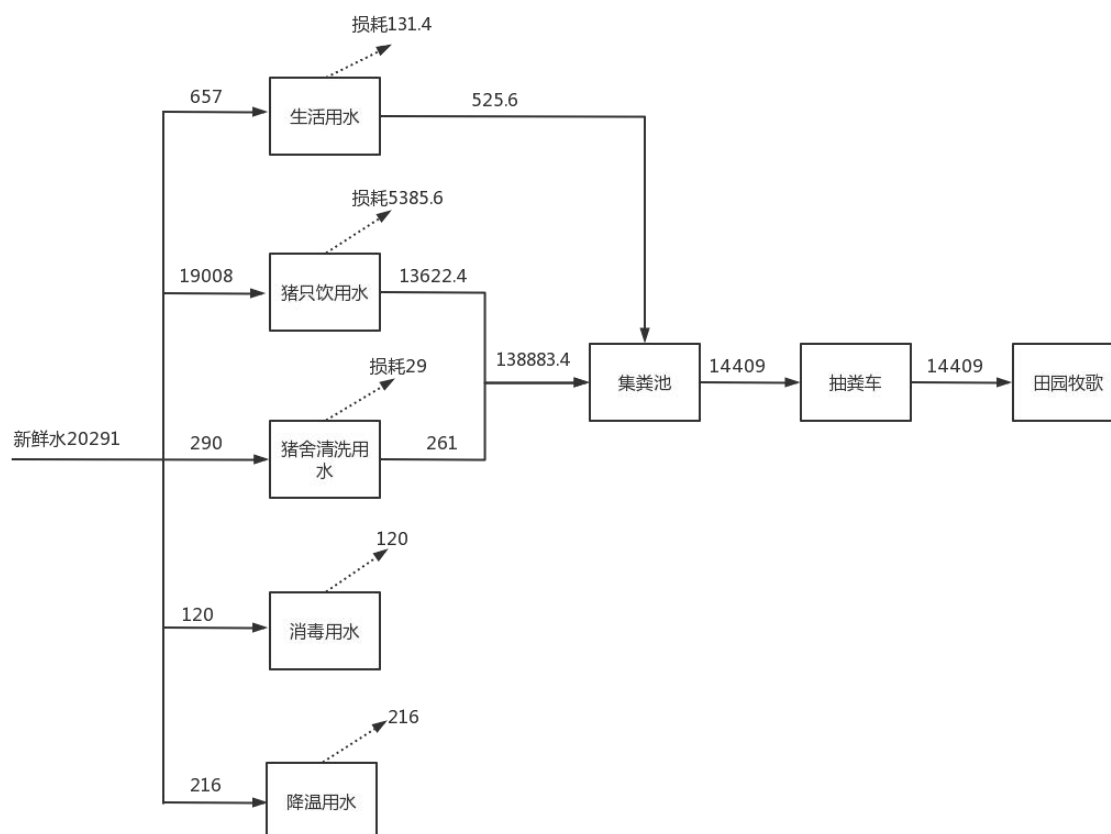
图 3.4-4 项目给排水平衡图 (单位: t/a)
