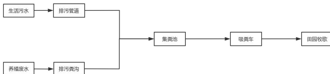
图6.3.1 项目废水处理流程图
