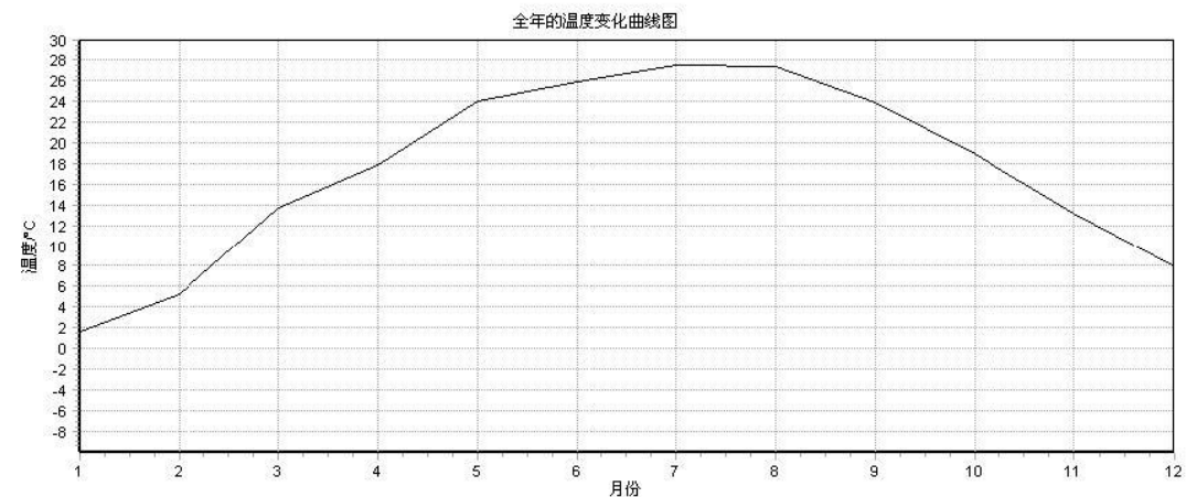
图 6.2-4 枝江市全年温度变化曲线图
