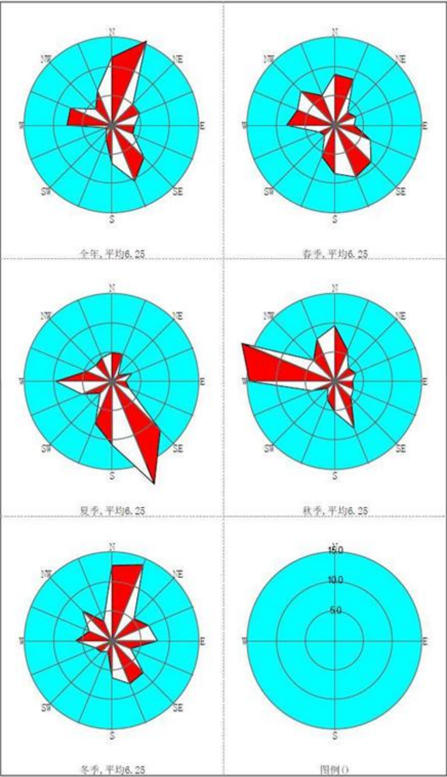
图 6.2-3 枝江市污染系数玫瑰图
