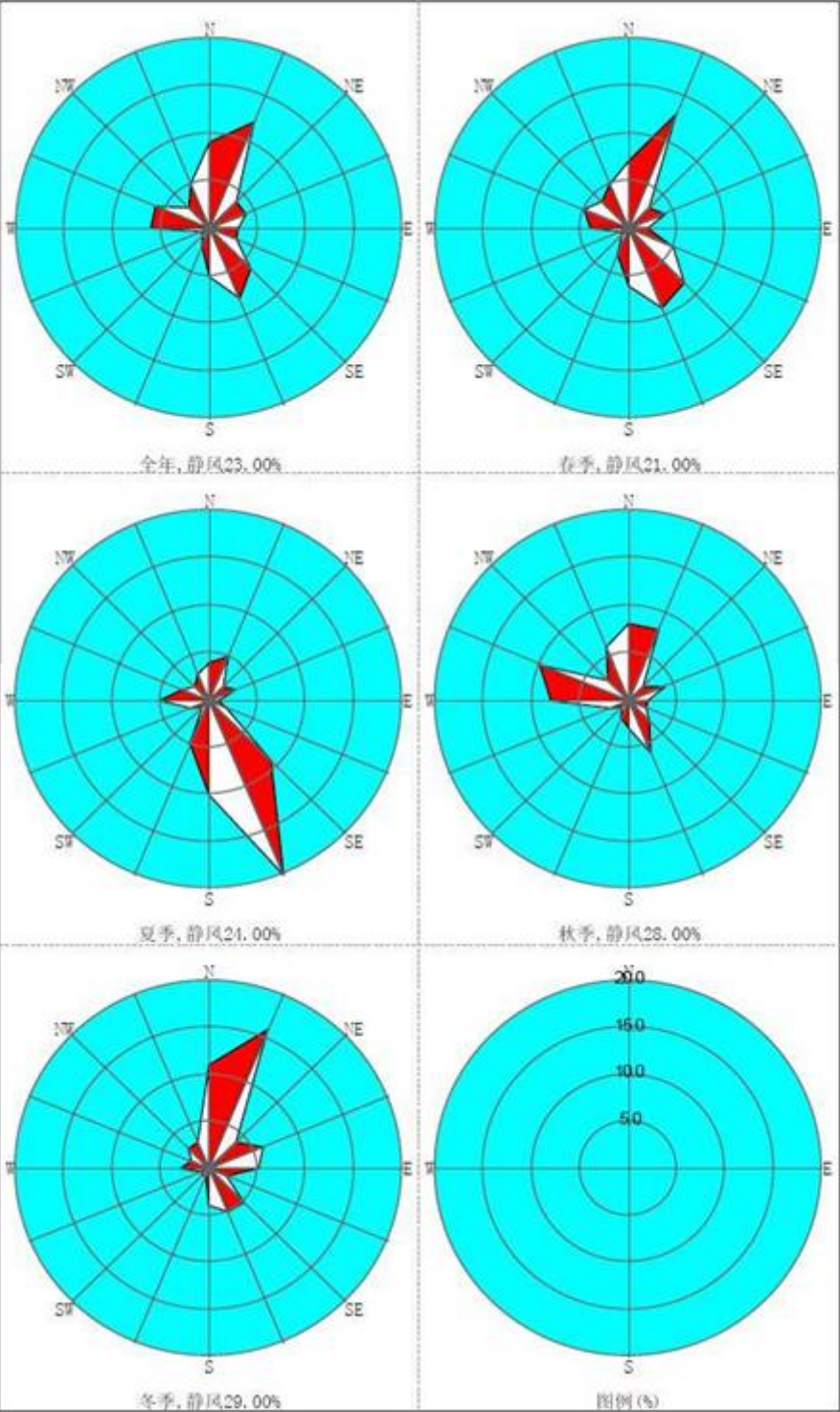
图 6.2-2 枝江市近五年风向风频玫瑰图
