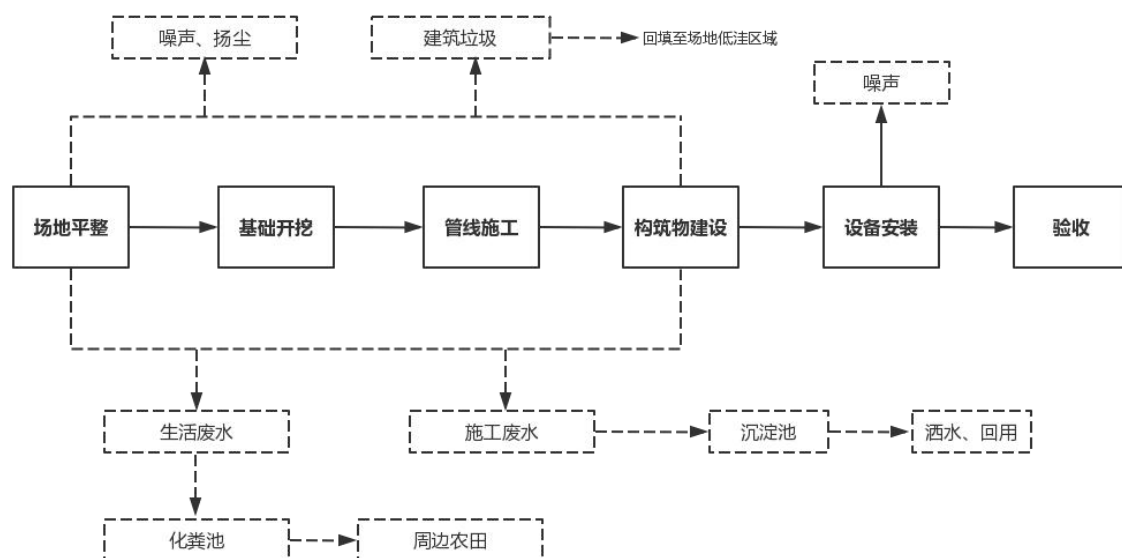
图 3.4-1 施工期工艺流程
