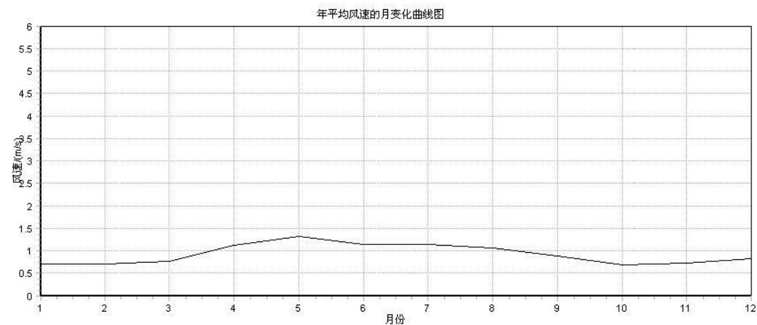
图 6.2-5 枝江市全年平均风速变化曲线图
