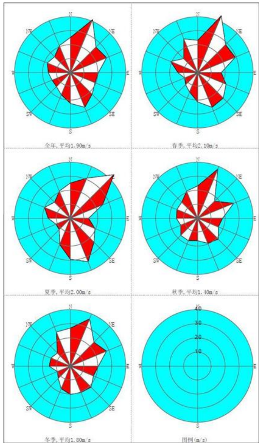
图 6.2-1 枝江市近五年风速玫瑰图
