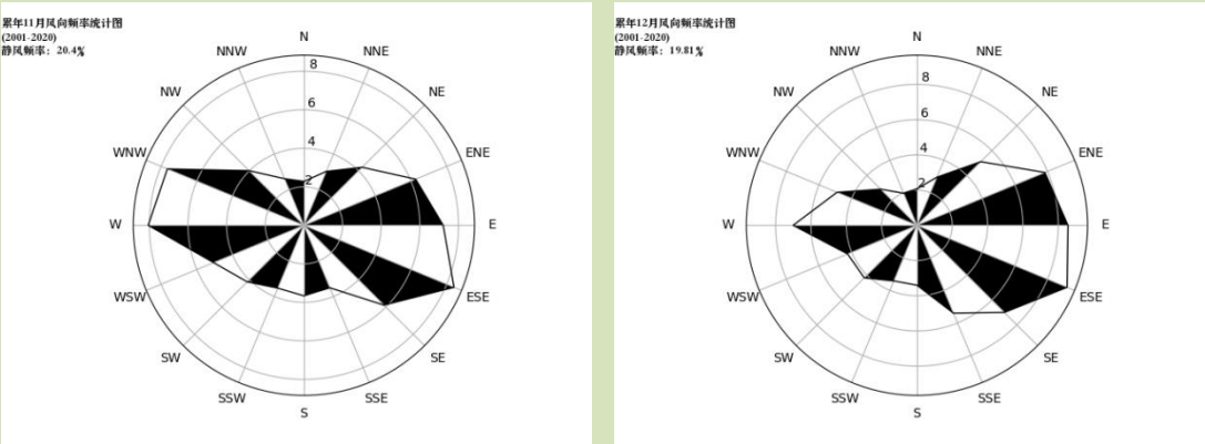
11 月静风 20.40%
