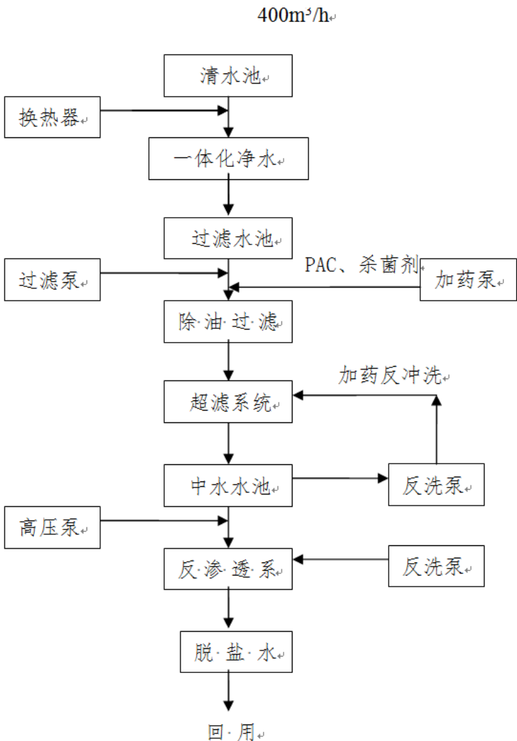
图 9.1-3 现有深度脱盐流程图
