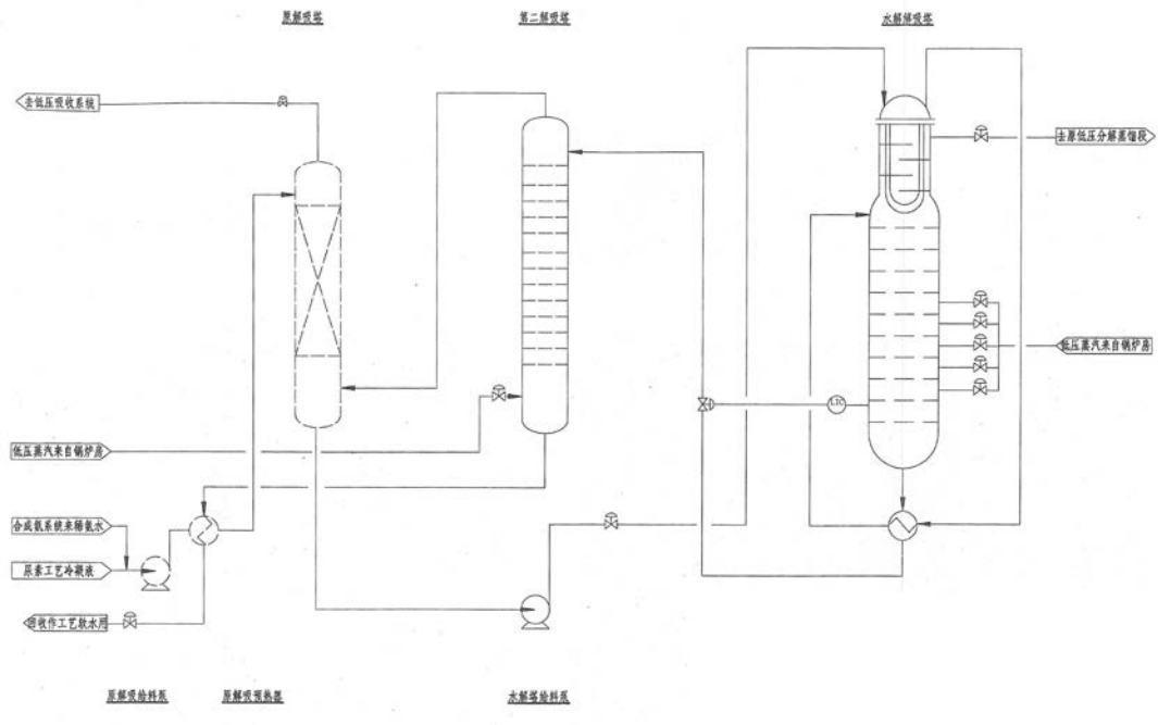
图9.1-1 尿素低压深度水解工艺流程图
