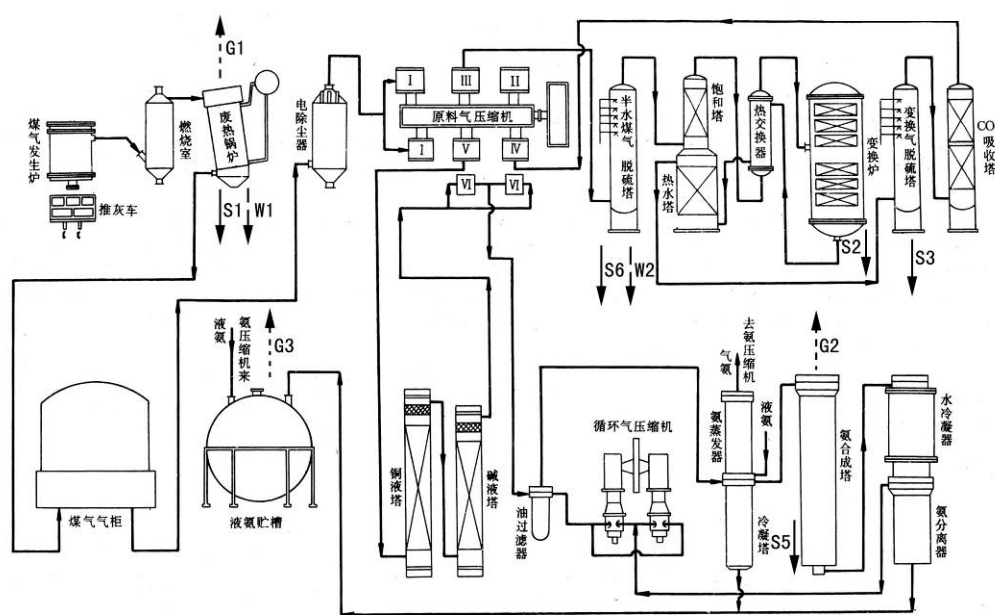
图 3.2-1 合成氨装置主要生产流程及排污节点示意图
