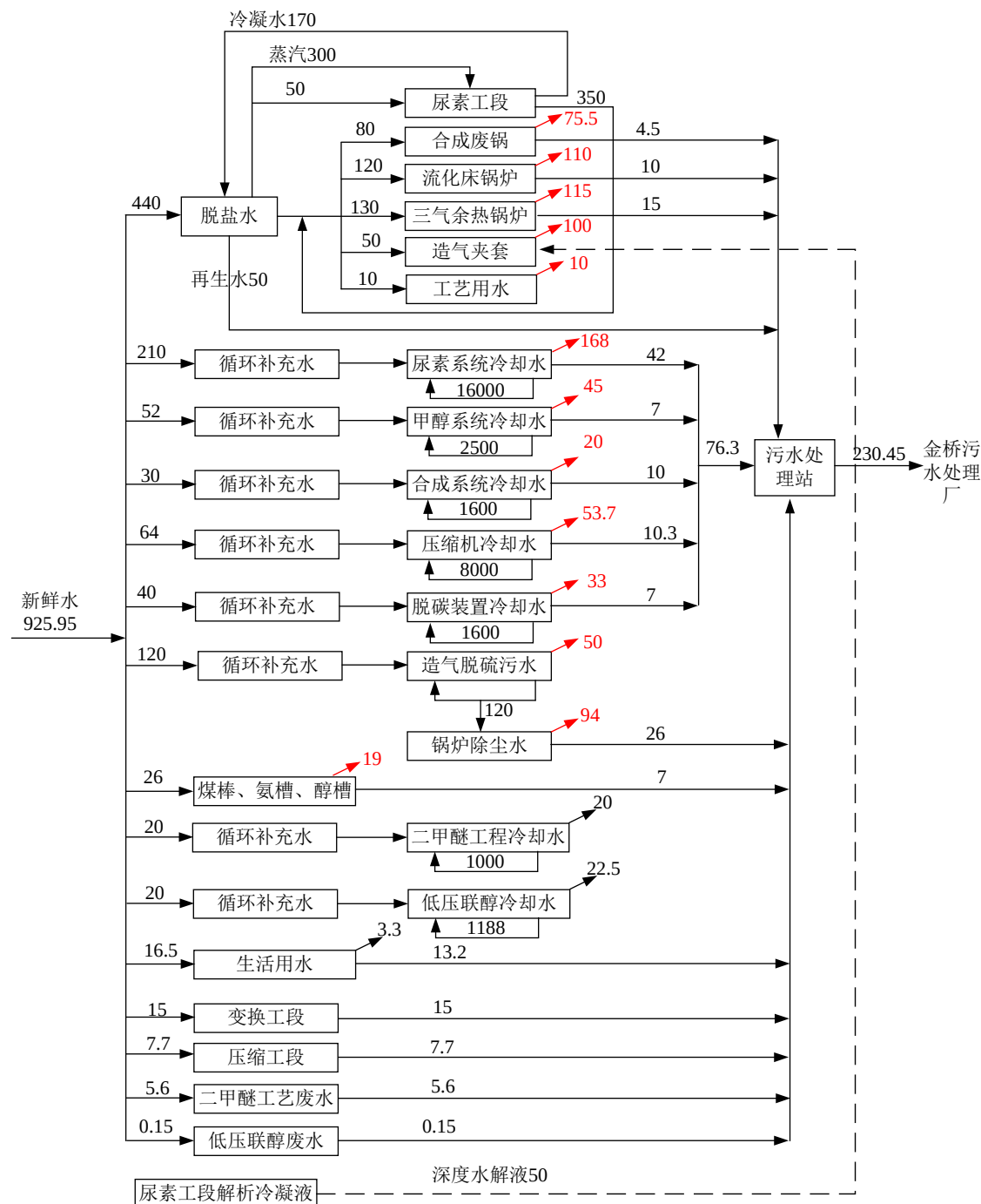
图 5.5-1 拟建项目建成后全厂给排水平衡图 (m³/h)
