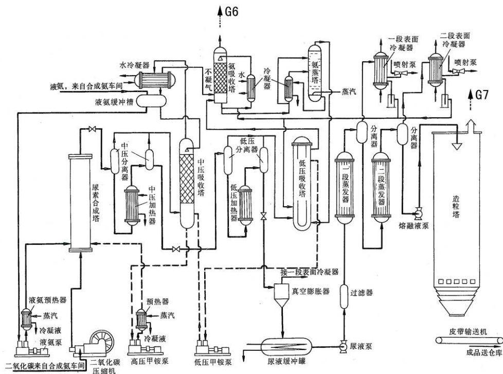
图 3.2-3 尿素装置工艺流程及排污节点示意图
