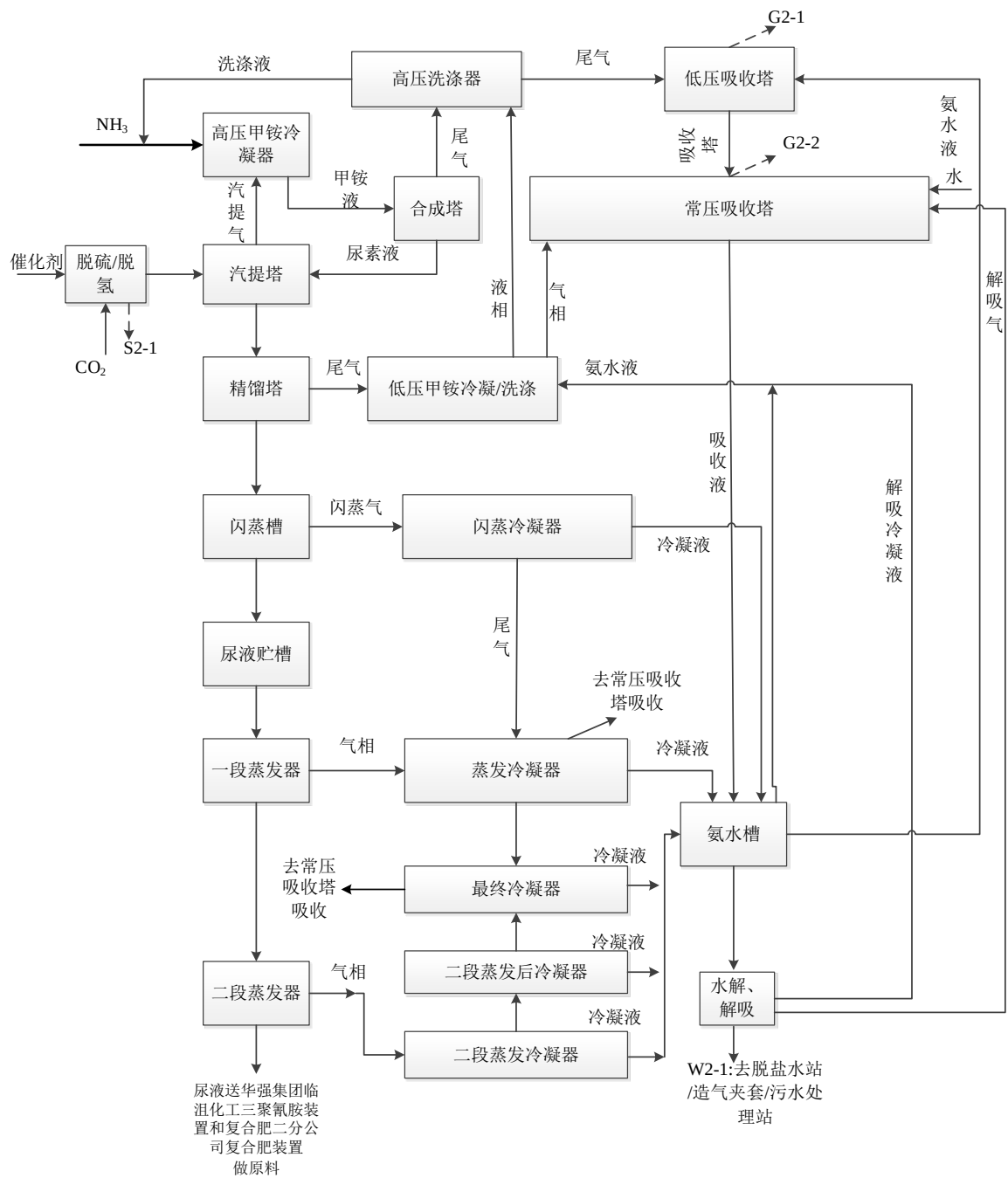
图 5.3-2 二期工程工艺流程及产排污节点图
