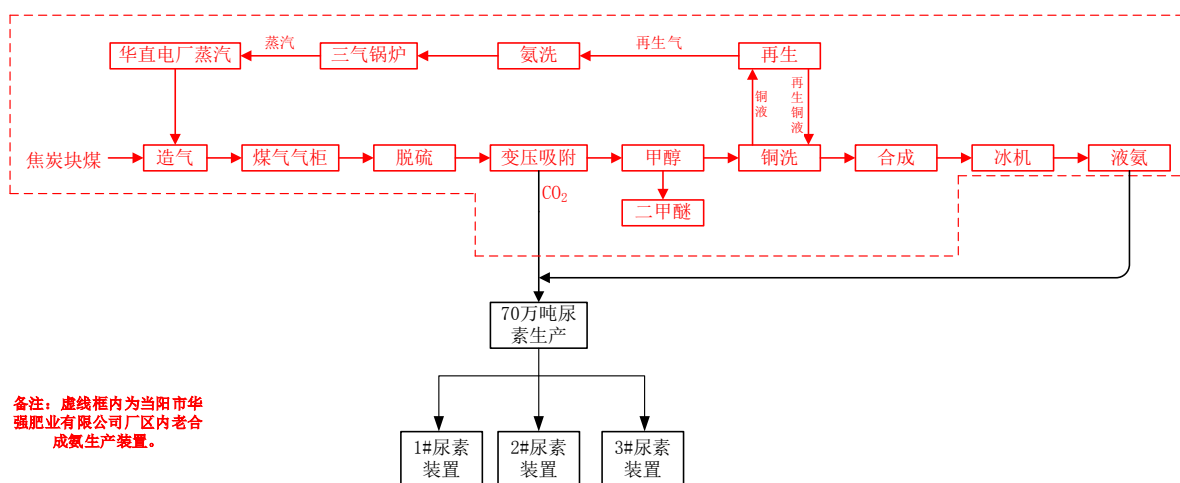
图 4.6-1 拟建项目建设前华强肥业公司全厂物料走向图
