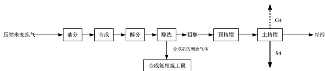
图 3.2-2 甲醇装置生产工艺流程及排污节点示意图
