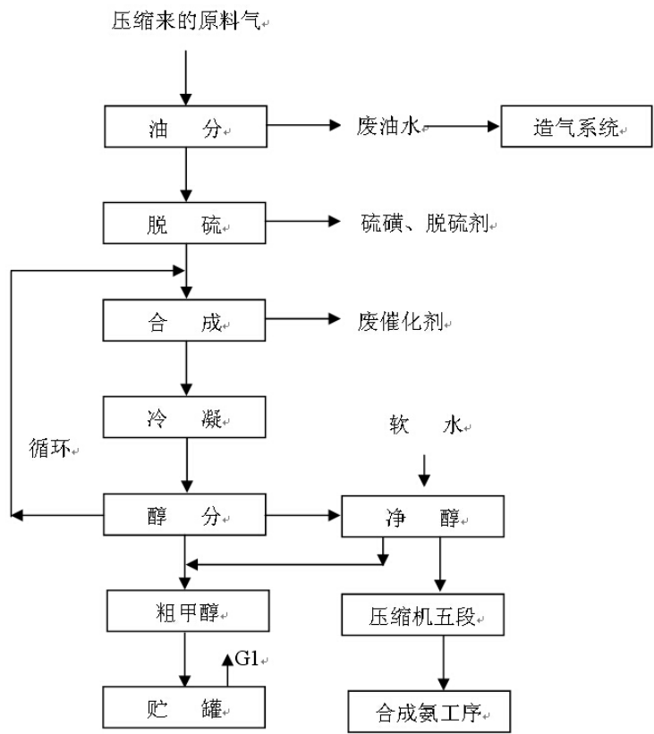
图 3.2-5 低压联醇生产工艺流程及排污节点图
