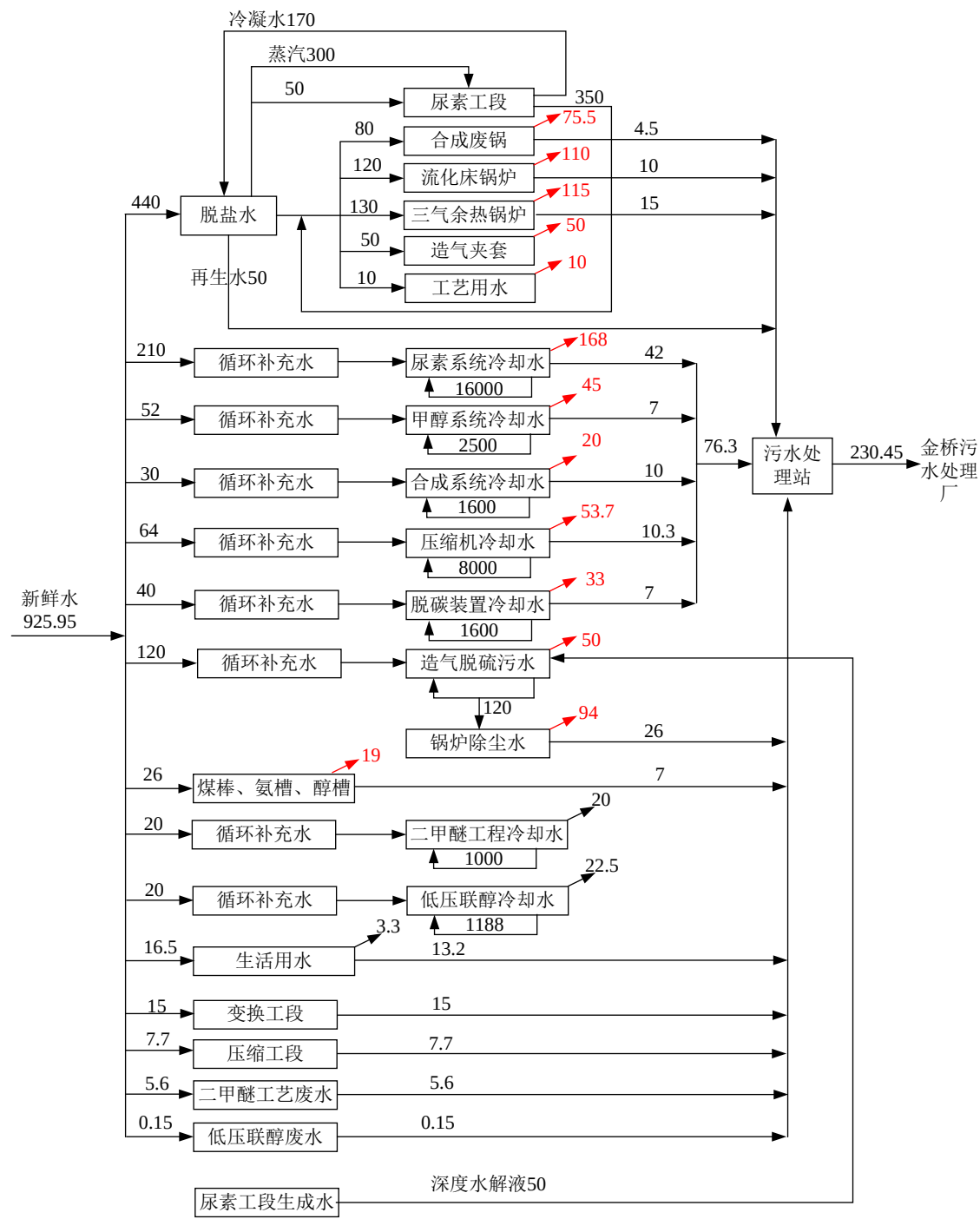
图 3.3-1 当阳市华强肥业有限公司给排水平衡图 (m³/h)
