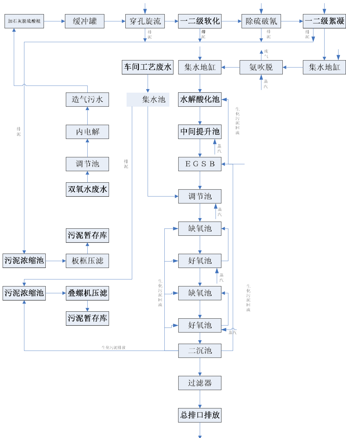
图 9.1-2 厂区现有污水处理站流程图
