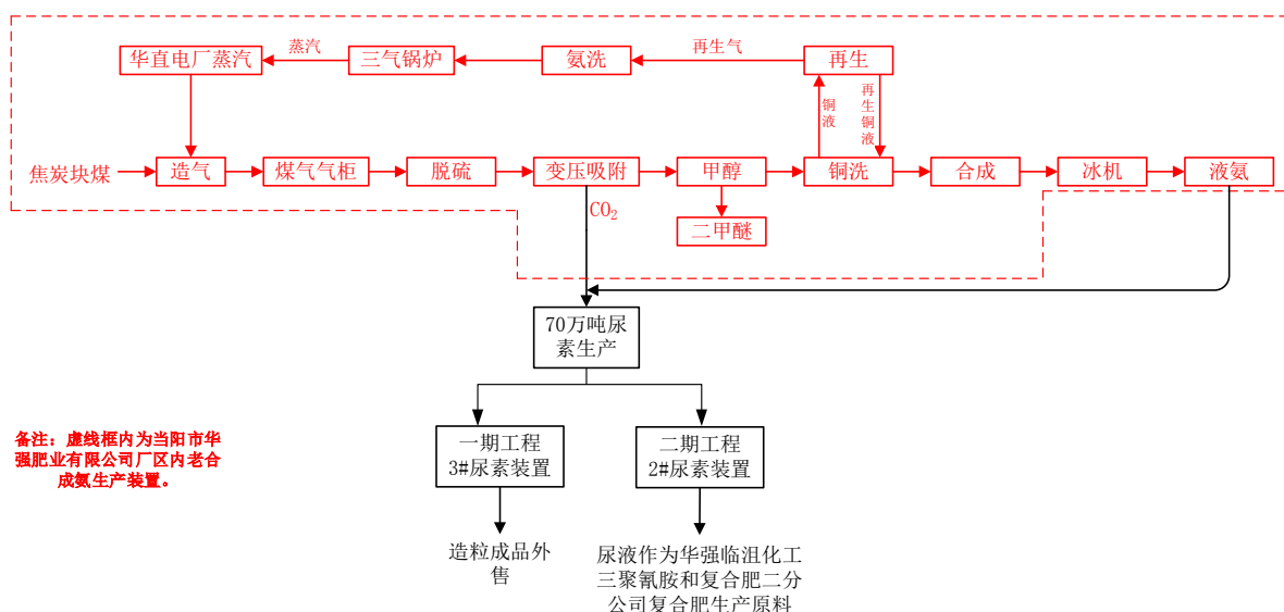
图 4.6-1 拟建项目建设前华强肥业公司全厂物料走向图
