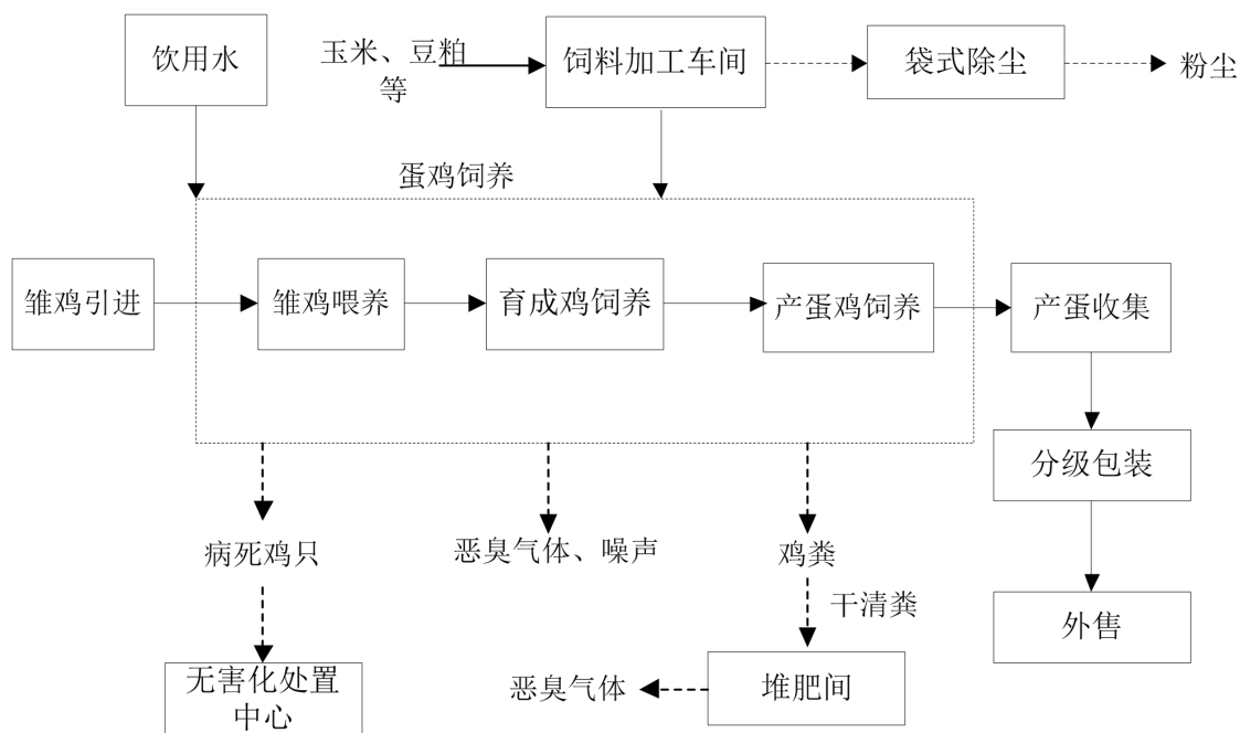
图 3.2-2 蛋鸡饲养工艺流程及产污节点图
