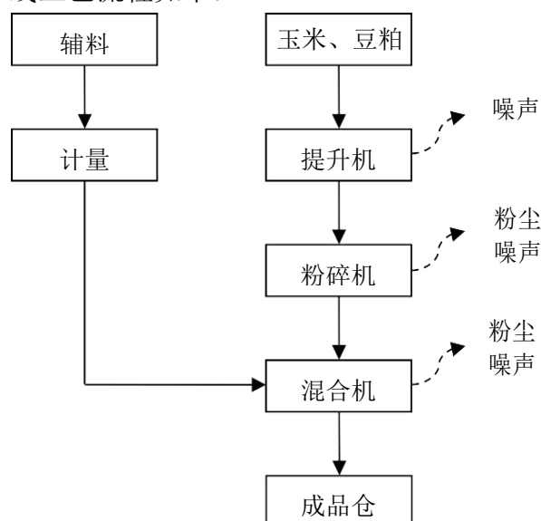
图 3.2-1 饲料加工工艺流程及产污节点图
