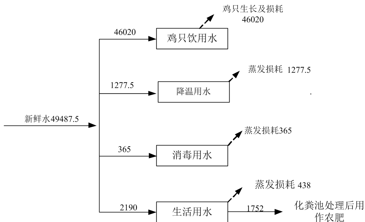
图 3.2-2 项目水平衡图 (单位: t/a)
