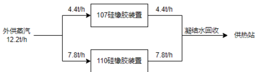
图 3.2-5 项目蒸汽平衡图
