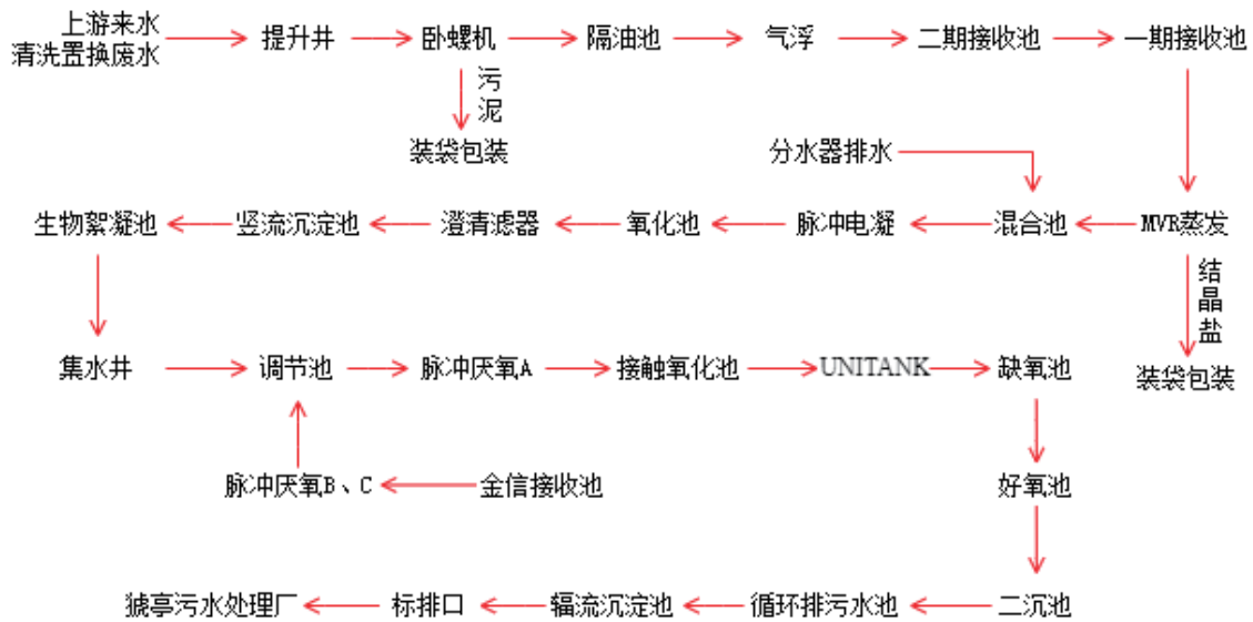
图 7.2-1 兴瑞公司有机硅污水处理站工艺流程示意图
