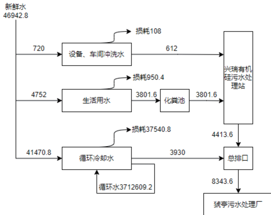
图 3.2-6 扩建项目水平衡图 ( \text{m}^3/\text{a} )
