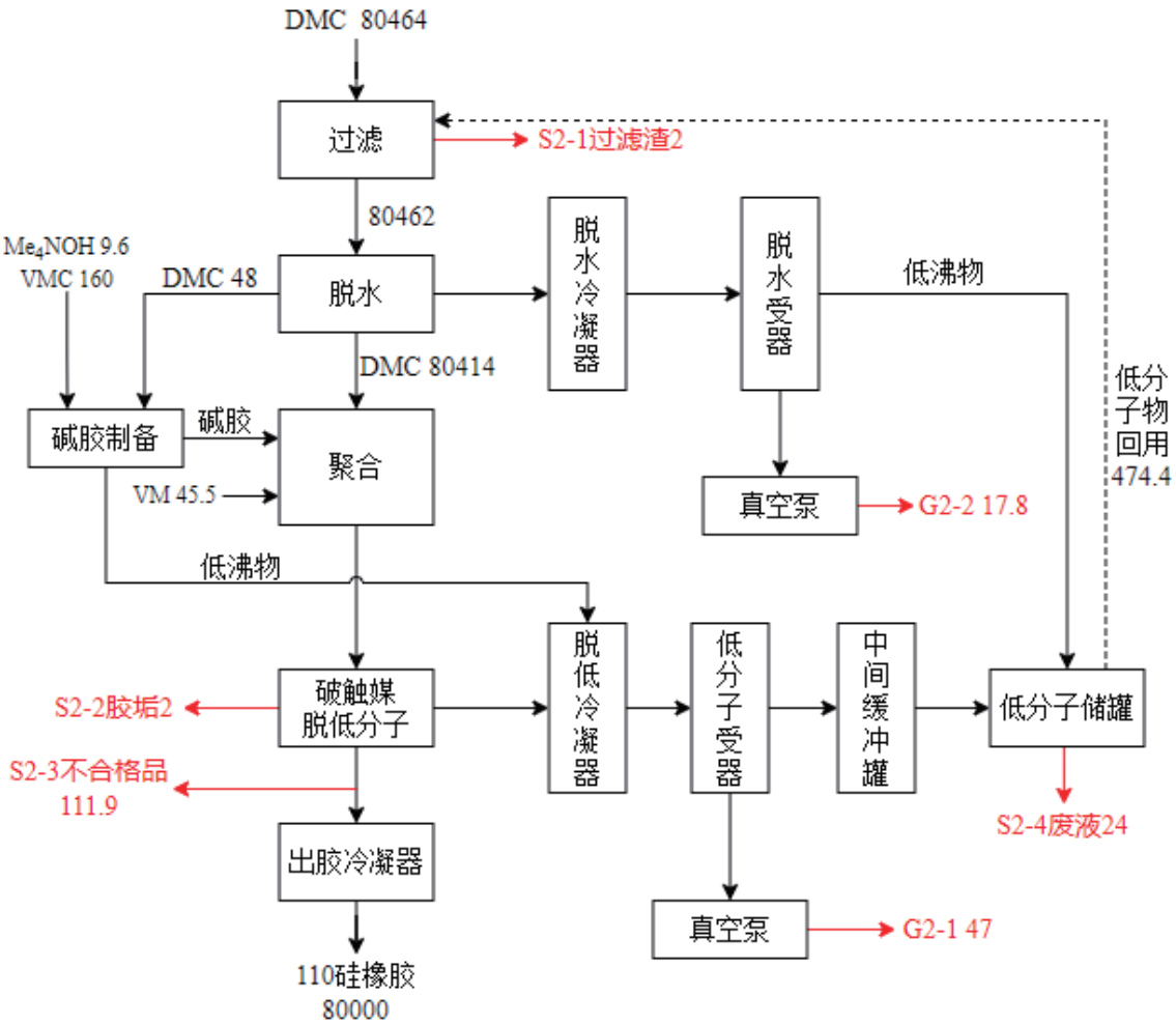
图 3.2-4 110 硅橡胶生产物料平衡图（单位：t/a）
