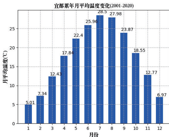
图 5.1-1 宜都月平均气温 (单位: °C)
