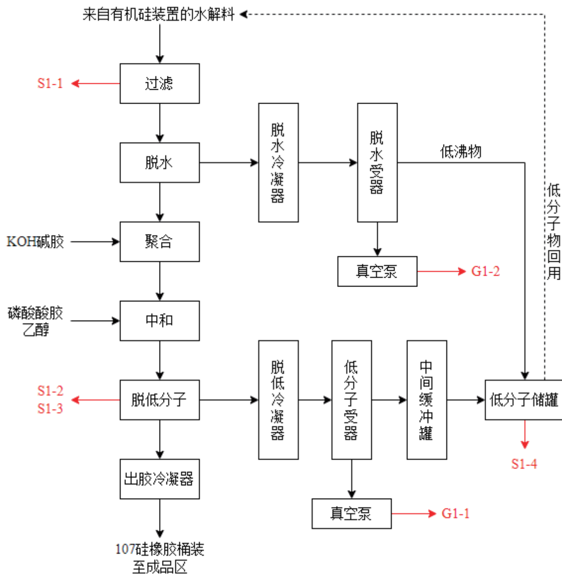
图 3.2-1 107 硅橡胶生产工艺及排污节点
