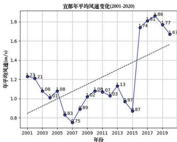
图 5.1-5 宜都 (2001-2020) 年平均风速 (单位: m/s, 虚线为趋势线)
