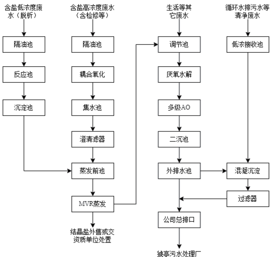
图 2.5-2 扩建污水处理站处理工艺流程
