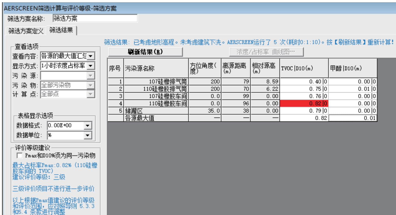
图 5.1-13 大气估算模型 AERSCREEN 计算结果
