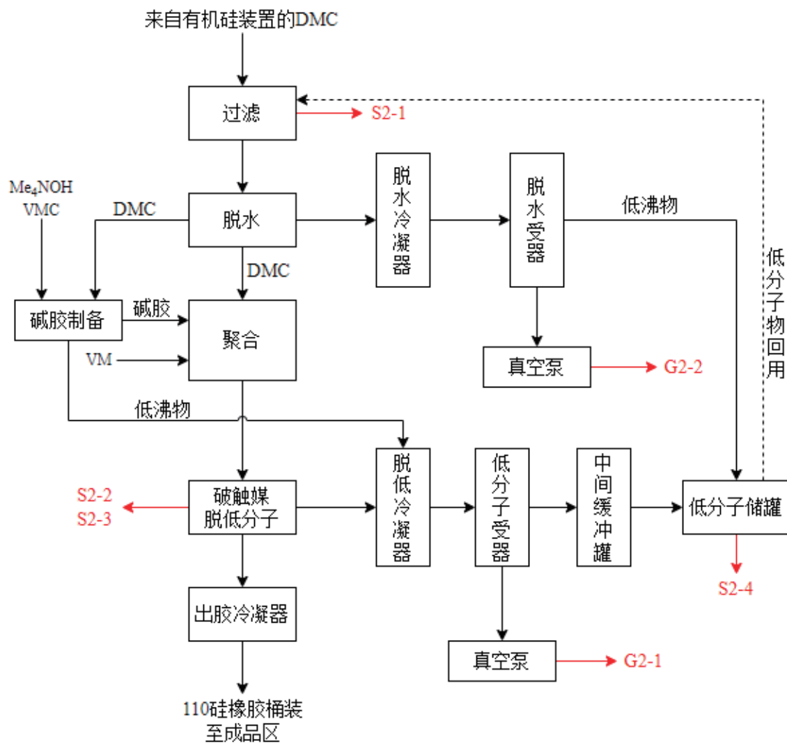
图 3.2-3 110 硅橡胶生产工艺及排污节点
