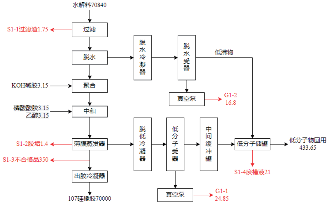
图 3.2-2 107 硅橡胶生产物料平衡图（单位：t/a）
