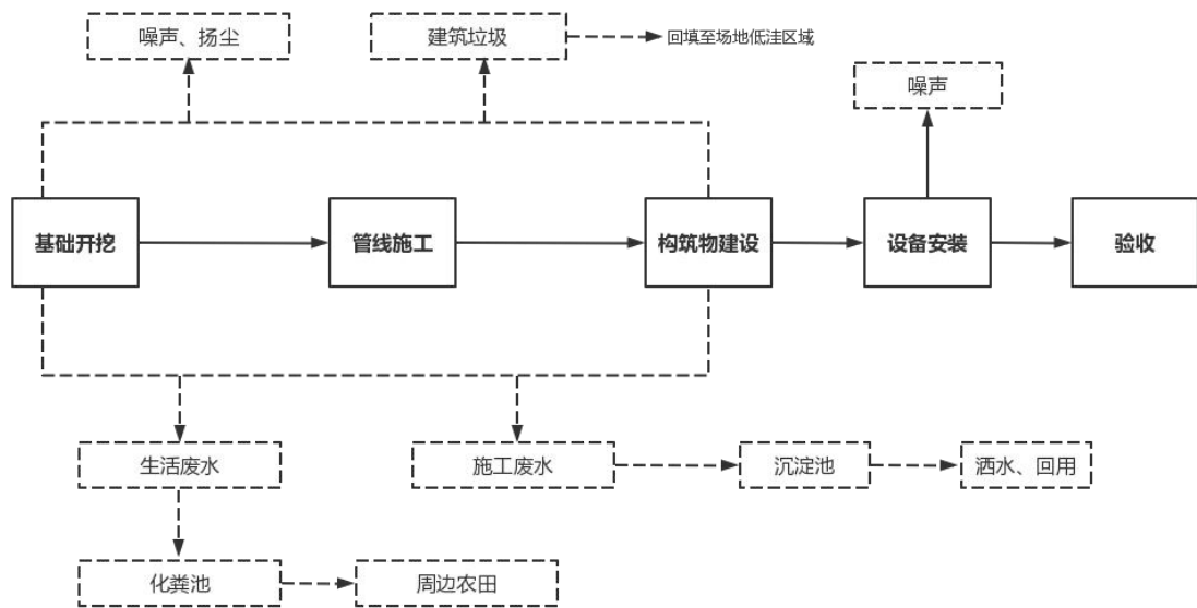
图 3.3-1 施工期工艺流程
