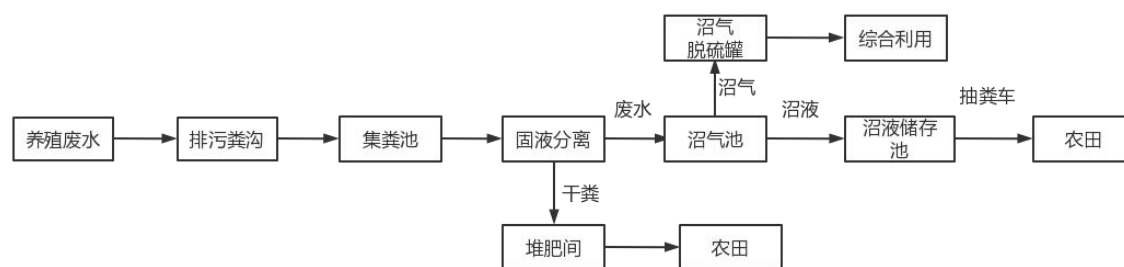
图6.3.1 项目A区废水处理流程图
