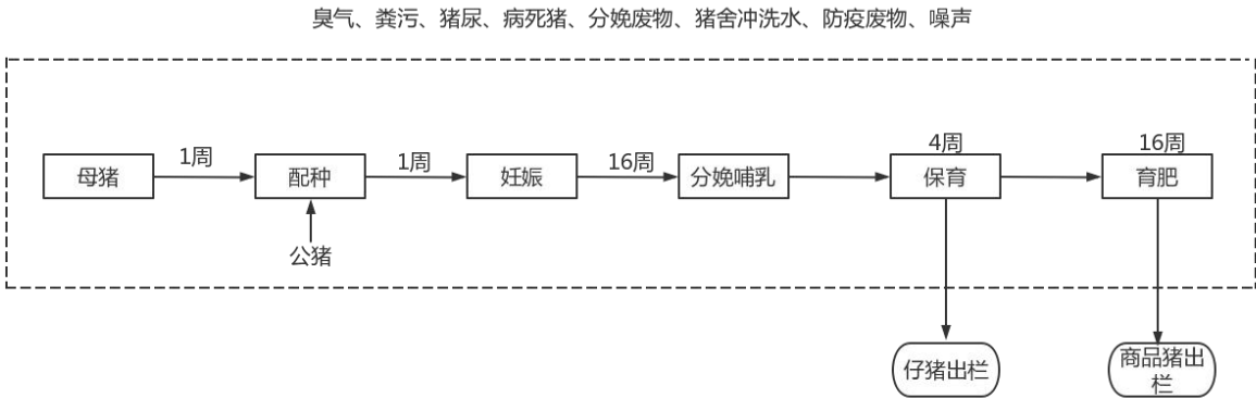
图 3.3-2 生猪养殖工艺流程图
