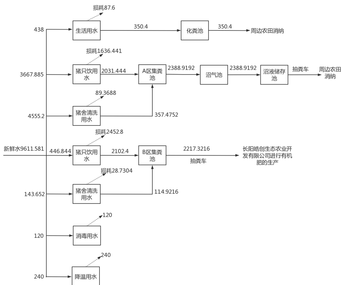
图 3.3-4 项目给排水平衡图 (单位: t/a)
