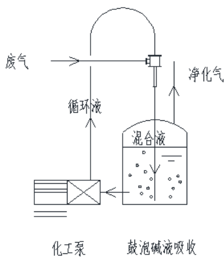
图 10.1.3-3 鼓泡吸收工艺示意图
