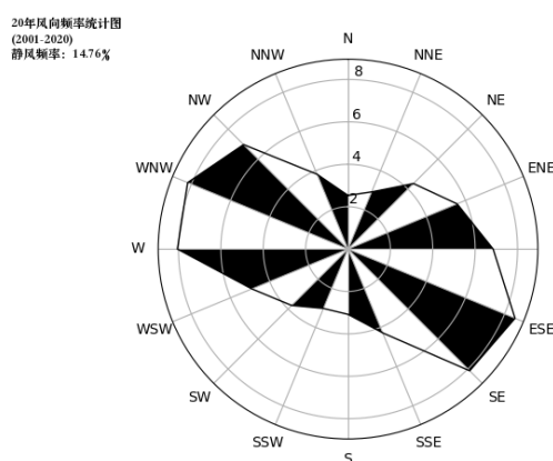
图 8.2.1-1 宜都风向玫瑰图（静风频率 14.76%）
