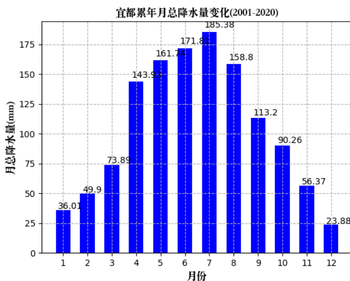
图 8.2.1-5 宜都月平均降水量（单位：毫米）
