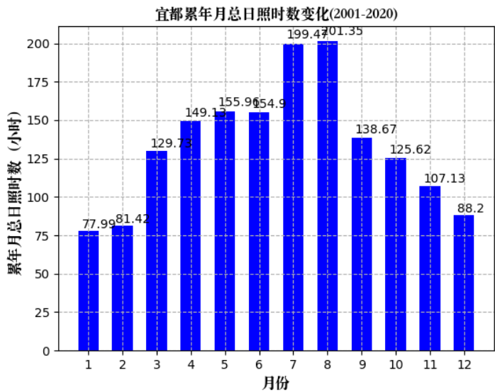
图 8.2.1-7 宜都月日照时数（单位：小时）
