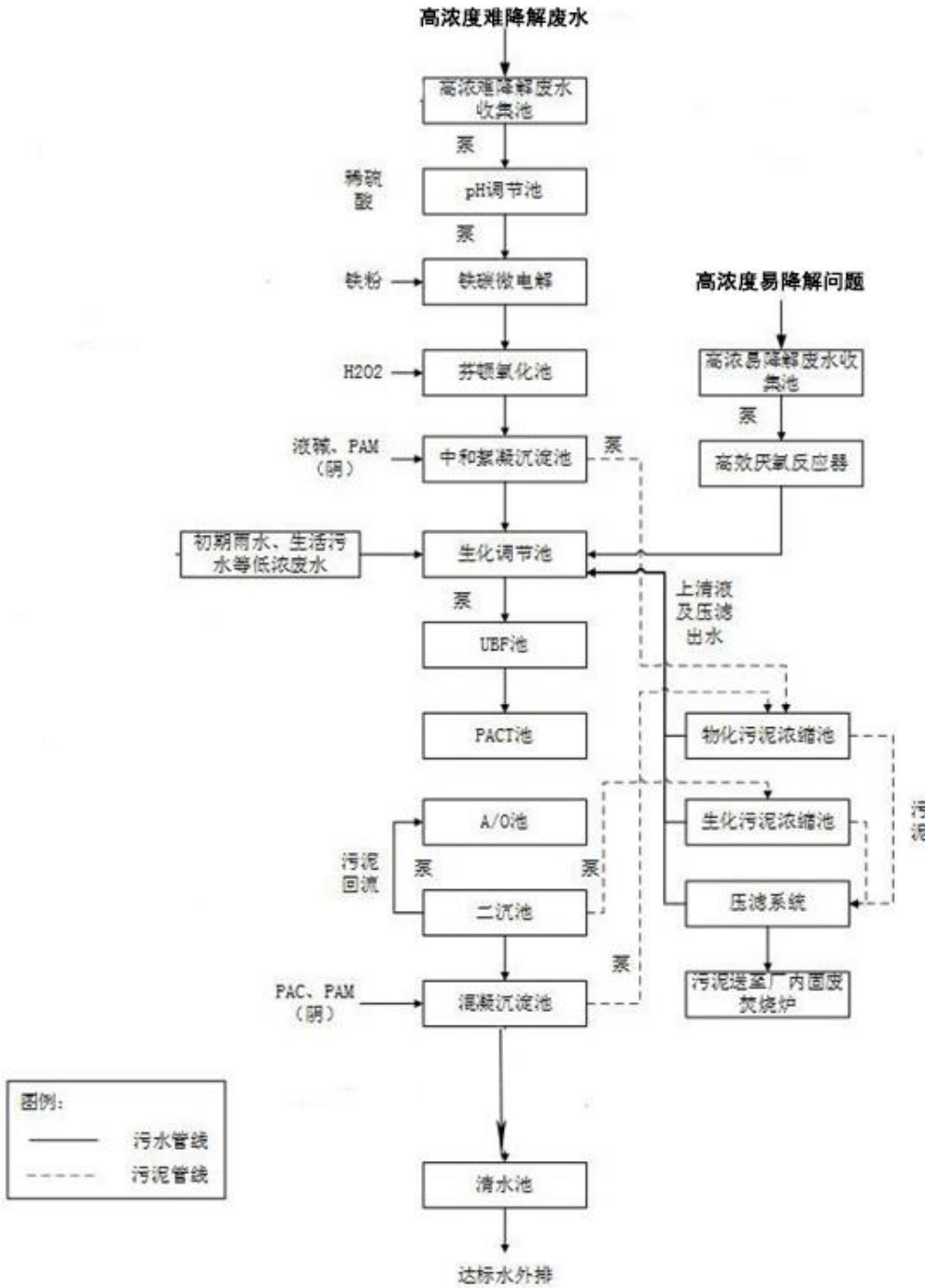
图 10.2.2-1 拟建项目污水处理站工艺流程图
