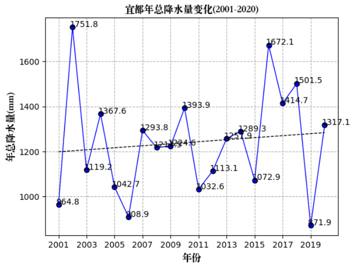
图 8.2.1-6 宜都（2001-2020）年总降水量（单位：毫米，虚线为趋势线）
