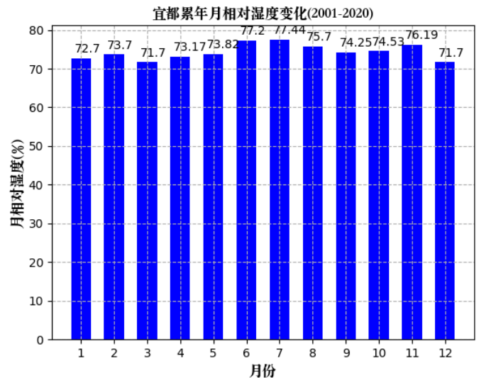
图 8.2.1-9 宜都月平均相对湿度（纵轴为百分比）
