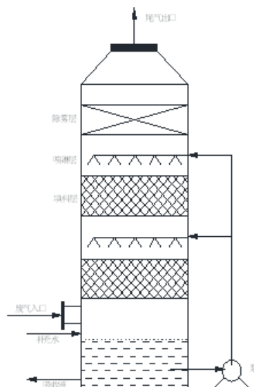
图 9.1.3-2 喷淋吸收工艺示意图
