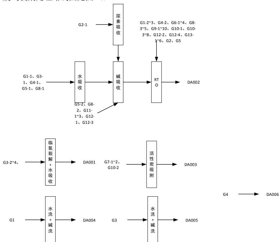
图 9.1-1 废气收集处理路线图
