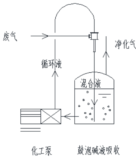
图 9.1.3-3 鼓泡吸收工艺示意图
