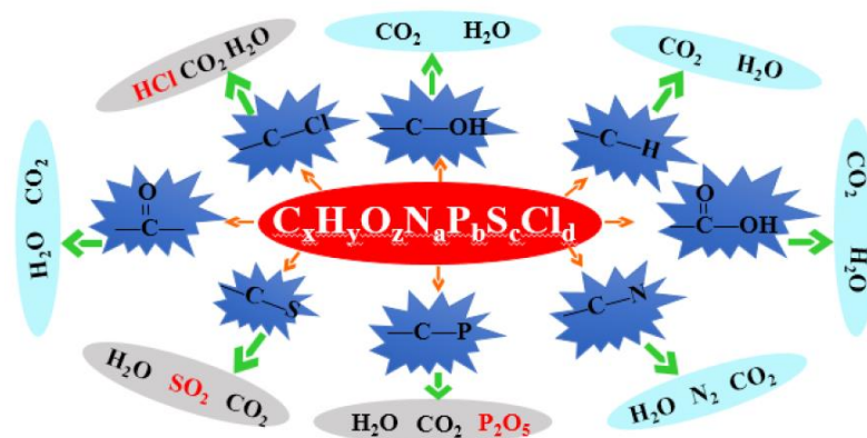
图 9.1.4-1 临氧裂解反应原理示意图
