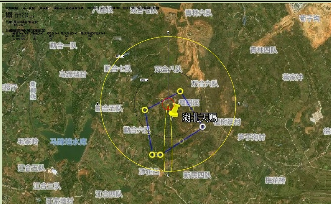
图 6.6-1 硫酸最不利气象条件下泄露扩散环境风险预测结果图
