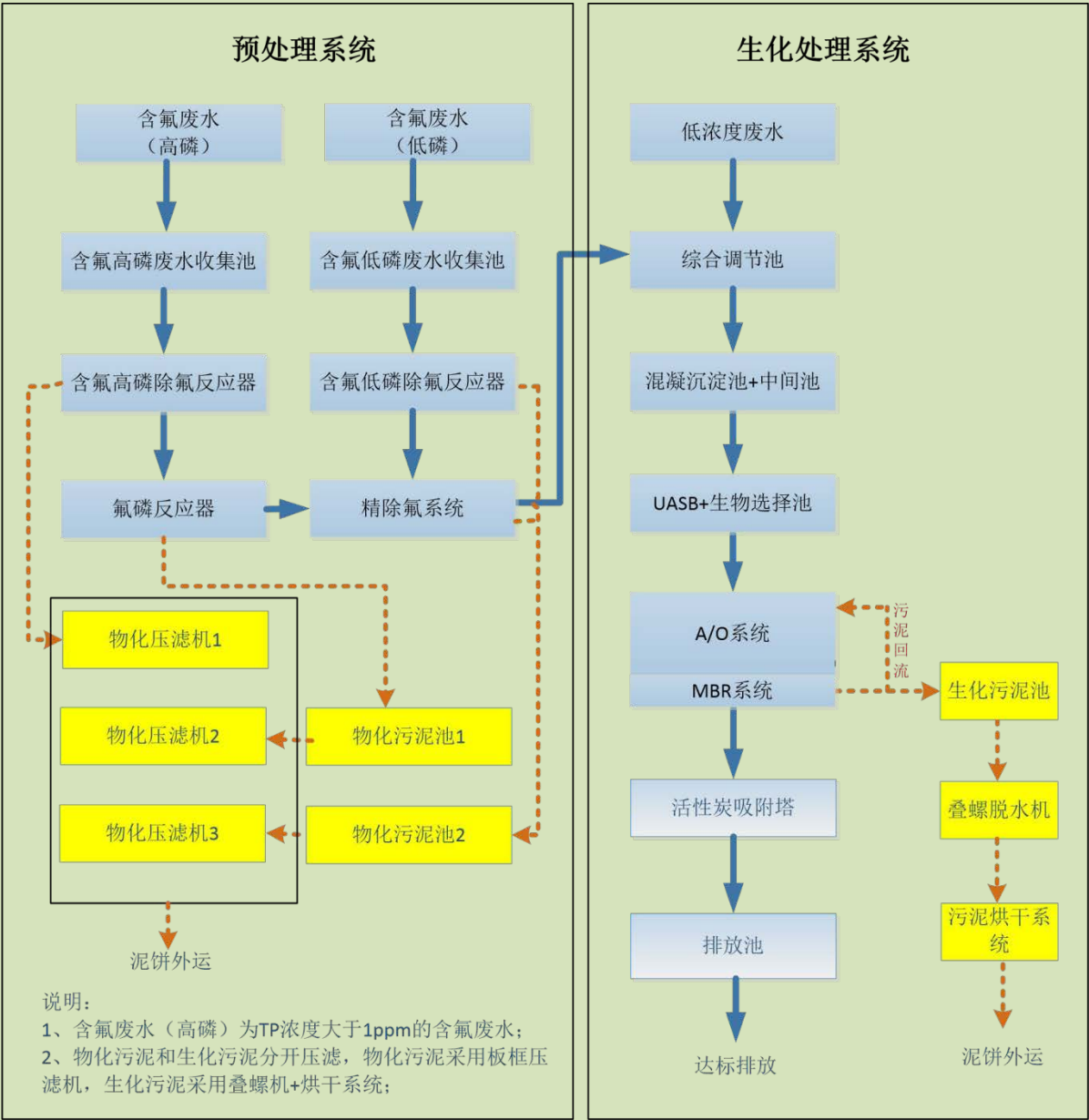
图 2.4-1 废水处理工艺流程图（含废水走向图）
