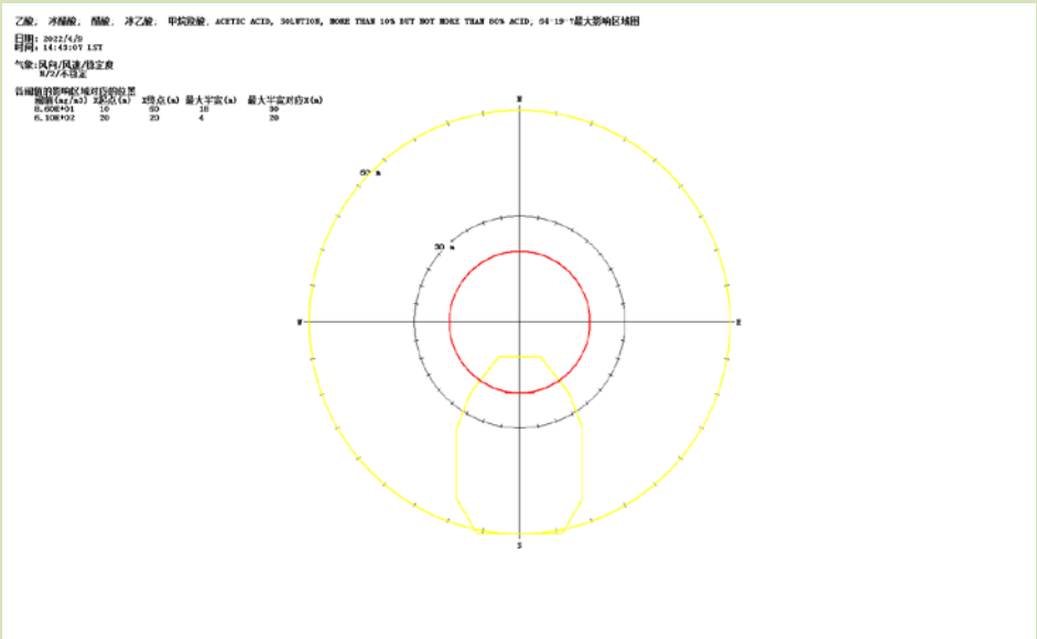
图 6.6-3 乙酸泄露扩散环境风险预测结果图
