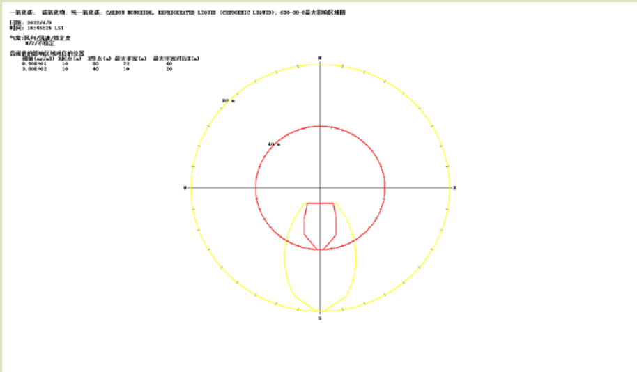
图 6.6-4 乙酸泄露火灾次生 CO 扩散环境风险预测结果图
