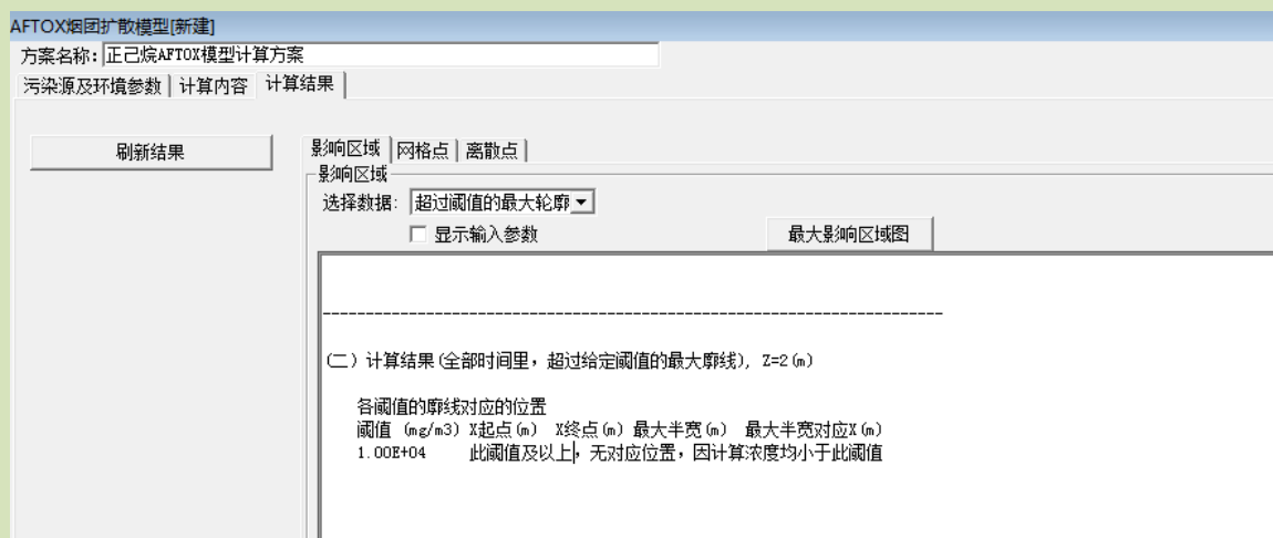
图 6.6-2 正己烷泄露扩散环境风险预测结果图
