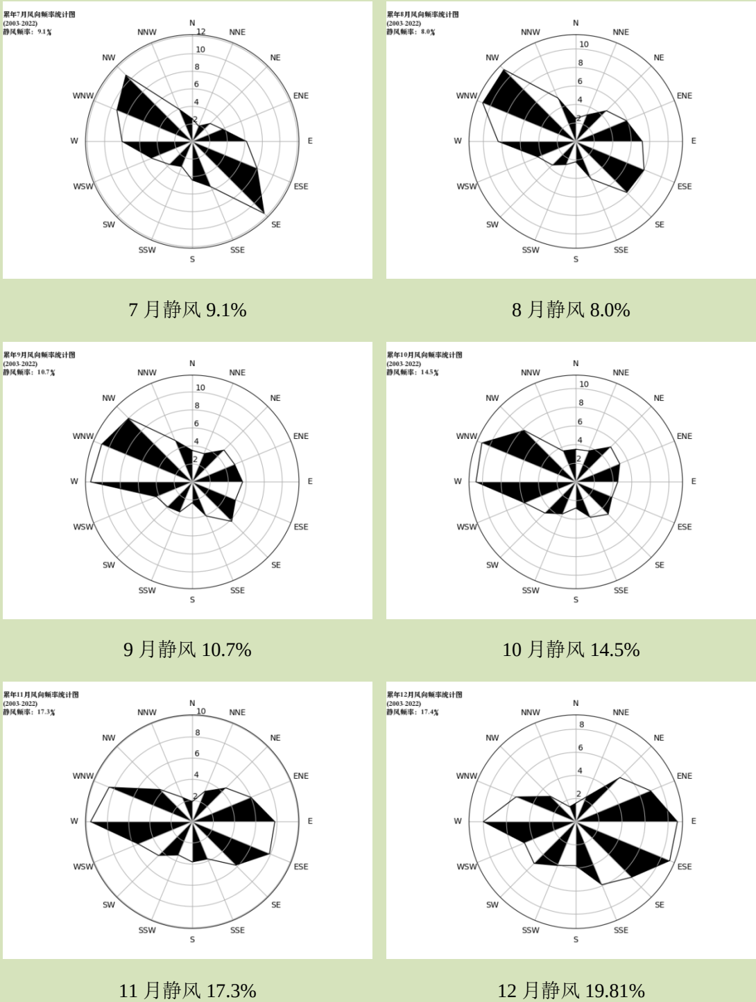
图 5.1-2 宜都月风向玫瑰图
