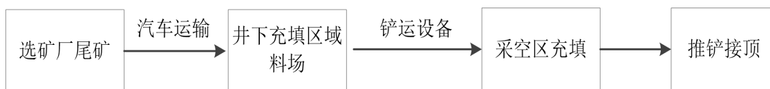
图 3.1-2 干式充填工艺流程
