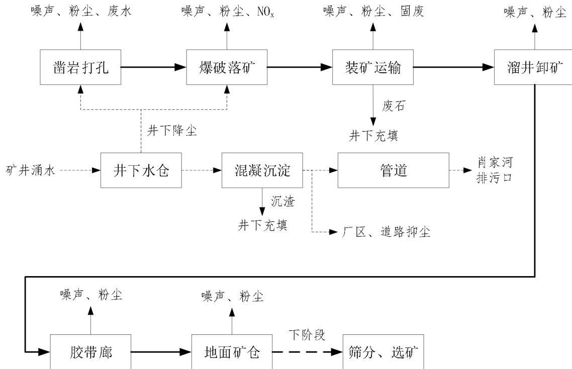
图 3.1-1 采矿工艺流程图
