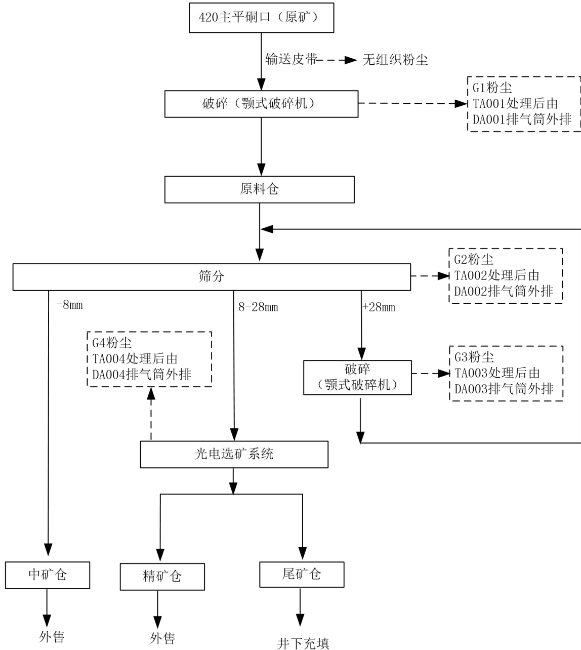
图 4-1 本项目生产工艺流程及产排污节点图
