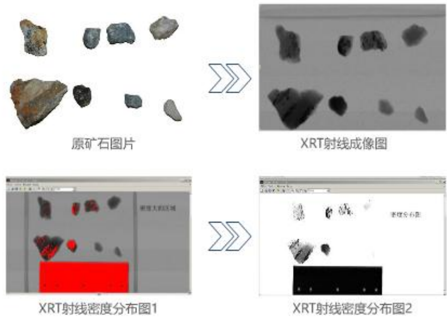
图 4.1-3 XRT 射线技术成像示例图
