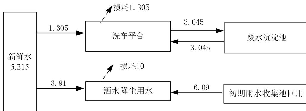
图 4.4-1 日水平衡图（单位： \text{m}^3/\text{d} ）
