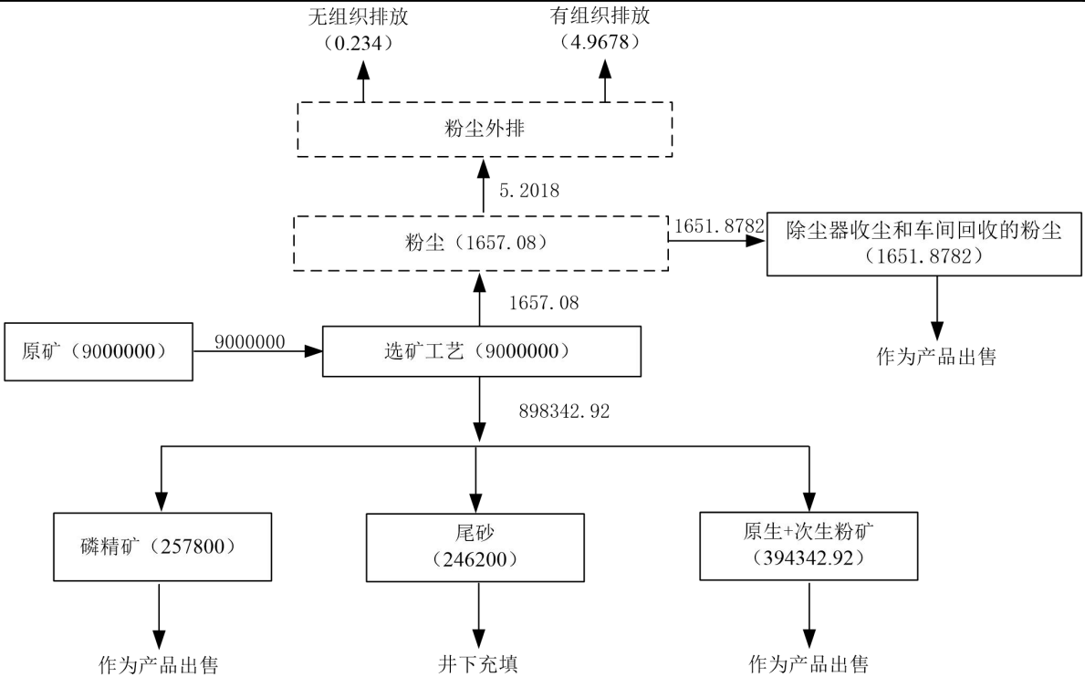
图 4.3-1 物料平衡图
