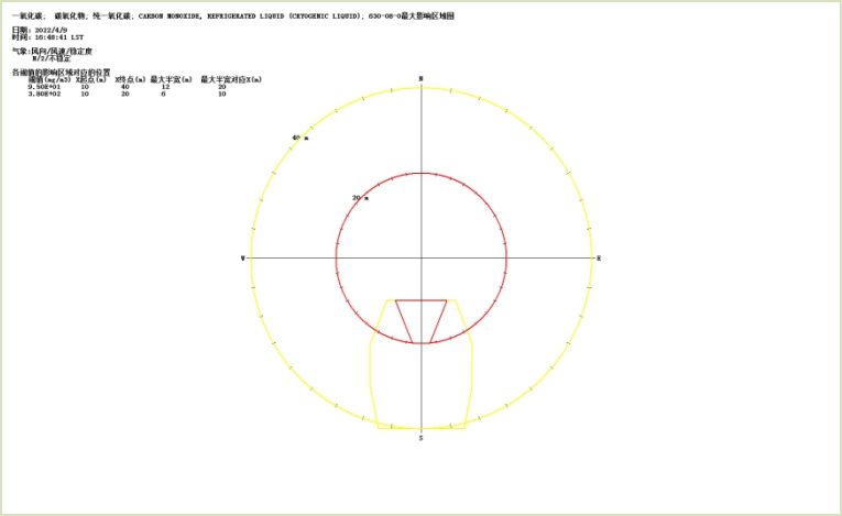
图 6.6-5 苯甲醛泄露火灾次生 CO 扩散环境风险预测结果图
