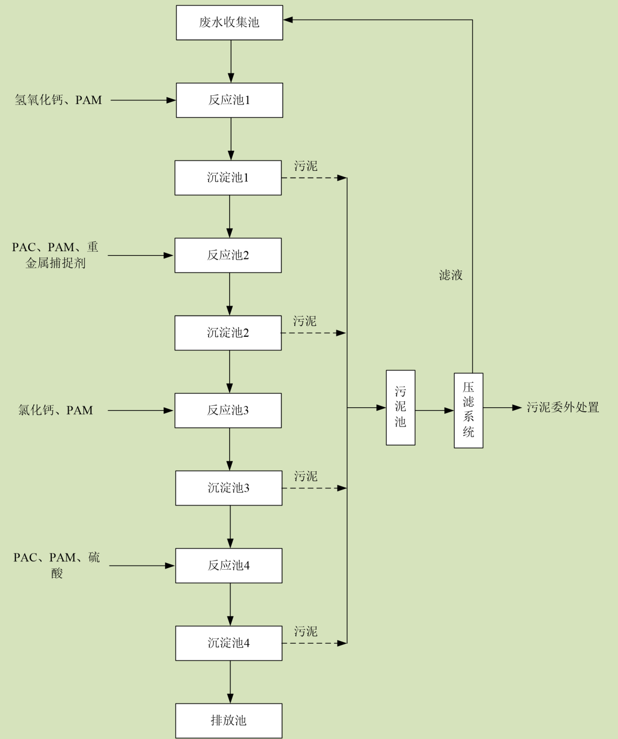
图 7.2-1 废水处理工艺流程图
