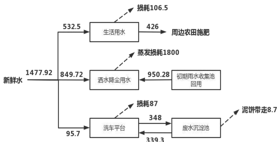
图 4.3-1 项目水平衡关系图 (单位: m³/a)
