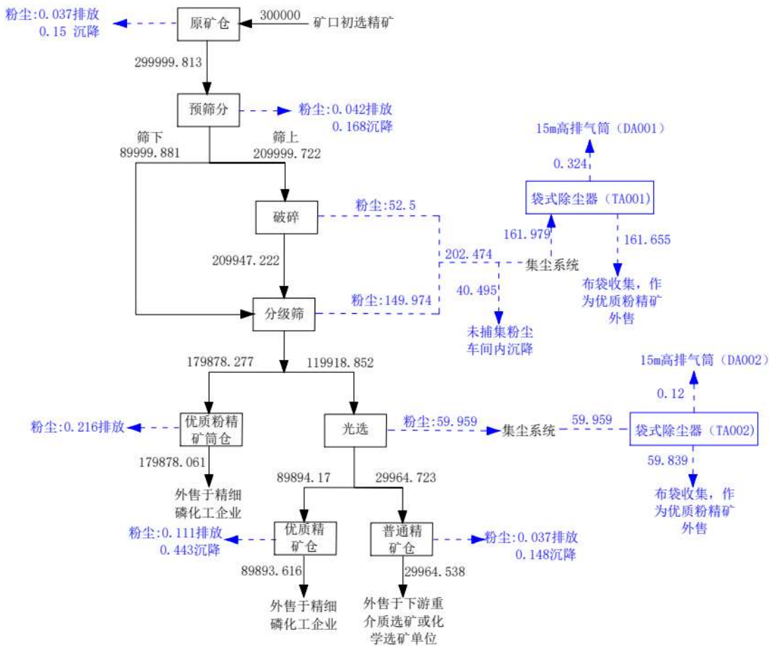
图 4.2-1 项目物料平衡图 (单位: t/a)
