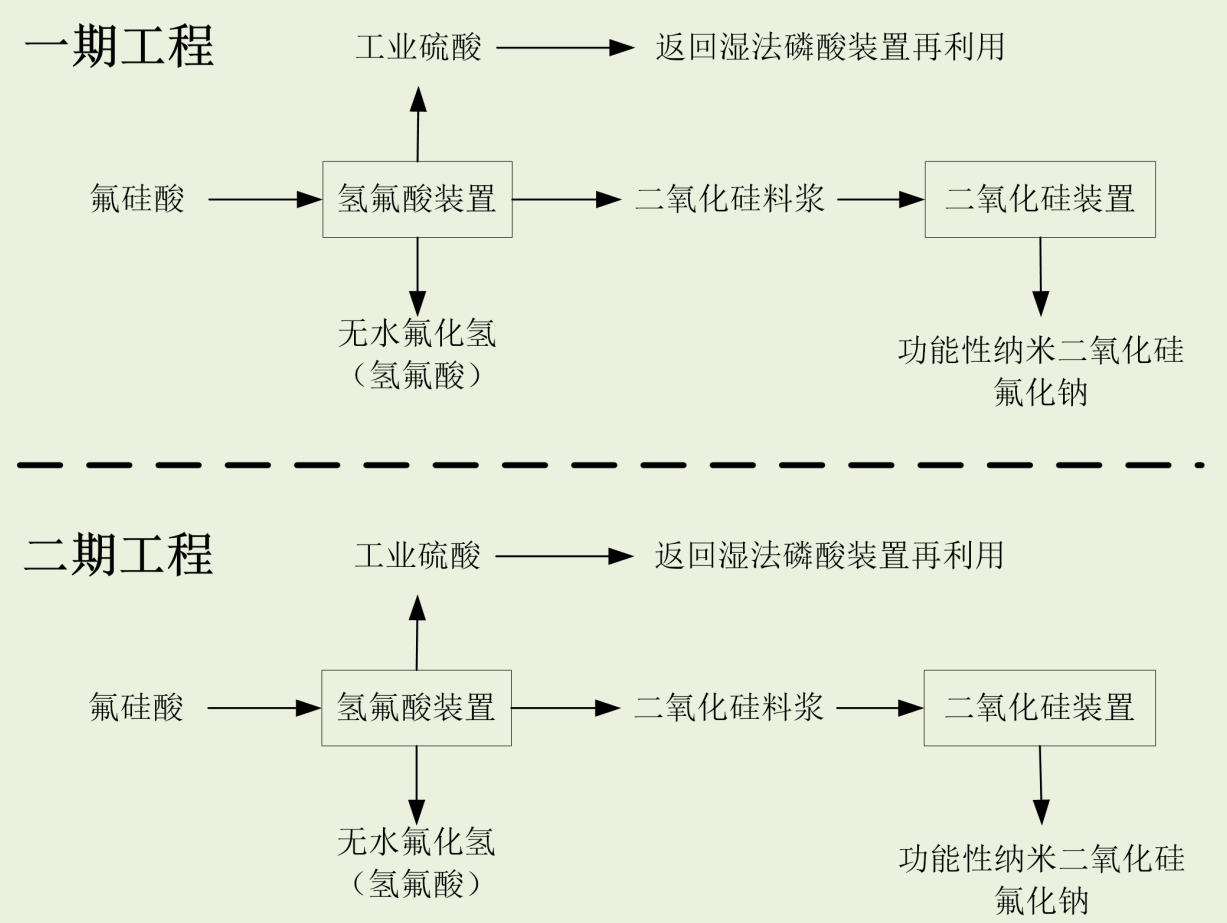
图 2.3-1 项目产品走向图
