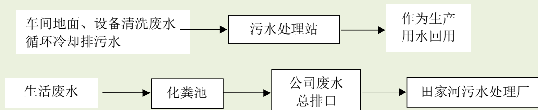
图 7.2-1 项目废水处理流向图
