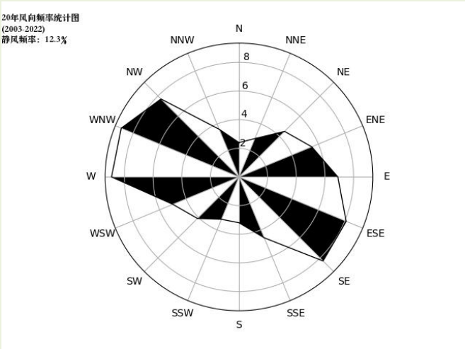
图 5.1-3 宜都风向玫瑰图（静风频率 14.76%）
