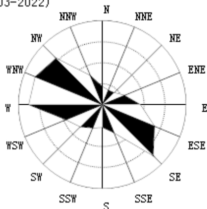
6月风向频率统计图 (2003-2022)
