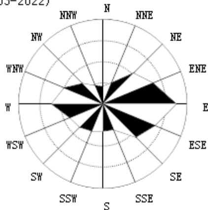
1月风向频率统计图 (2003-2022)
