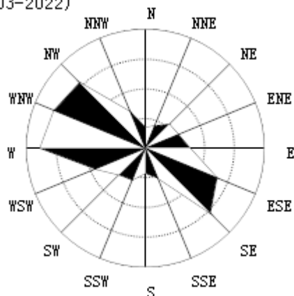
5月风向频率统计图 (2003-2022)
