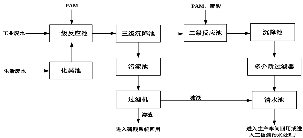
图3.3-1污水处理站工艺流程图
