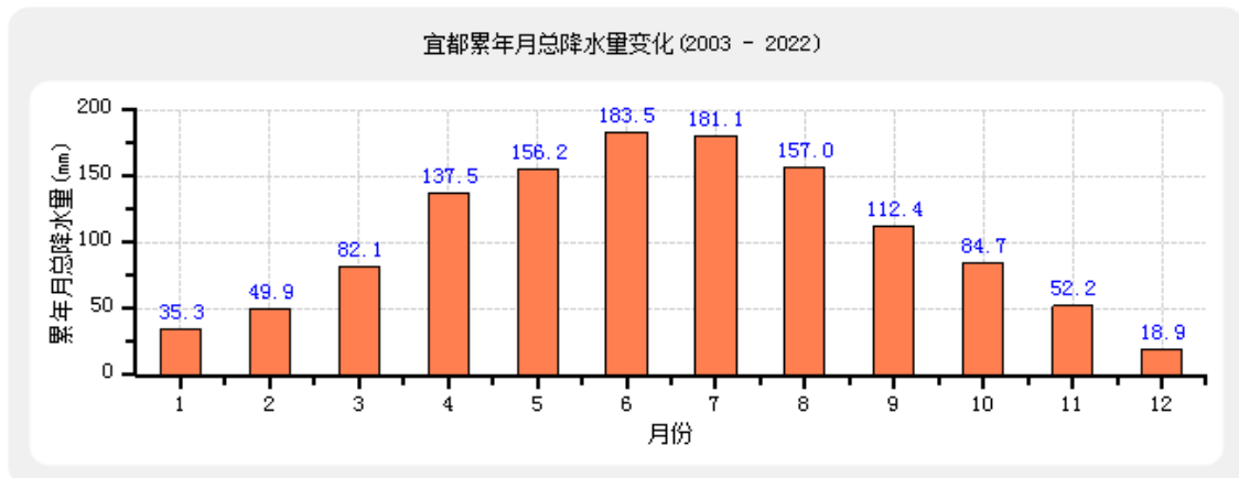
图7.2-5 宜都月平均降水量(单位: 毫米)
