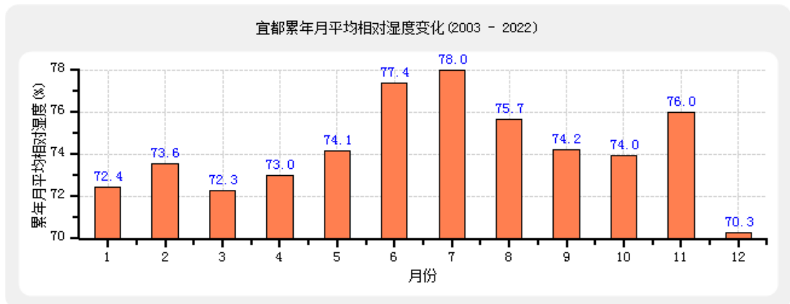
图7.2-9 宜都月平均相对湿度(纵轴为百分比)
