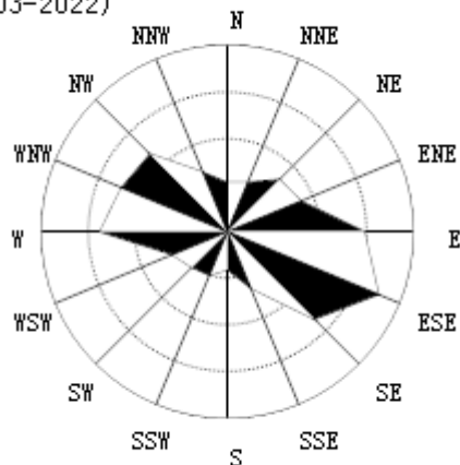
3月风向频率统计图 (2003-2022)
