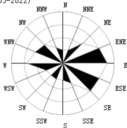
2月风向频率统计图 (2003-2022)
