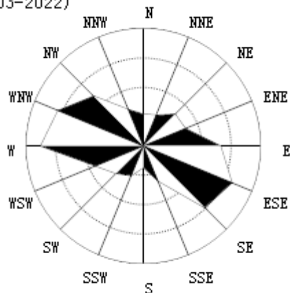
4月风向频率统计图 (2003-2022)
