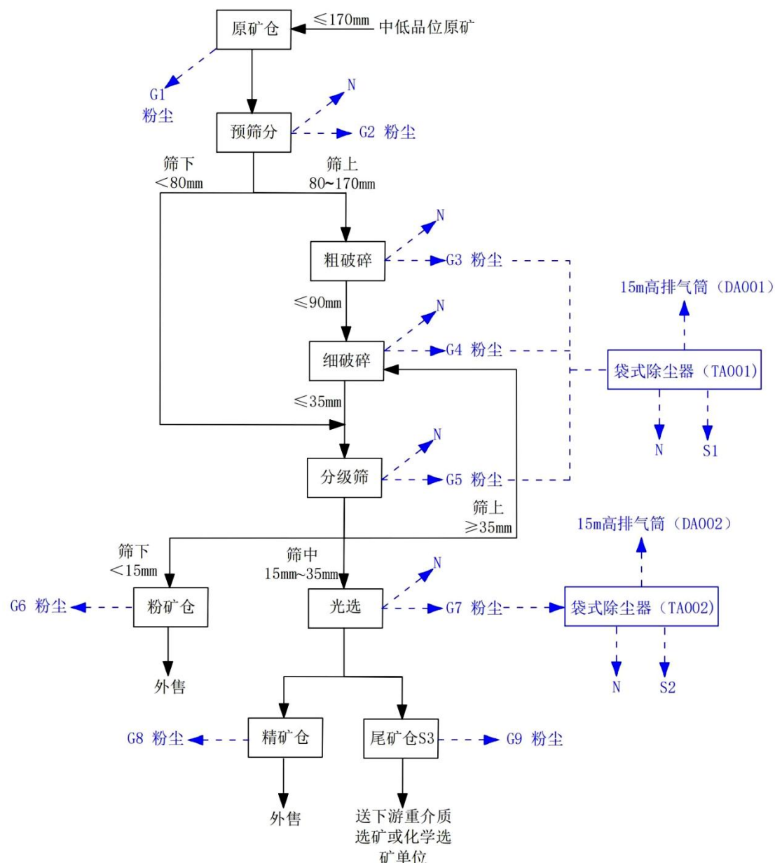
图 4.1-5 项目选矿工程工艺流程及产污环节图
