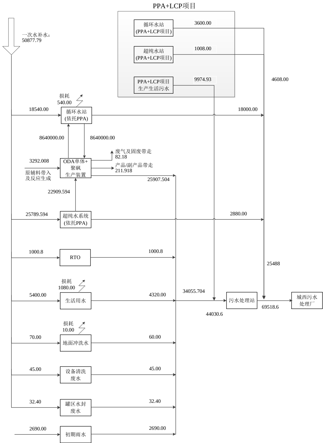
图 3.2-2 在建项目水平衡图（ODA 单体及聚砜产品路线）（单位 \text{m}^3/\text{a} ）
