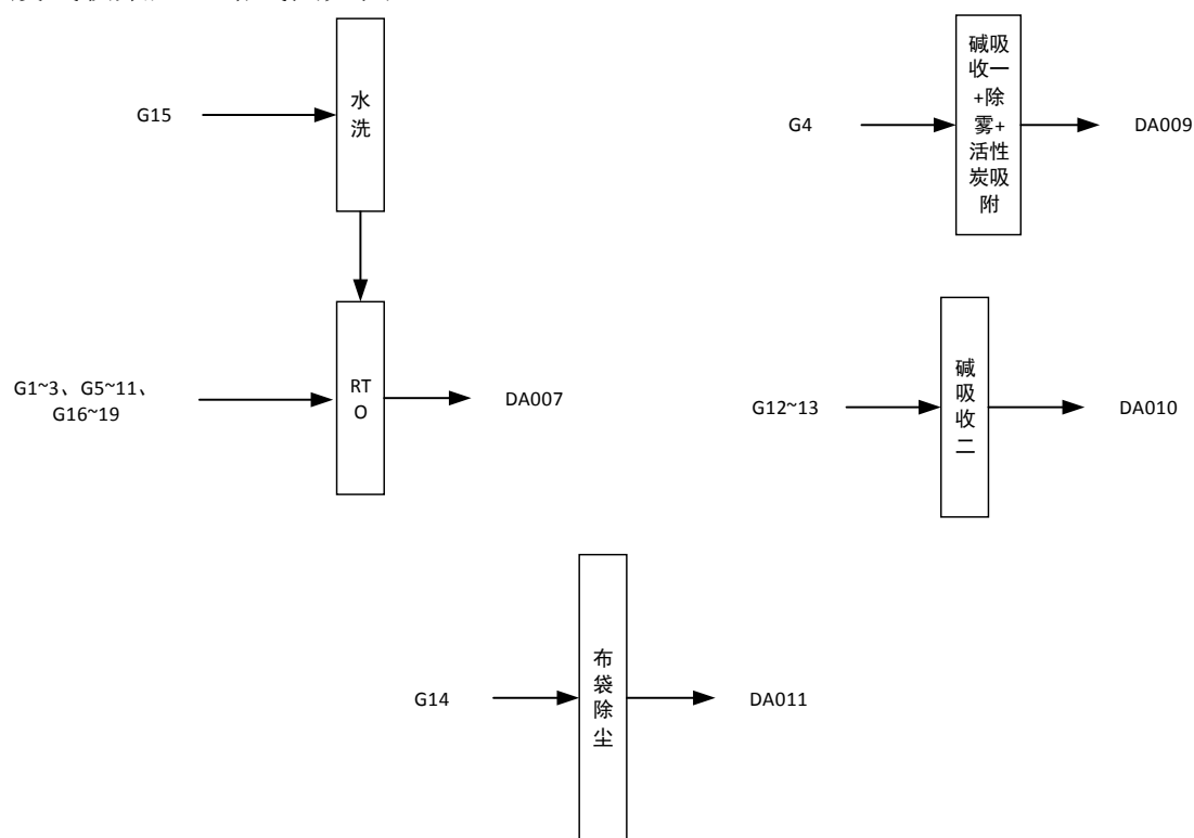
图 10.1-1 废气收集处理路线图
