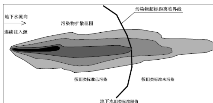
图 8.2.3-2 一维稳定流动一维水动力弥散问题污染物运移示意图
