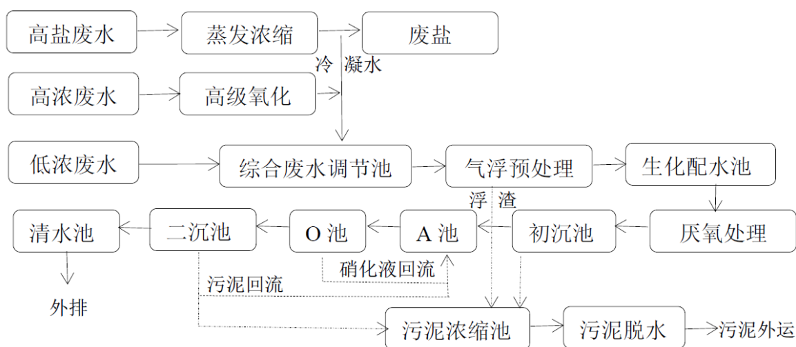
图 10.2.2-1 废水处理路线图
