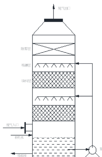
图 10.1.2-2 喷淋吸收工艺示意图
