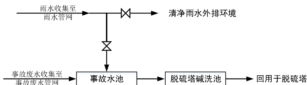
图 8.6.2-1 防止事故水进入外环境的控制、封堵系统图
