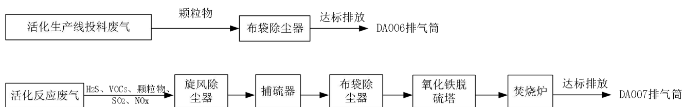
图 9.2-1 项目废气收集、处理走向图
