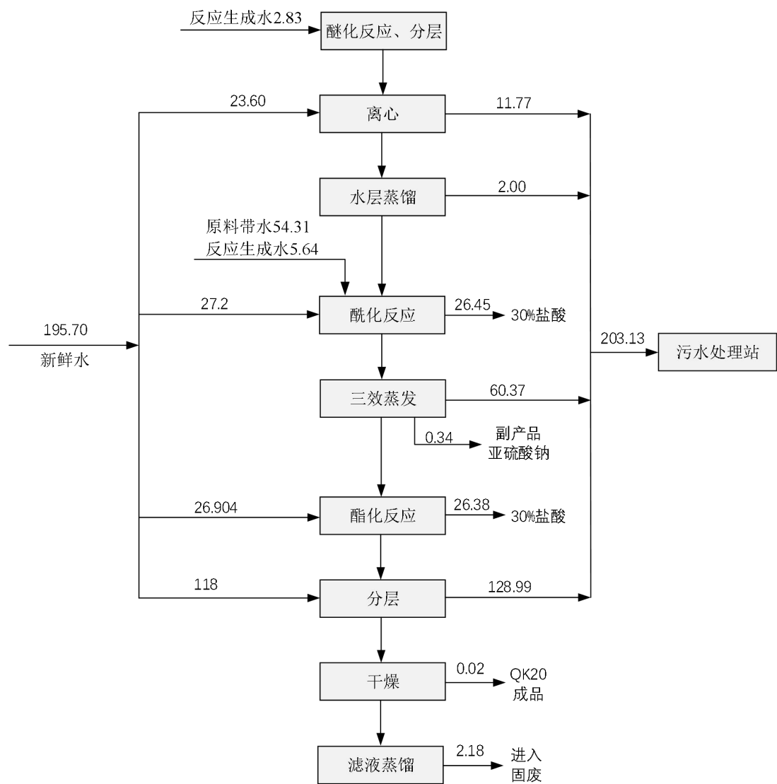
图 4.13-25 QK20 工艺水平衡图 单位：t/a
