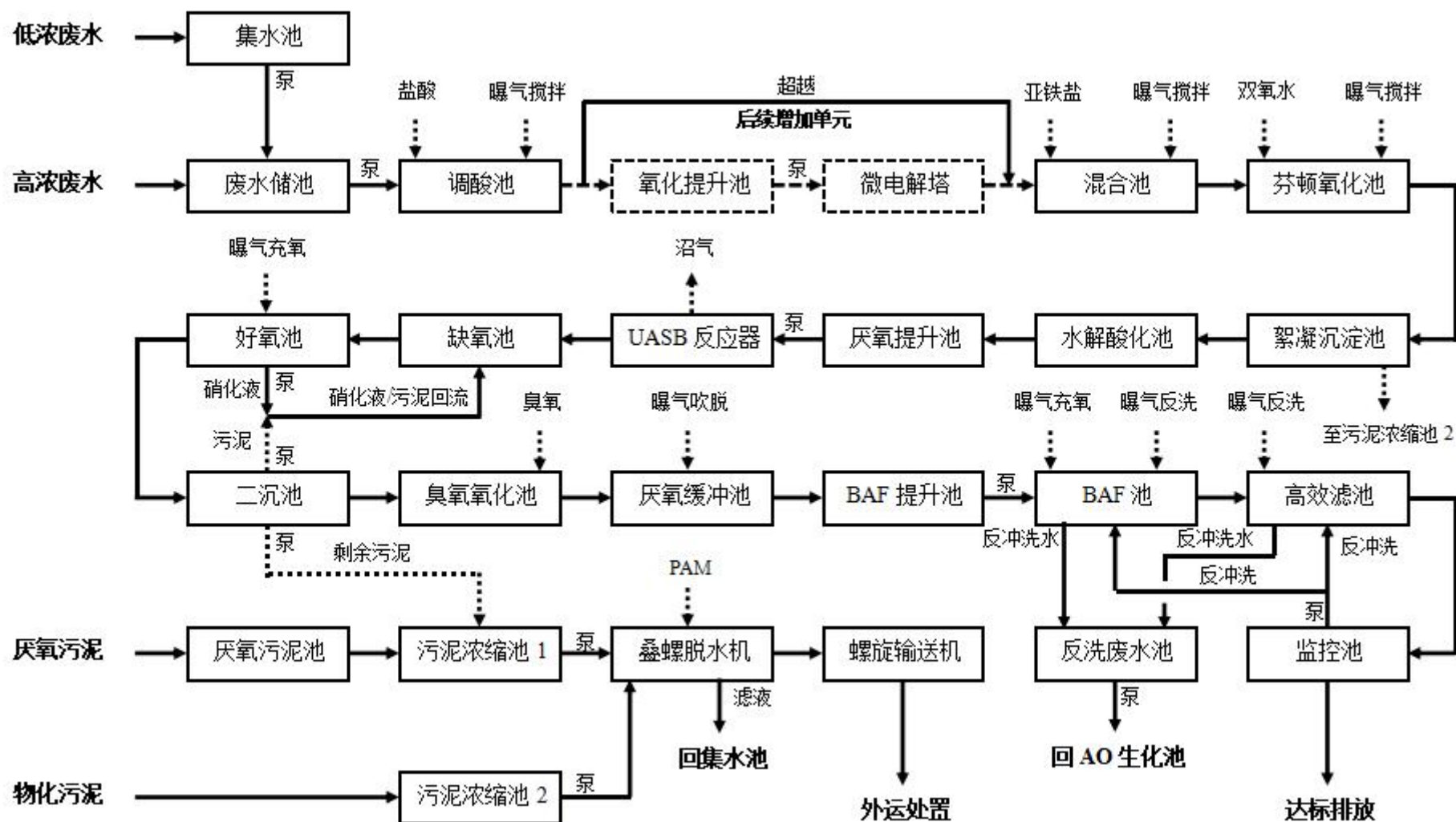
图 8.1-2 综合污水处理工艺流程图
