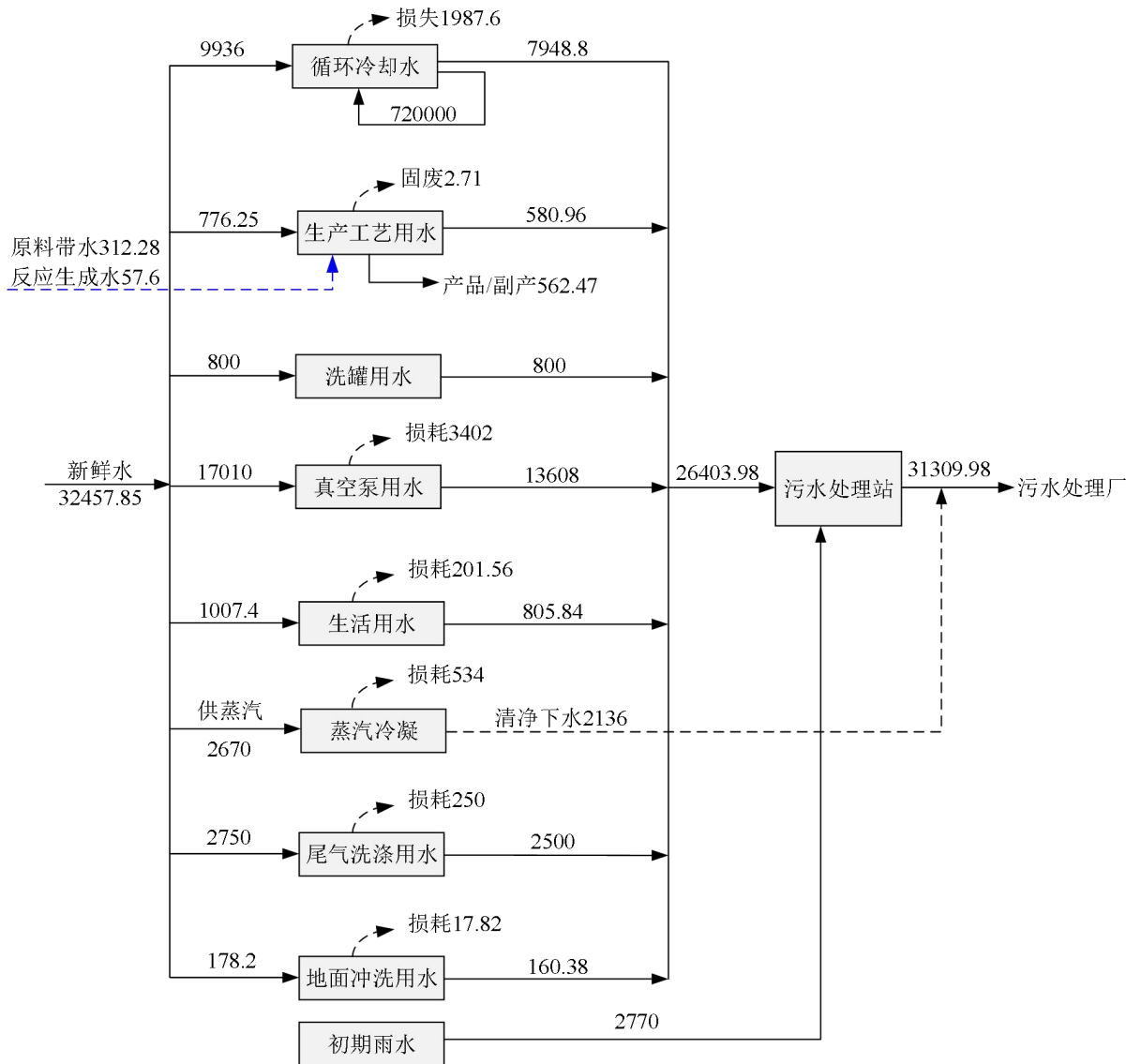
图 4.15-1 中试项目水平衡图 (单位: t/a)
