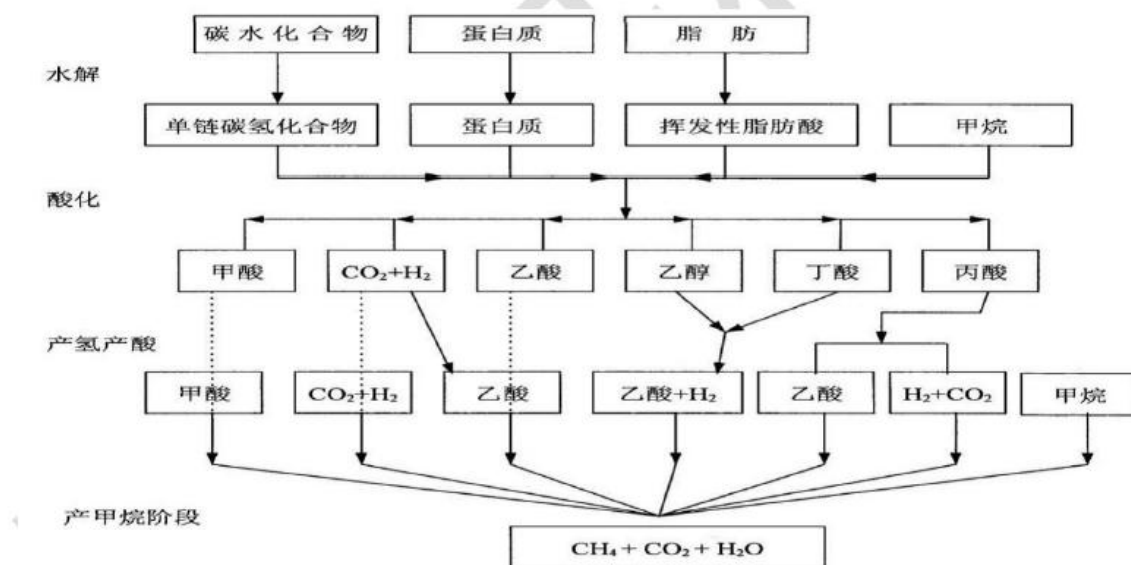
图 8.1-3 厌氧分解图
