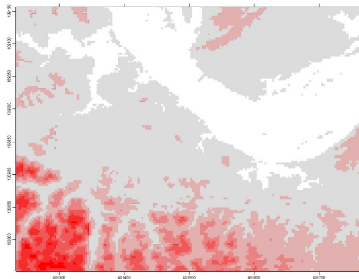
图6.1-9 中试项目所在地地形数据图
