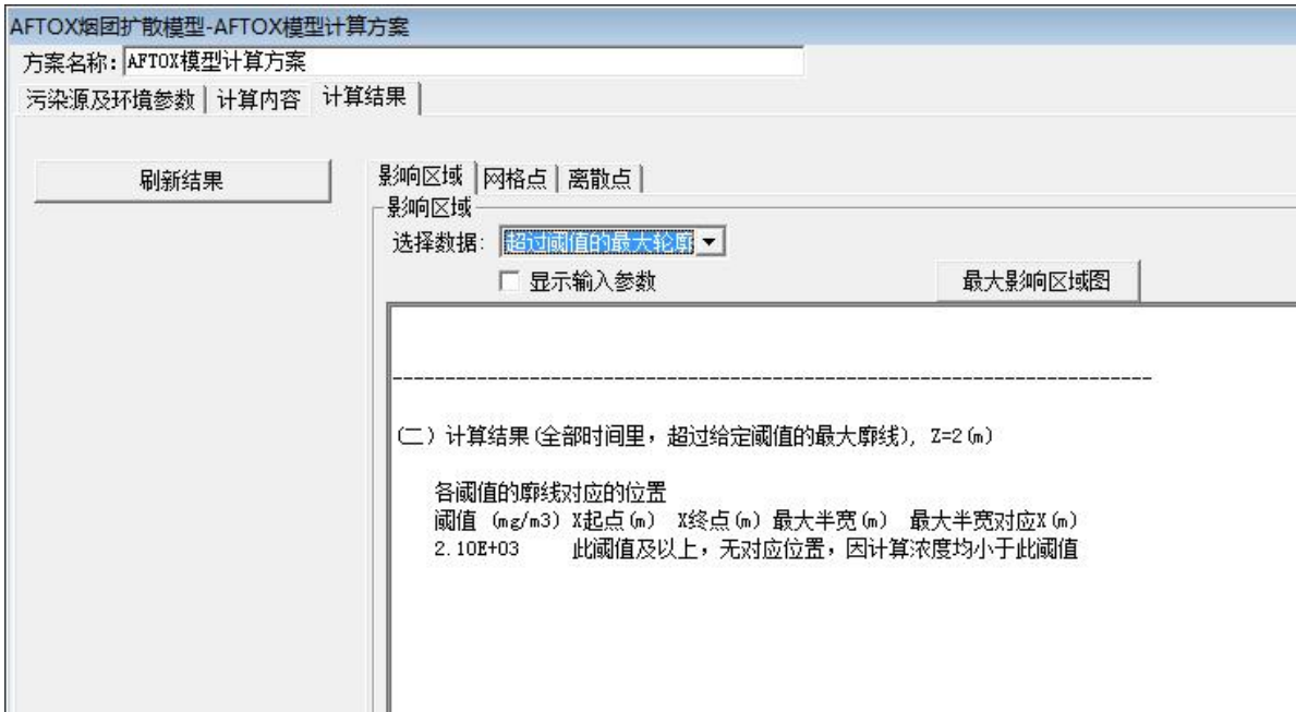
图 7.8-2 甲苯泄漏扩散环境风险预测结果图
