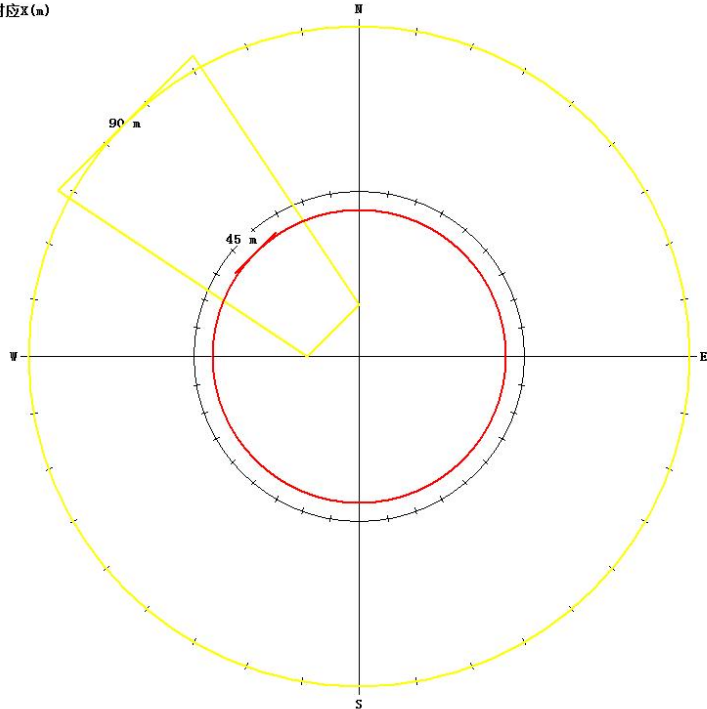
图 7.8-1 盐酸储罐泄漏扩散环境风险预测结果图
