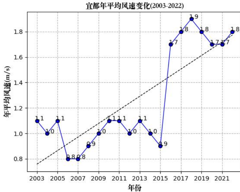
图 6.1-2 宜都（2003-2022）年平均风速（单位：m/s，虚线为趋势线）
