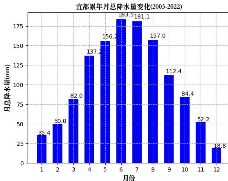
图 6.1-3 宜都月平均降水量（单位：毫米）
