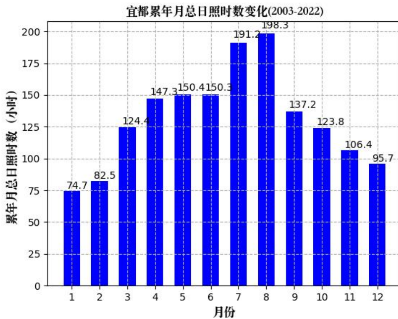
图 6.1-5 宜都月日照时数（单位：小时）
