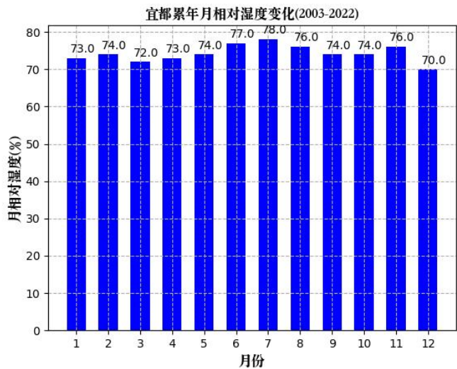
图 6.1-7 宜都月平均相对湿度（纵轴为百分比）
