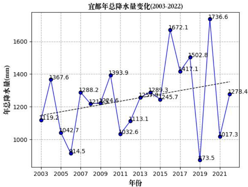
图 6.1-4 宜都（2003-2022）年总降水量（单位：毫米，虚线为趋势线）
