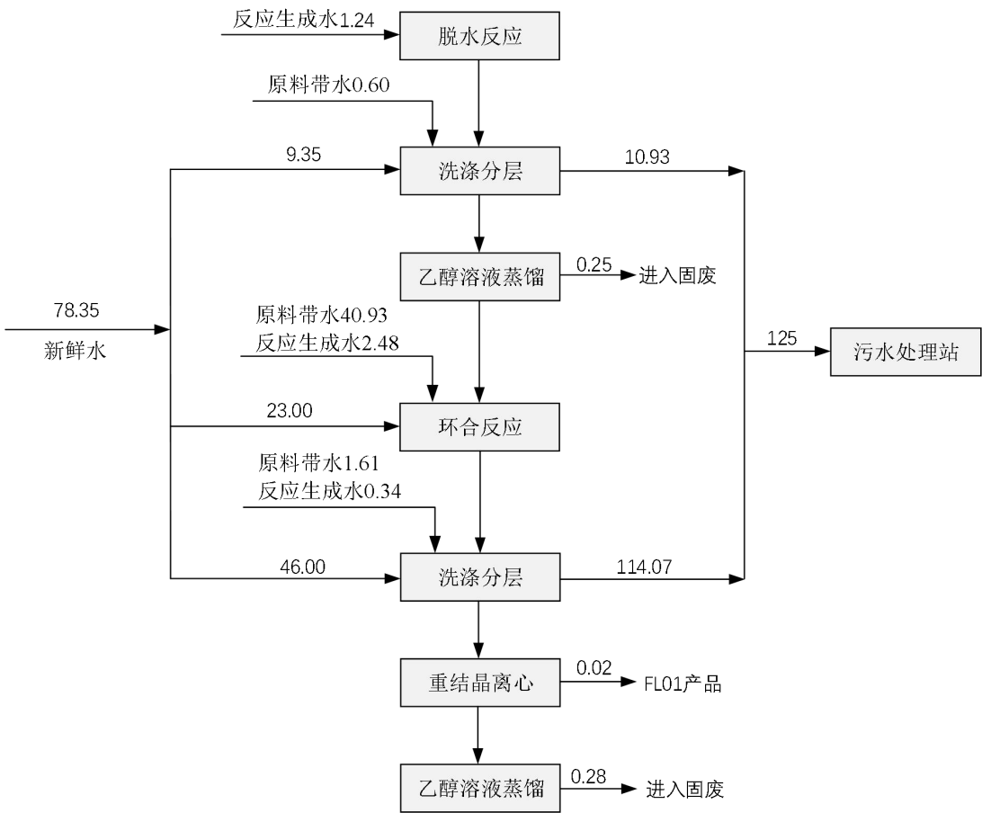
图 4.13-24 FL01 工艺水平衡图 单位: t/a
