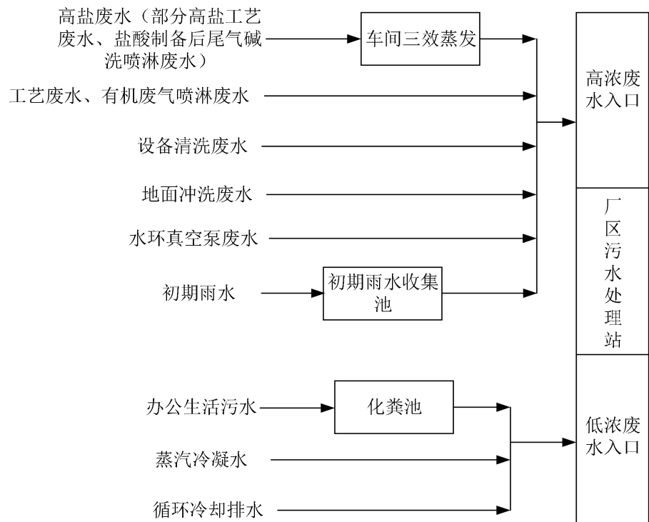
图 8.1-1 项目废水分类分质收集处理示意图
