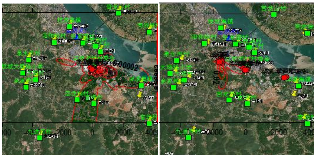
甲醇小时值
