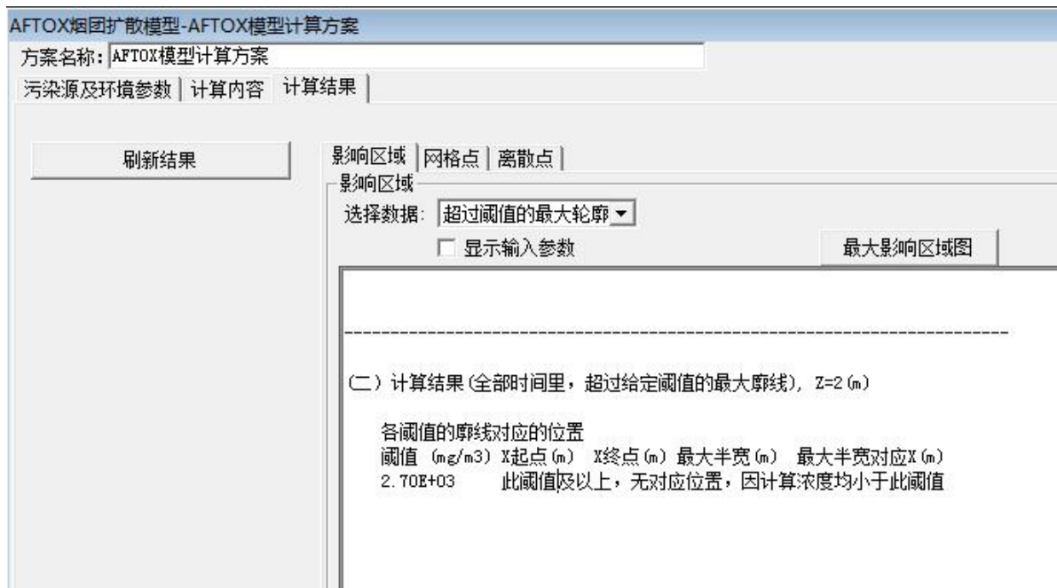
图 7.8-3 甲醇泄漏扩散环境风险预测结果图
