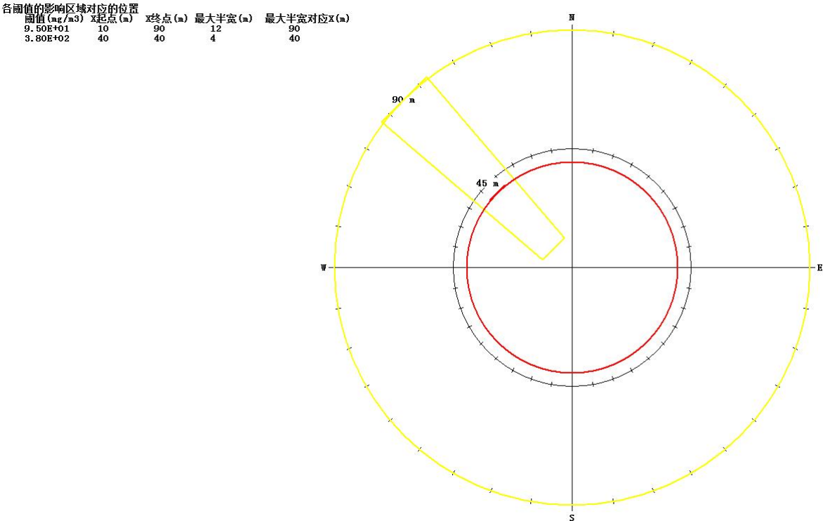
图 7.8-8 甲醇泄露火灾次生 CO 扩散环境风险预测结果图
