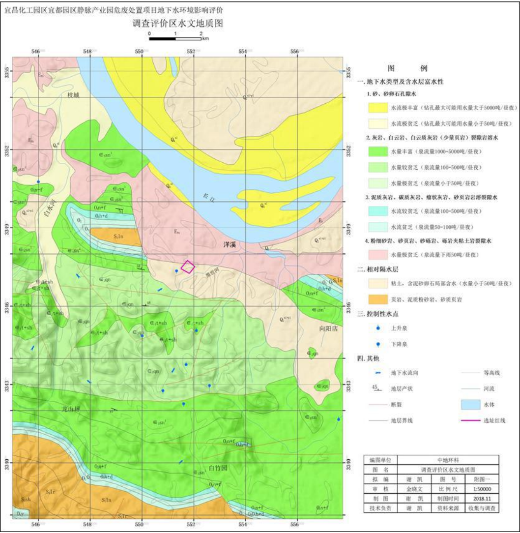
图 6.4-1 中试项目所在区域 1：50000 水文地质图
