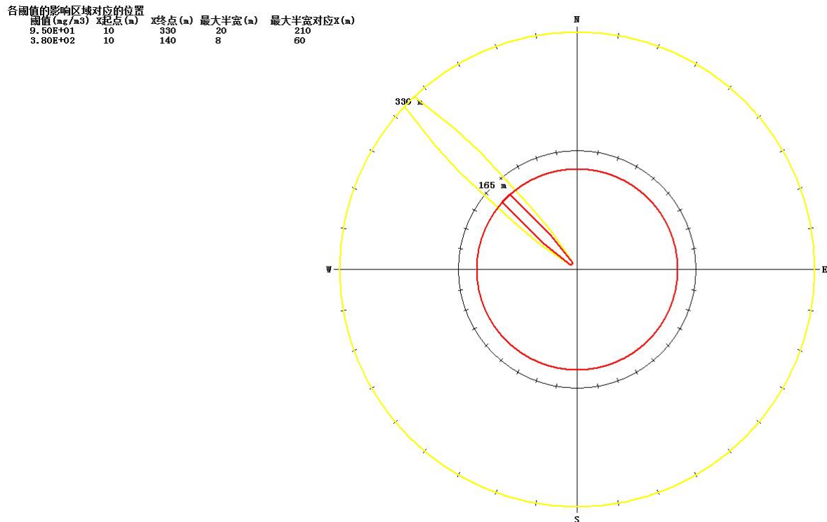
图 7.8-10 甲苯泄露火灾次生 CO 扩散环境风险预测结果图
