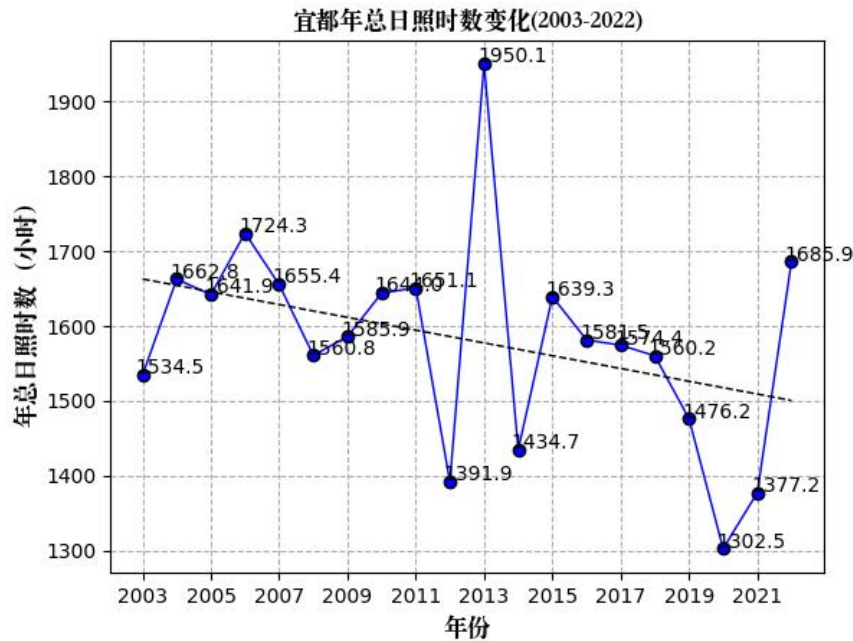
图 6.1-6 宜都（2003-2022）年日照时长（单位：小时，虚线为趋势线）
