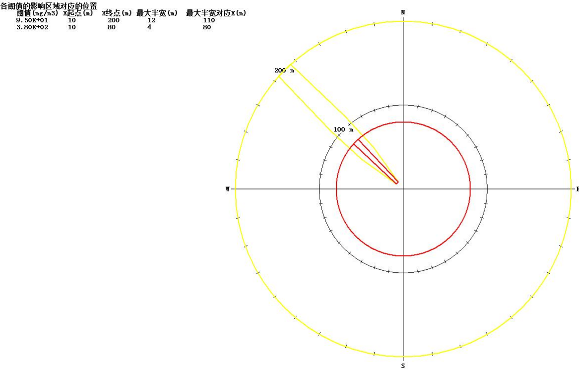
图 7.8-10 四氢呋喃泄露火灾次生 CO 扩散环境风险预测结果图
