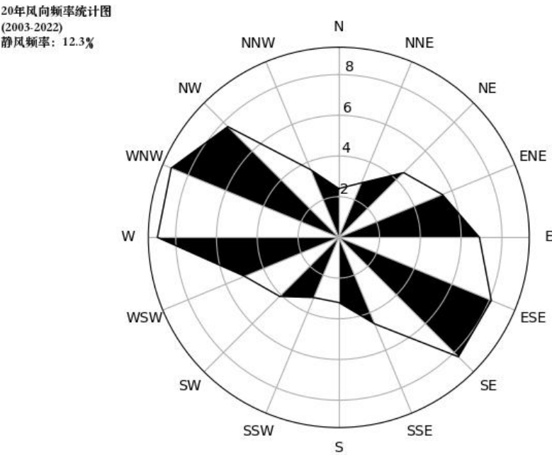
图 6.1-1 宜都风向玫瑰图（静风频率 12.3%）
