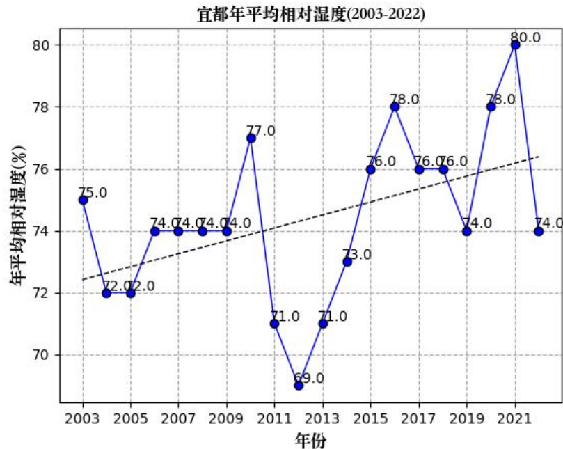
图 6.1-8 宜都（2003-2022）年平均相对湿度（纵轴为百分比，虚线为趋势线）
