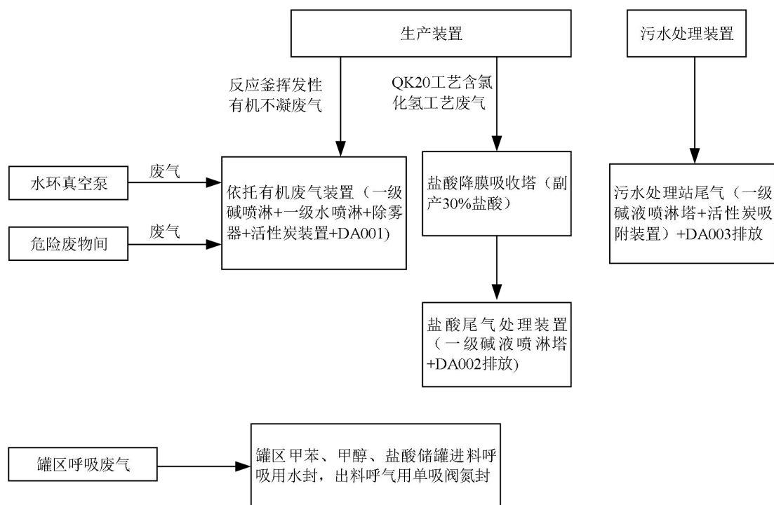
图 8.2-1 中试项目废气收集处理方案路线图
