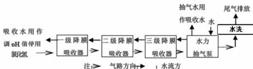
图 7.1-1 氯化氢尾气三级降膜吸收工艺流程
