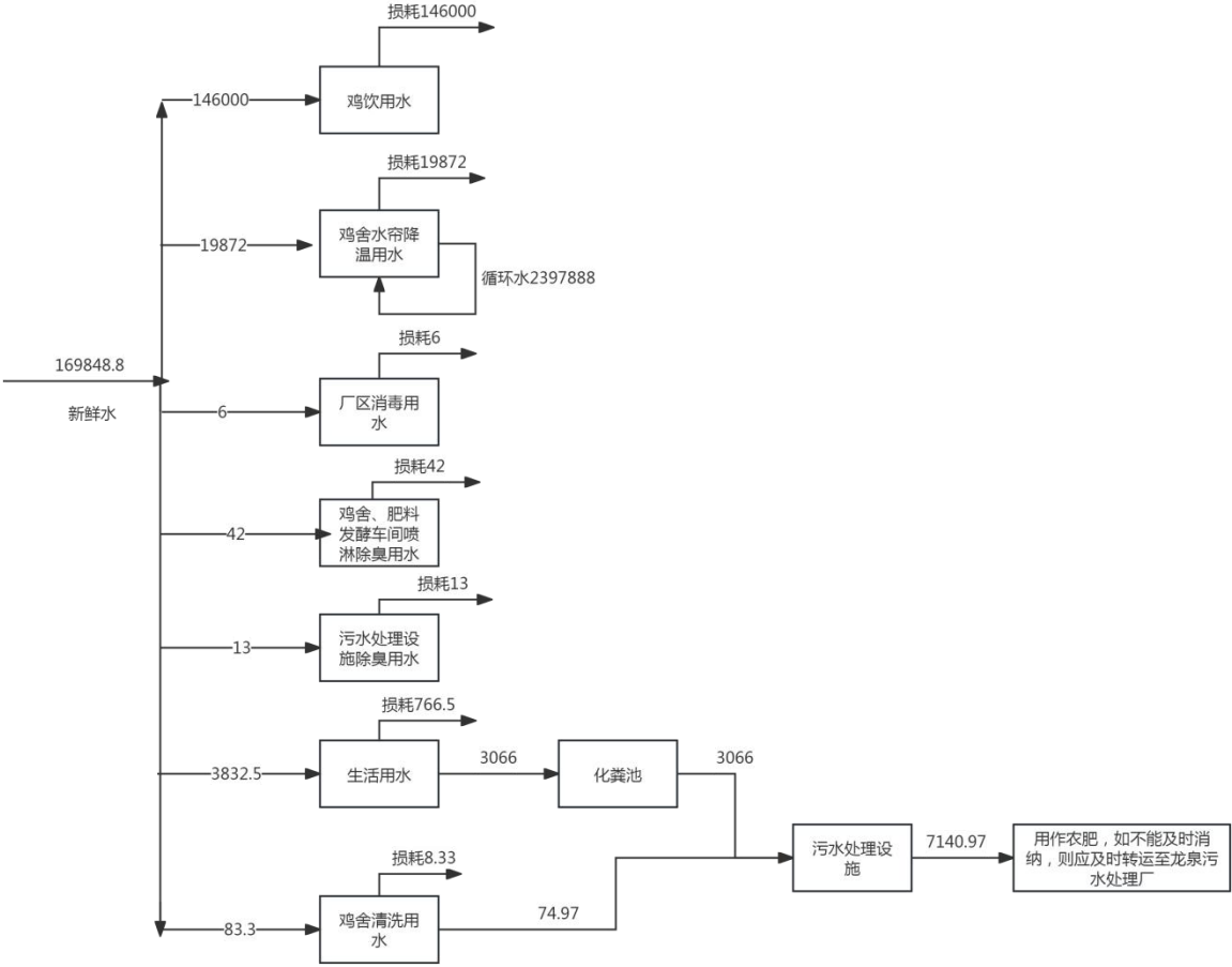
图4.1-5 水平衡示意图 单位：m³/a
