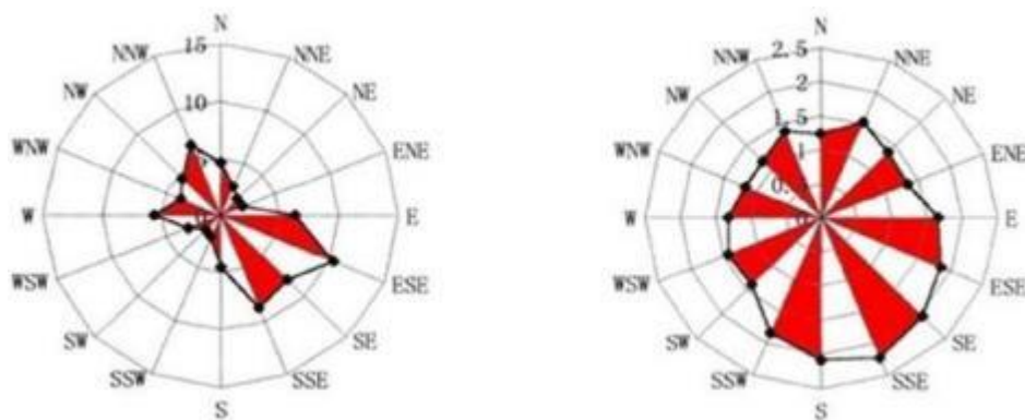
图7.2-5 风玫瑰图
