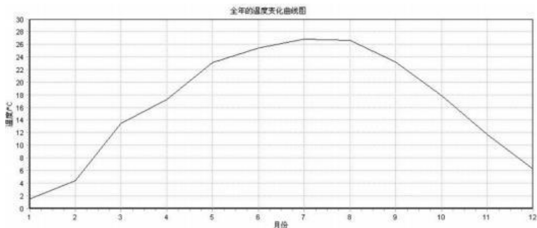
图7.2-2 全年温度变化曲线图
