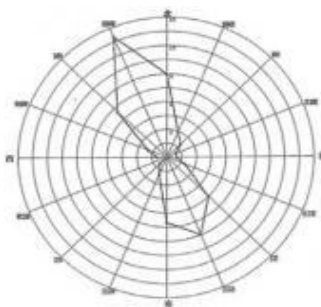
图7.2-1 风向频率玫瑰图
