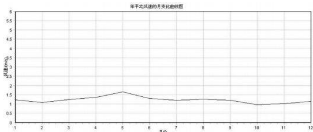
图7.2-3 全年风速变化曲线图
