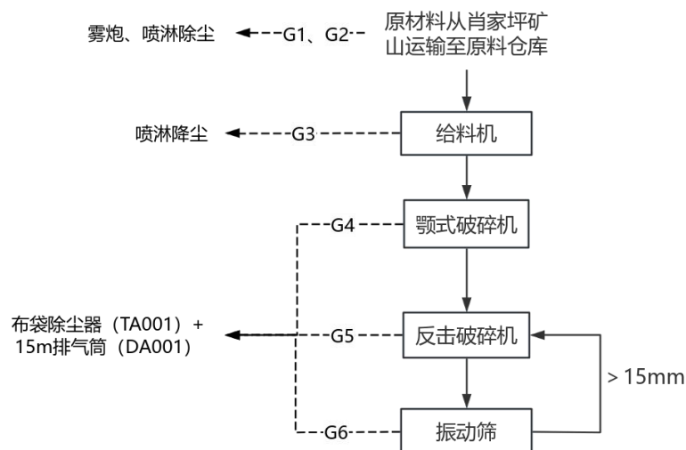
图9.2-1 项目废气流向及废气治理设施示意图
