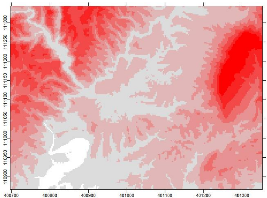
图7.2-6 项目所在地地形高程图
