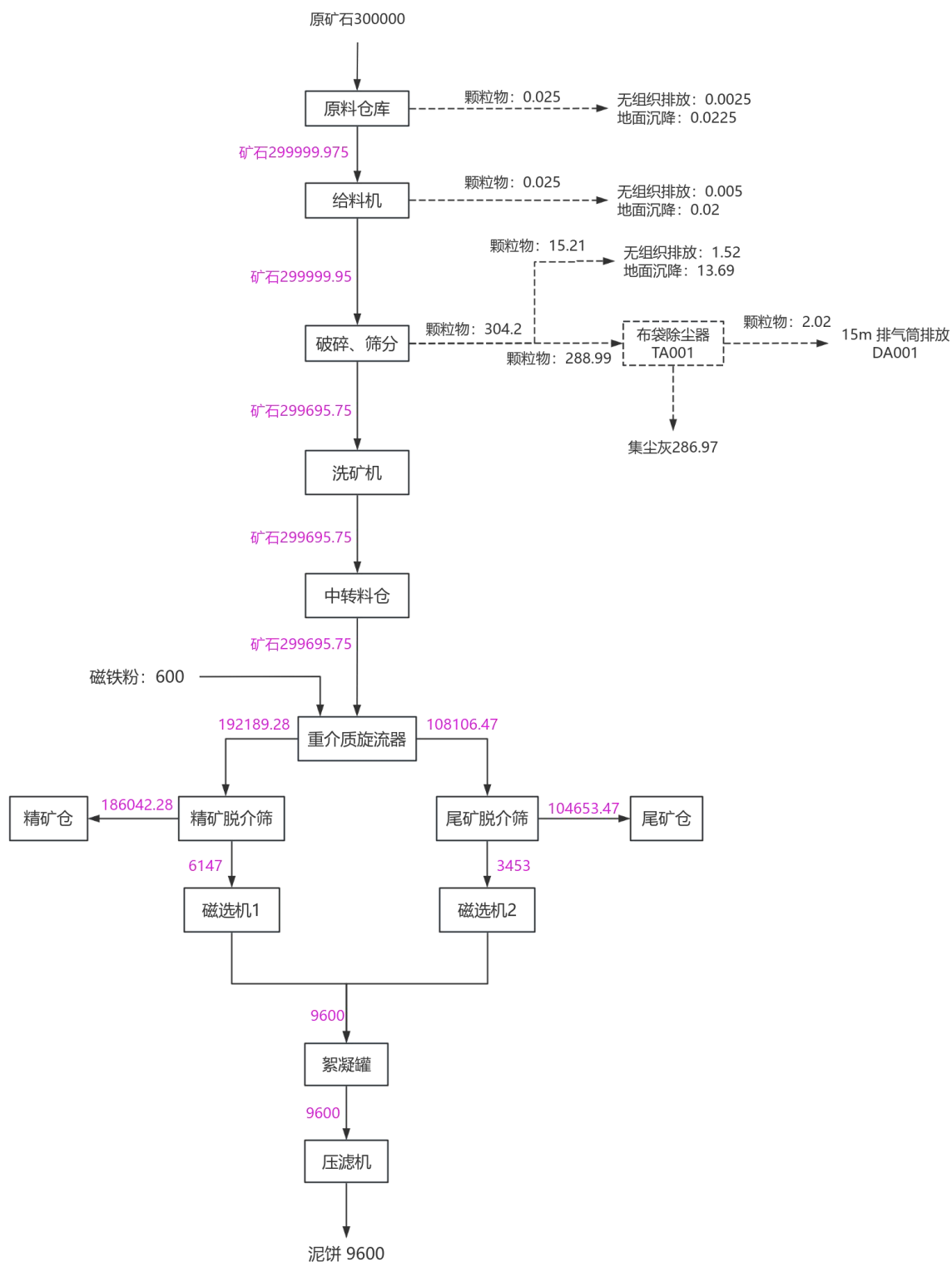
图 5.4-1 项目物料平衡图 (单位: t/a)
