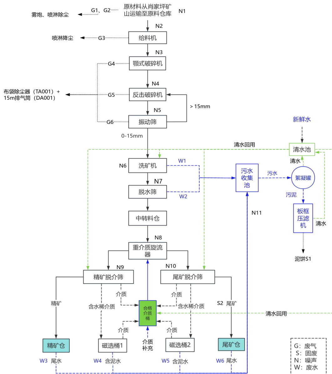
图5.3-1 项目工艺流程图
