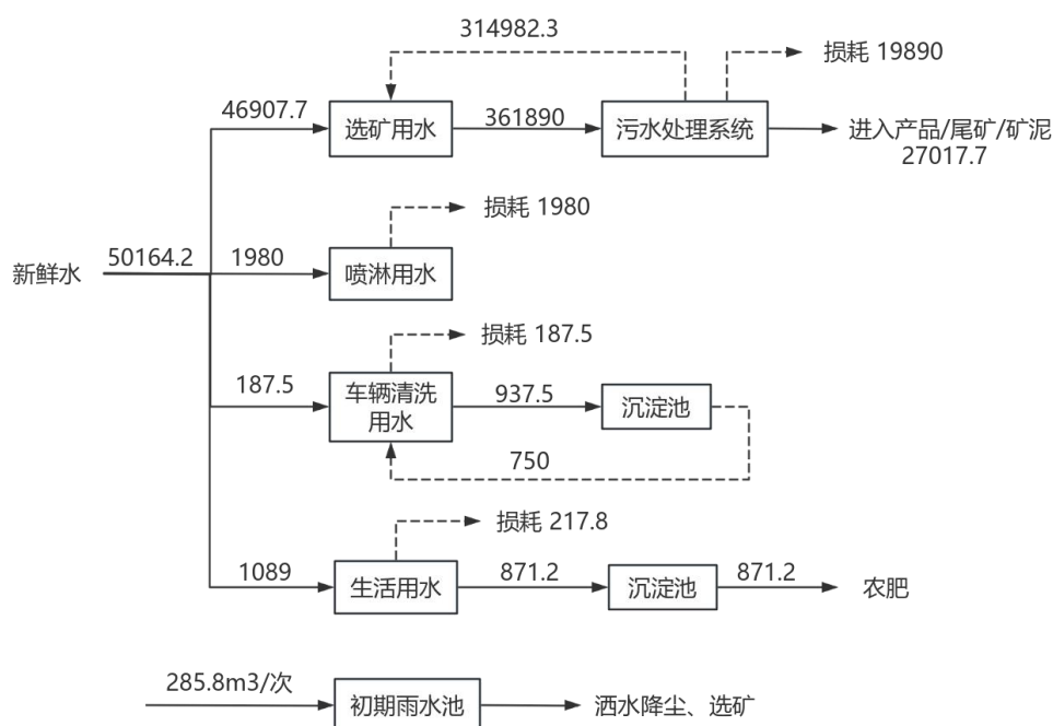
图 5.5-1 本项目水平衡图（单位：m 3 /d）
