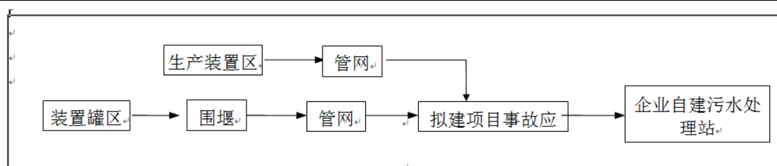
图 8.9-1 事故三级防控体系图
