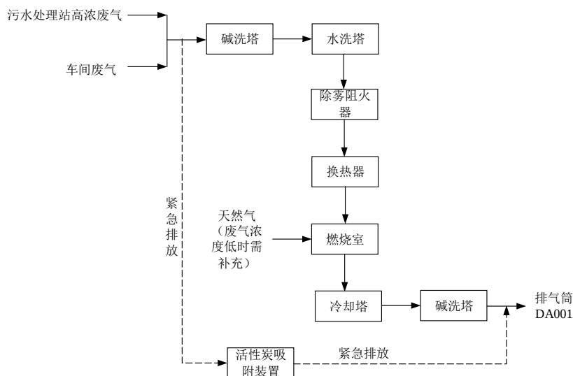
图 9.2-2 RTO 废气处理工艺流程图
