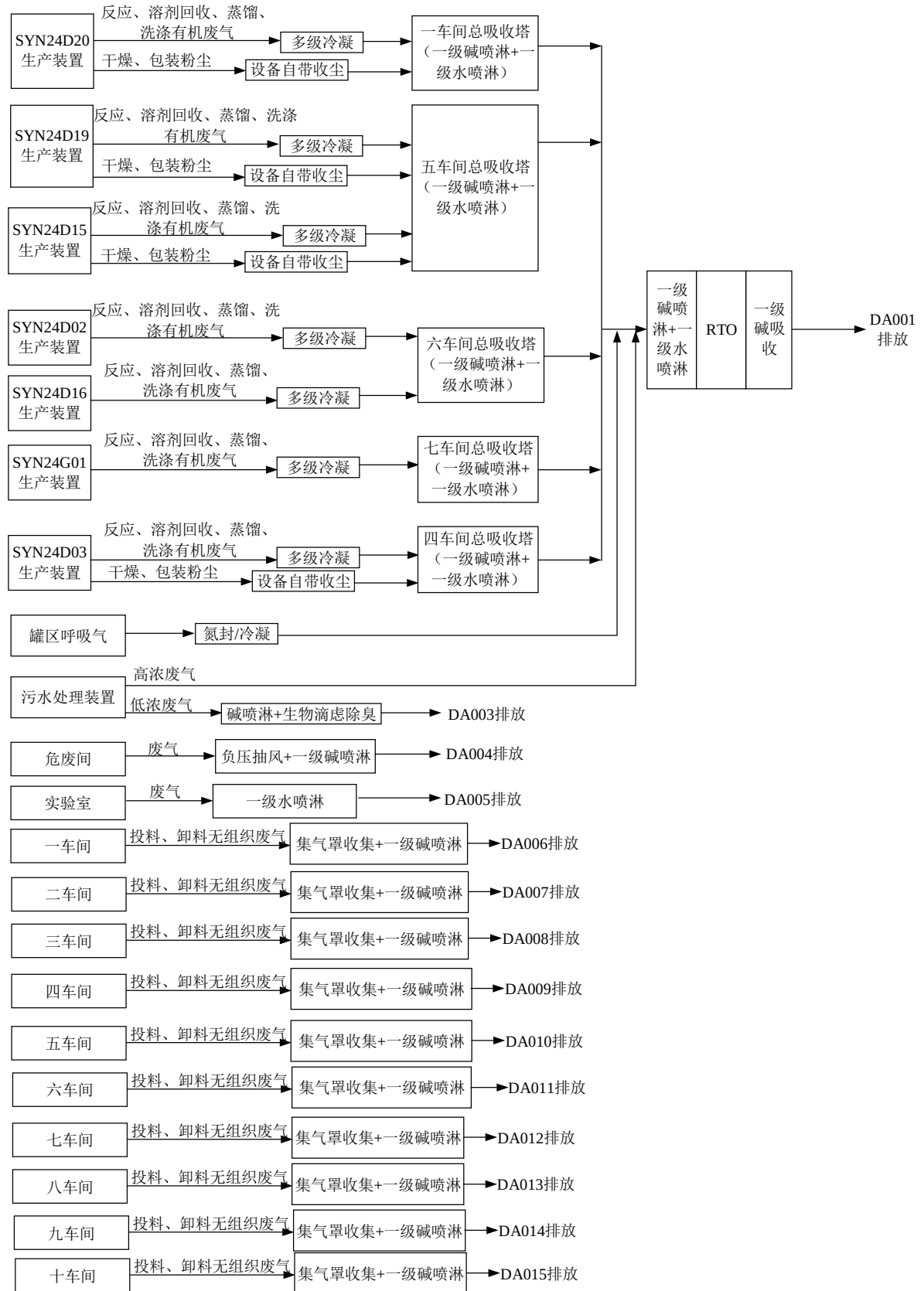
图 9.2-1 本项目废气收集处理方案路线图
