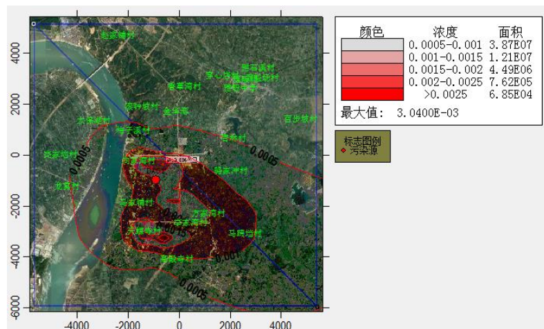
NO x 叠加年平均浓度
