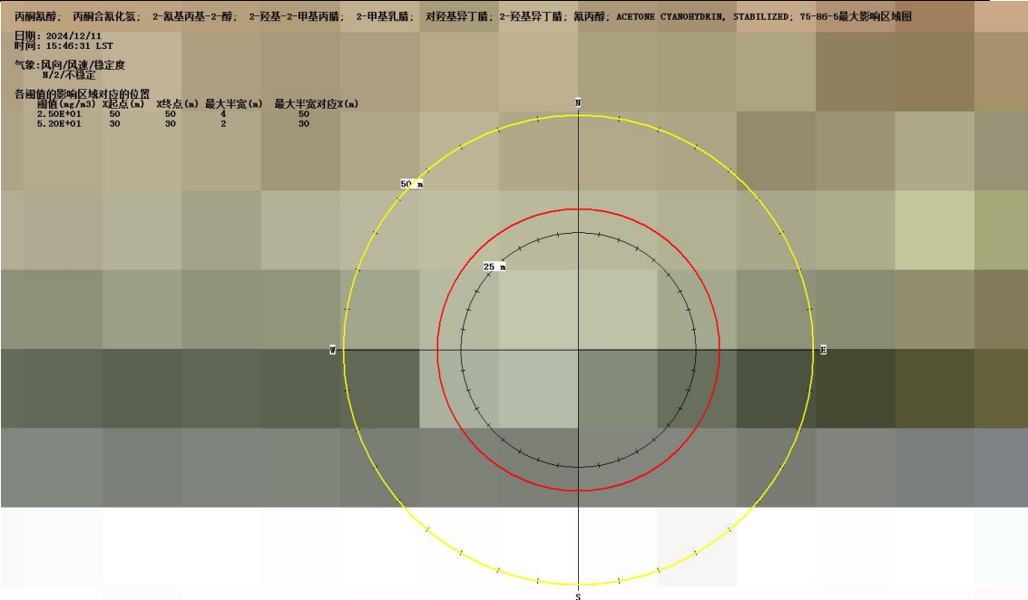
图 8.8-1 丙酮氰醇泄漏环境风险预测结果图
