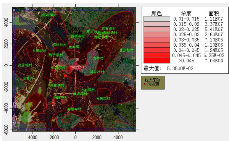
NO x 叠加小时平均浓度
