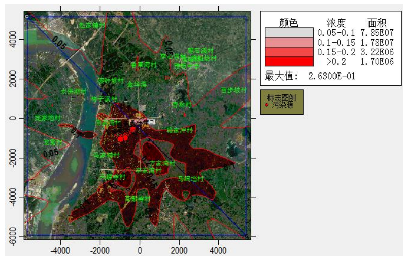
TVOC 叠加小时值平均浓度
