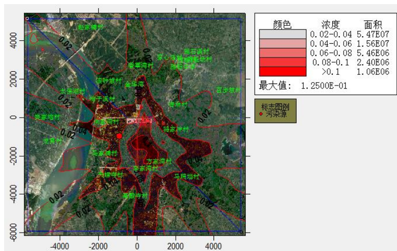
PM 10 叠加小时平均浓度
