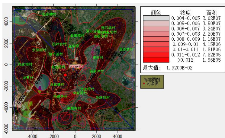
SO 2 叠加小时平均浓度
