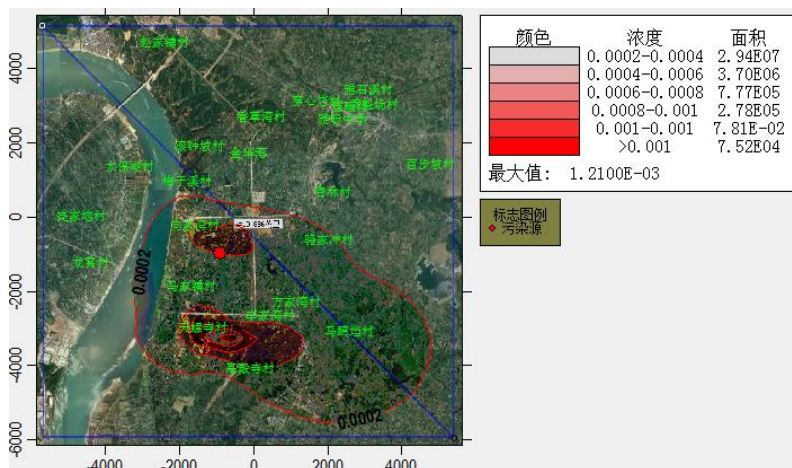
SO 2 叠加年平均浓度
