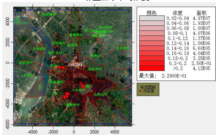
甲醇叠加小时平均浓度
