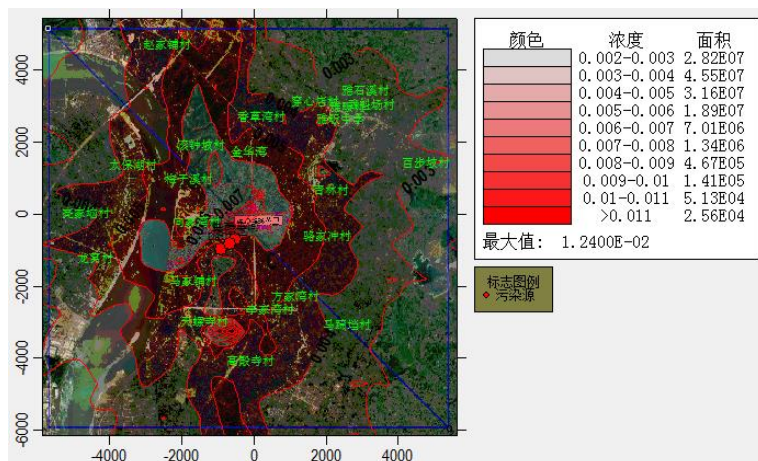
HCl 叠加小时值平均浓度
