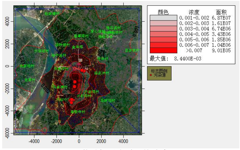
甲苯叠加后小时平均浓度
