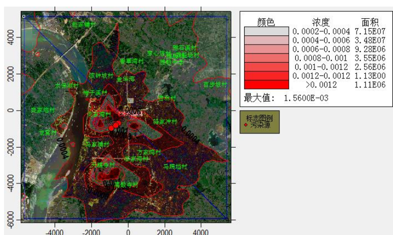
HCl 叠加日值平均浓度
