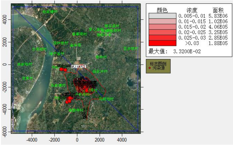
甲醇叠加日平均浓度
