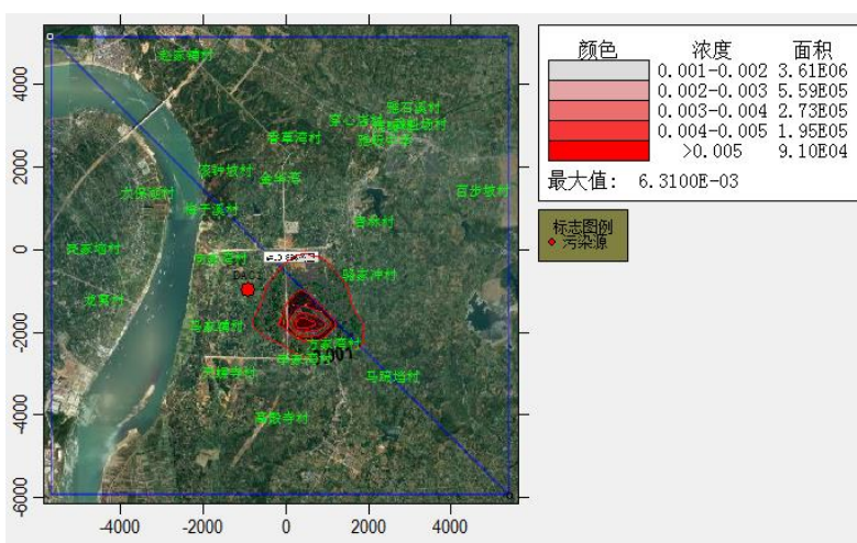
PM 10 叠加年平均浓度
