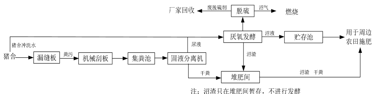
图 6.2-1 粪污处理工艺流程图
