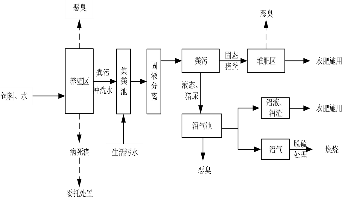
图 3.2-4 项目产污环节示意图
