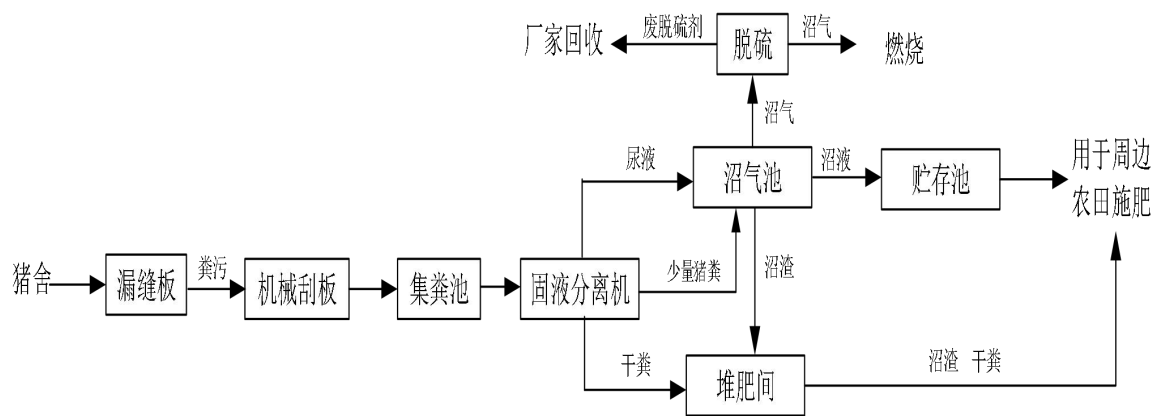
图 3.2-3 粪污处理工艺流程图
