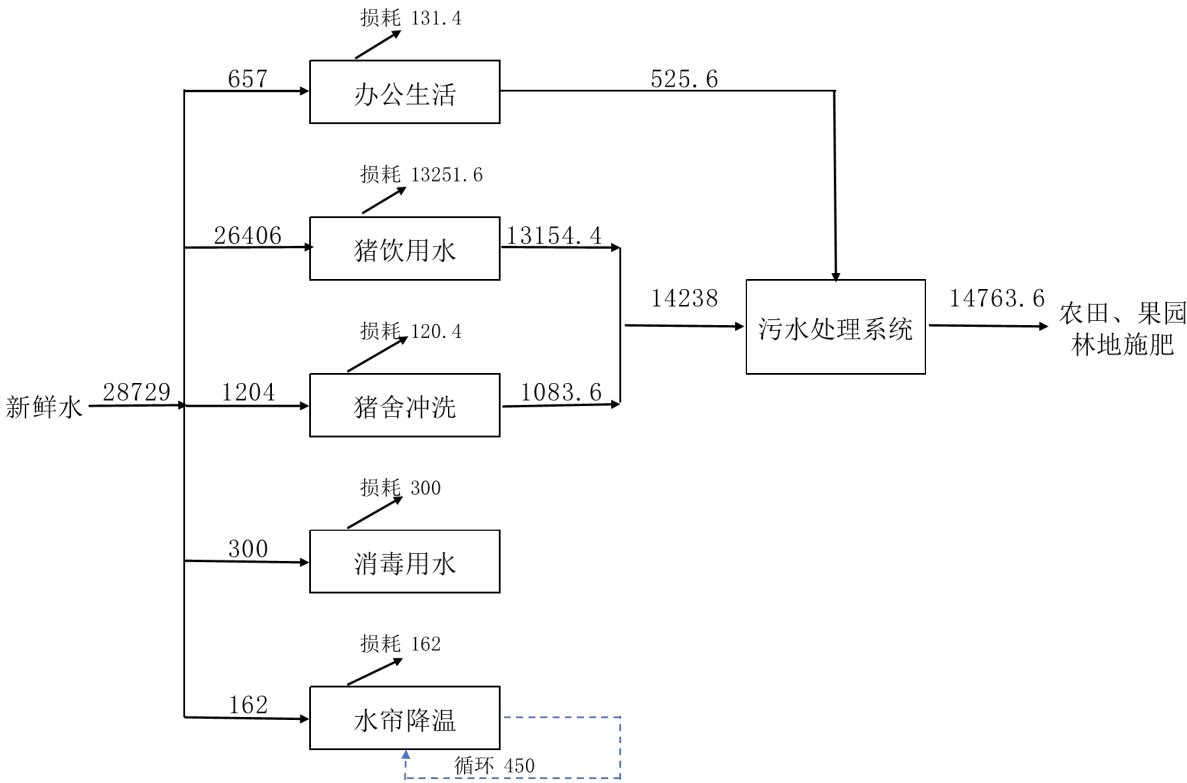
图 3.2-5 项目给排水平衡图 (单位: t/a)
