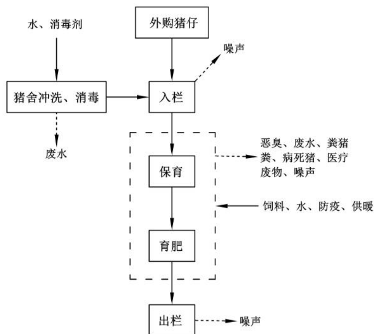
图 3.2-1 养殖工艺流程图
