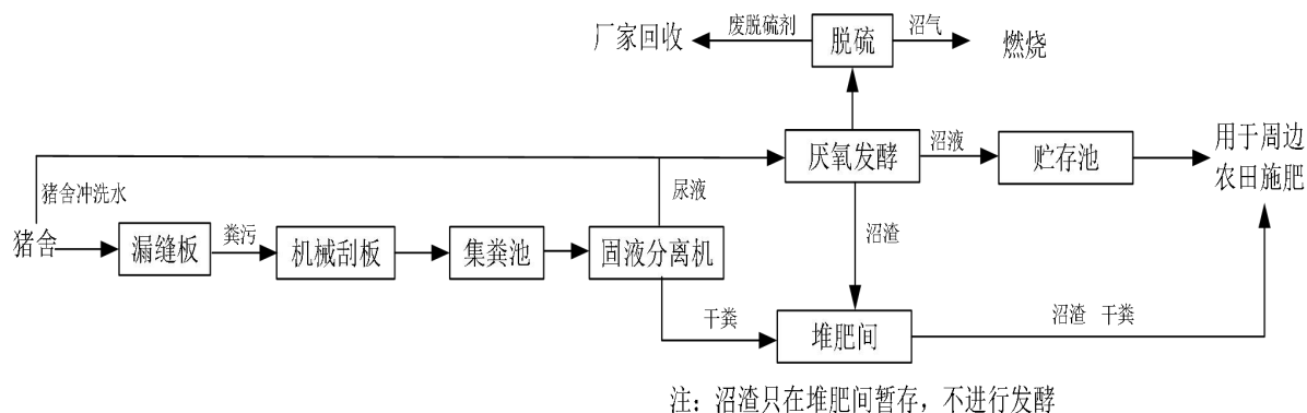
图 8.2-1 粪污处理工艺流程图
