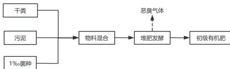
图 3.3-3 干粪堆肥发酵工艺流程图
