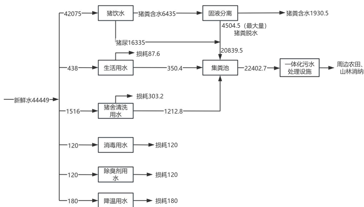
图 3.3-5 项目给排水平衡图（单位：t/a）
