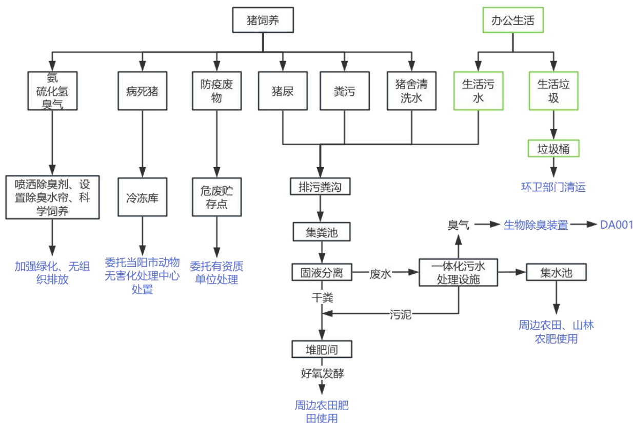
图 3.3-4 项目产污环节示意图
