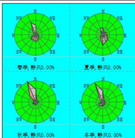
图 5.2-5 荆门地区 2022 年各季风频玫瑰图
