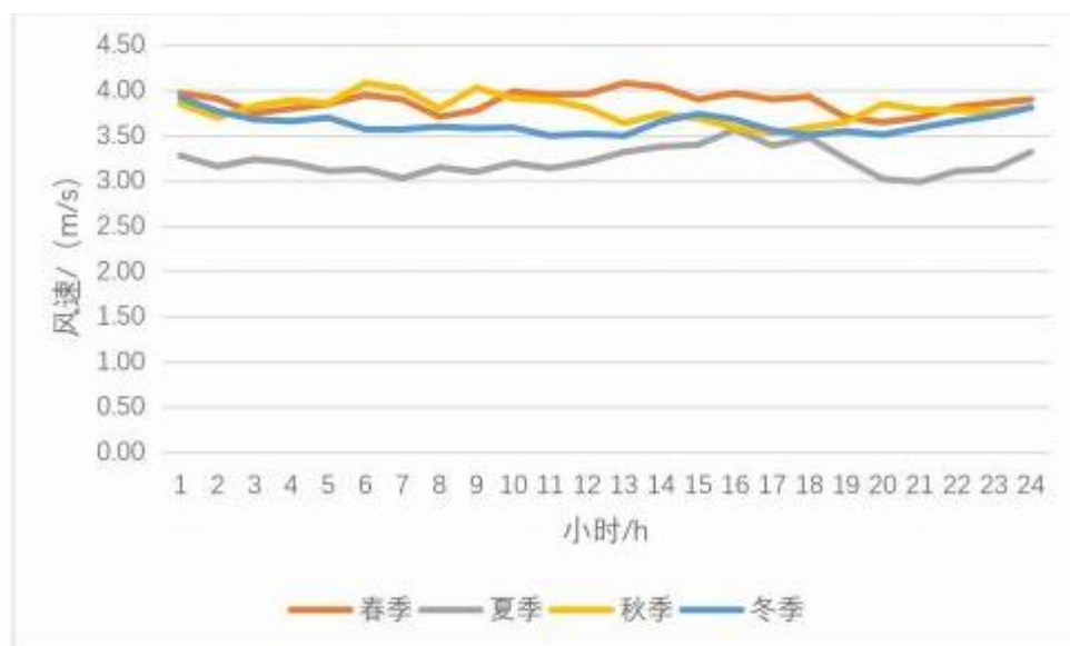
图 5.2-4 荆门地区 2022 年季平均风速小时变化图
