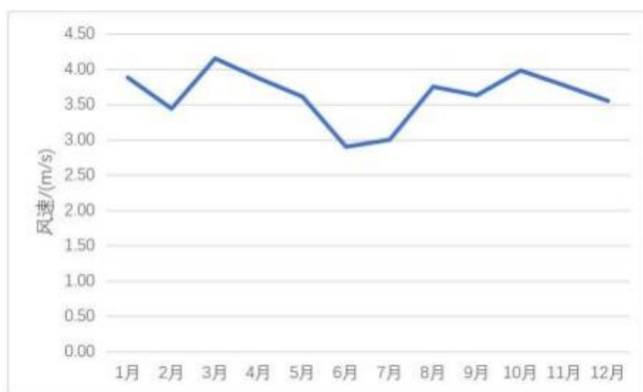
图 5.2-3 荆门地区 2022 年平均风速月变化图
