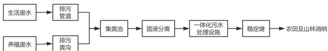
图 5.2-8 项目废水处理流程图
