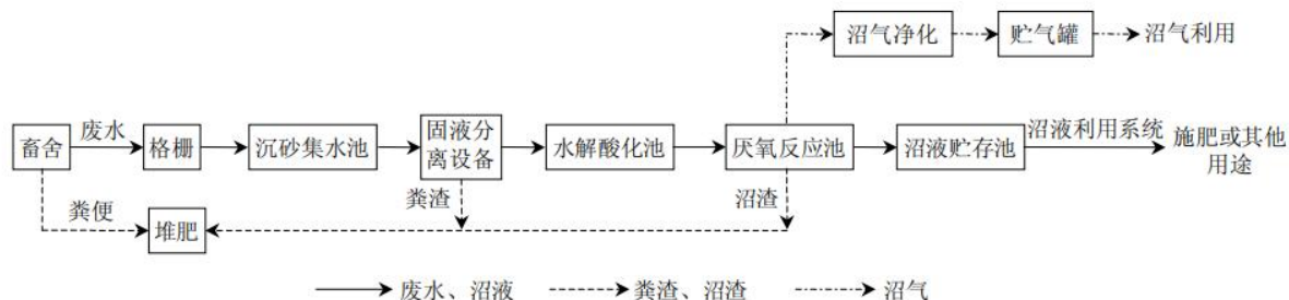
图 7.2-1 模式II工艺基本流程
