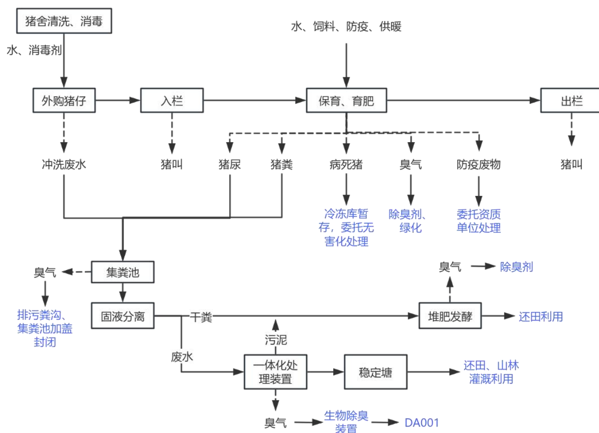
图 3.3-2 生猪养殖工艺流程图
