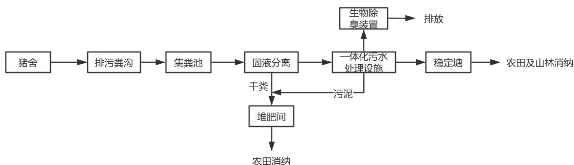
图 7.2-2 本项目粪污工艺基本流程
