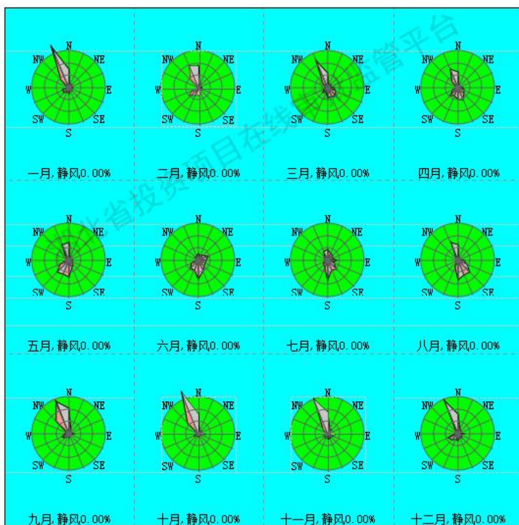
图 5.2-6 荆门地区 2022 年全年风频玫瑰图
