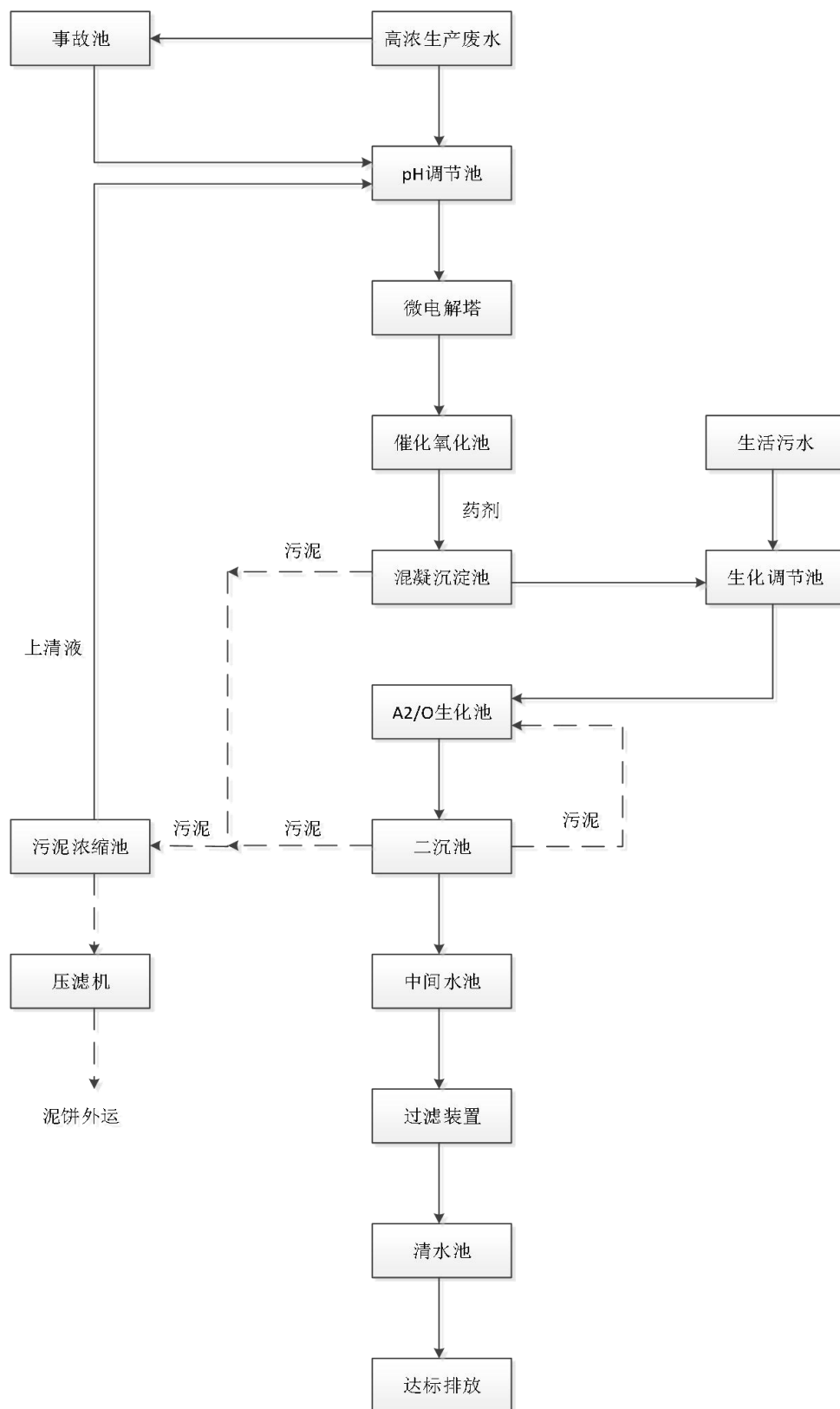
图 7.3-1 厂区废水处理工艺流程图
