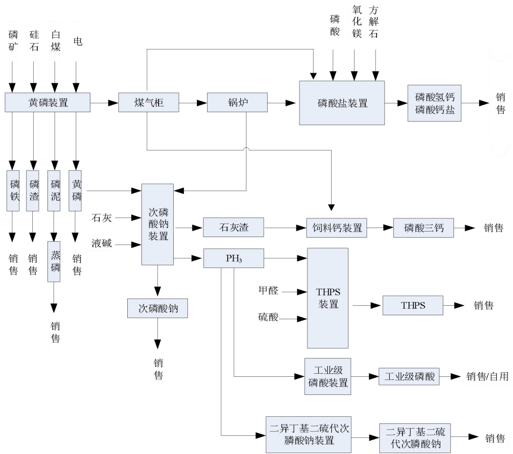
图2.1-1 湖北吉星化工集团有限责任公司全厂现有产品路线图
