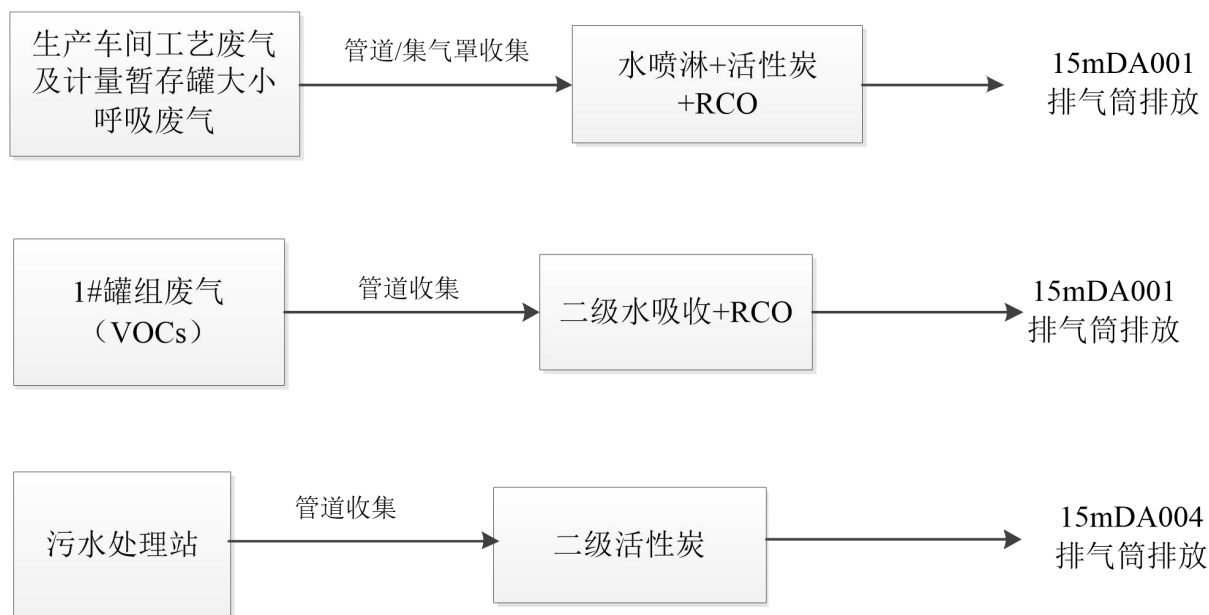
图 7.2-1 项目废气收集处理措施工艺流程图
