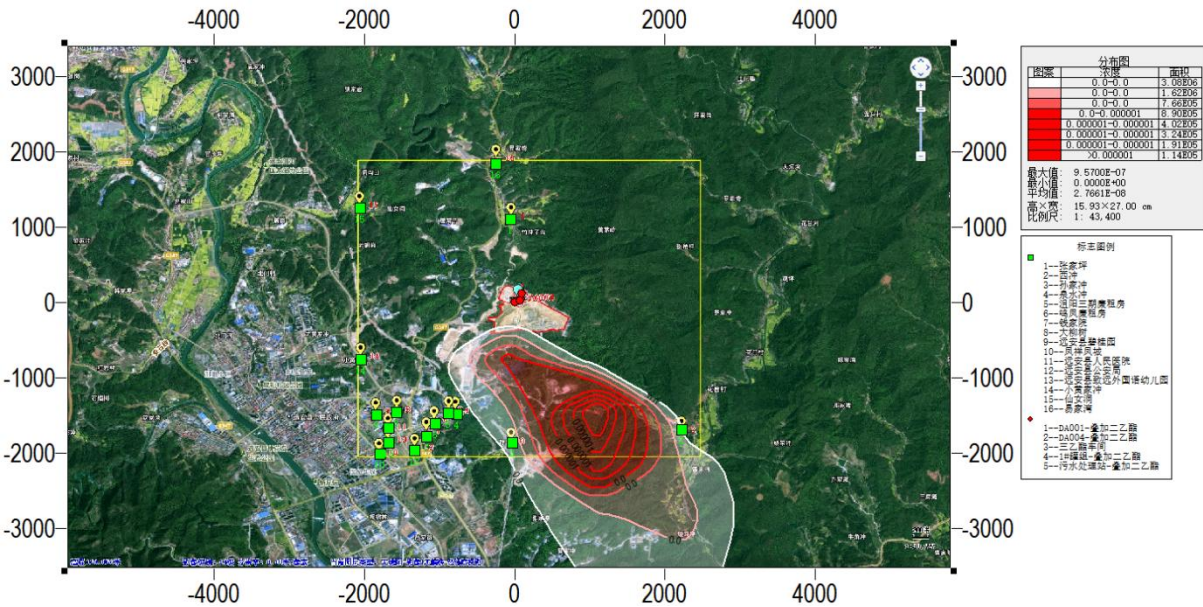
图 5.2-13 氨小时平均浓度最大贡献值浓度分布图（单位：mg/m³）
