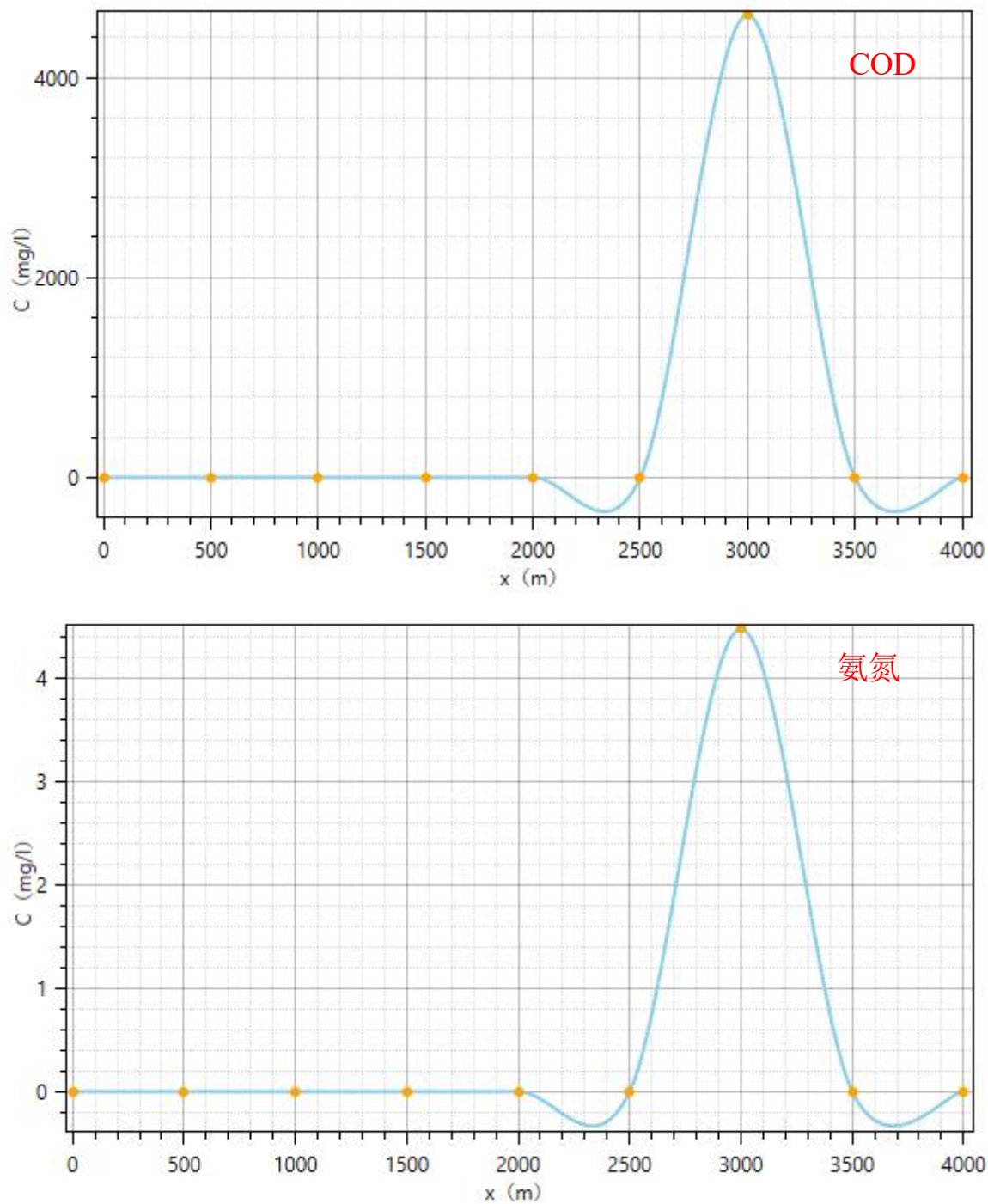
图 5.2-31 COD、氨氮 1000d 不同距离的预测结果变化趋势图
