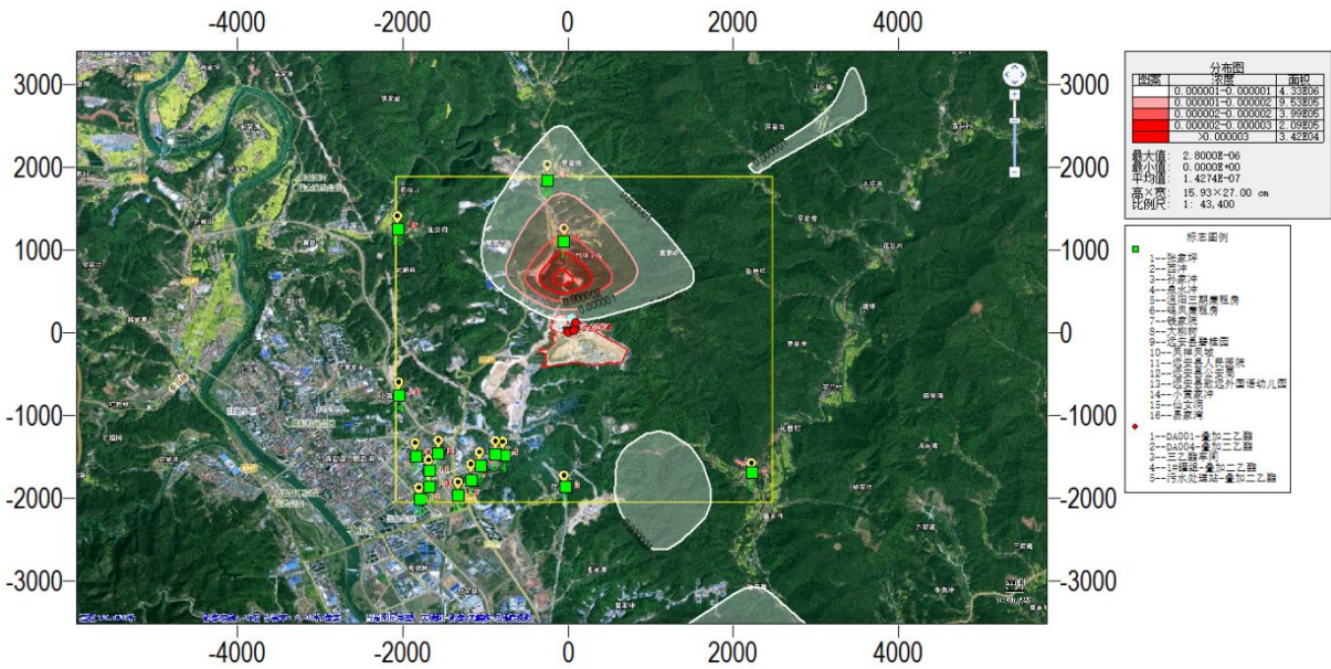
图 5.2-8 PM 10 日平均浓度最大贡献值浓度分布图（单位：mg/m 3 ）
