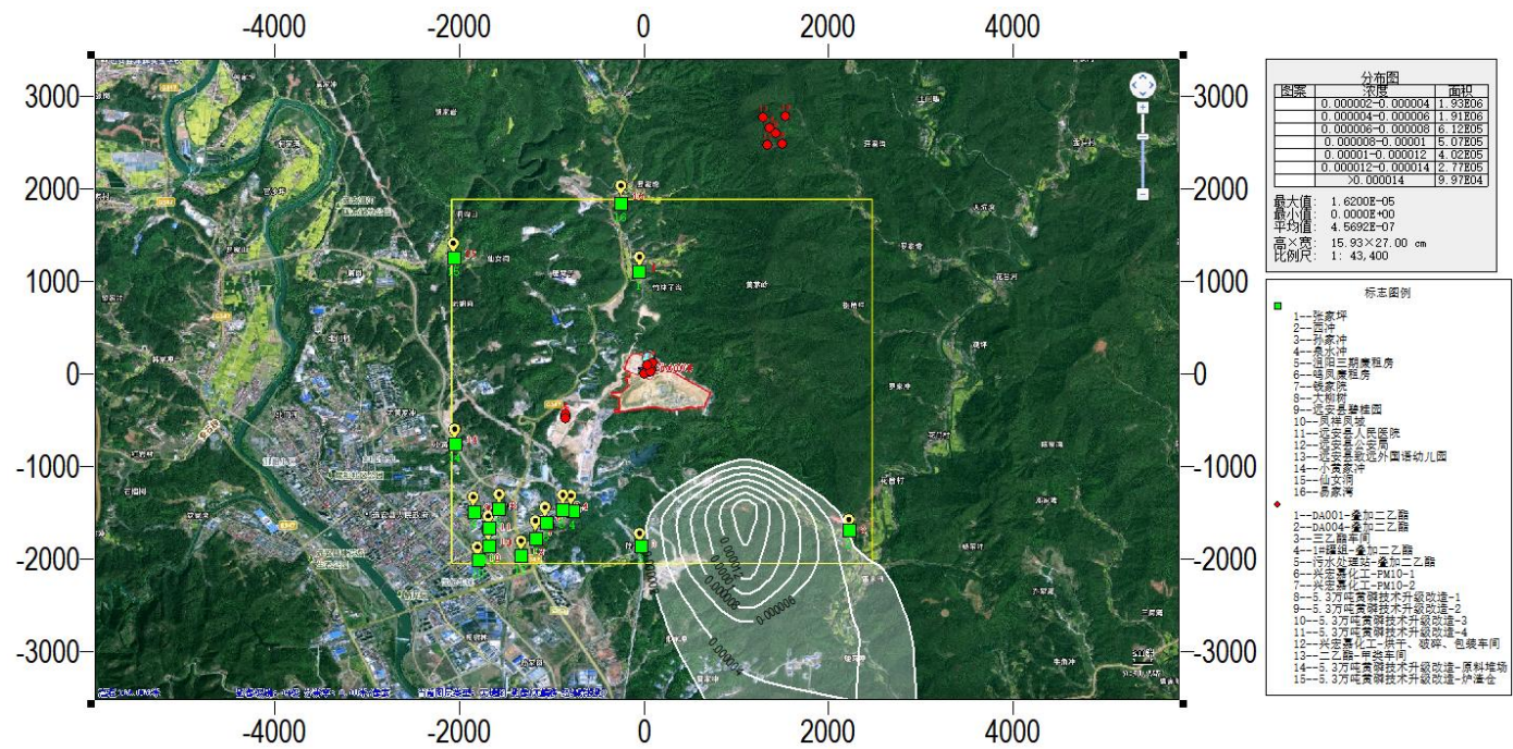
图 5.2-20 氨叠加后小时平均浓度分布图（单位：mg/m³）
