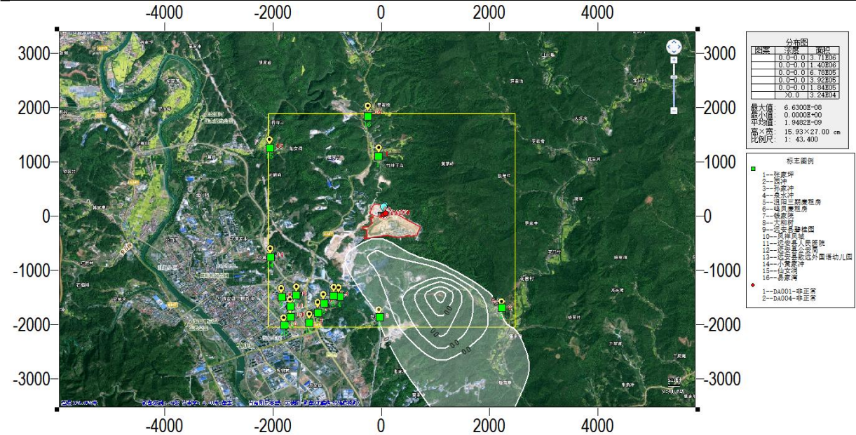
图 5.2-25 硫化氢非正常排放小时平均最大贡献值浓度分布图（单位：mg/m³）
