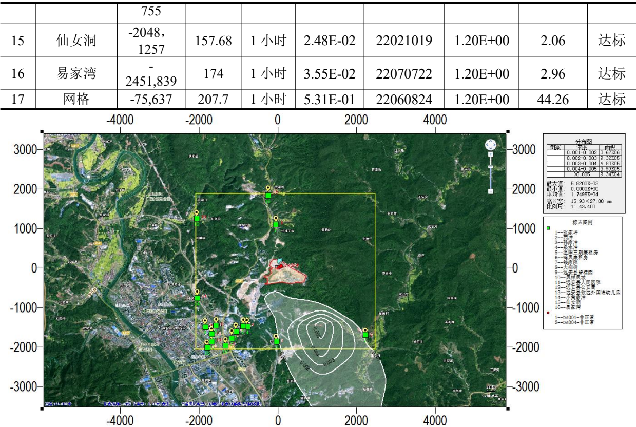
图 5.2-23 TVOC 非正常排放小时平均最大贡献值浓度分布图（单位：mg/m³）
