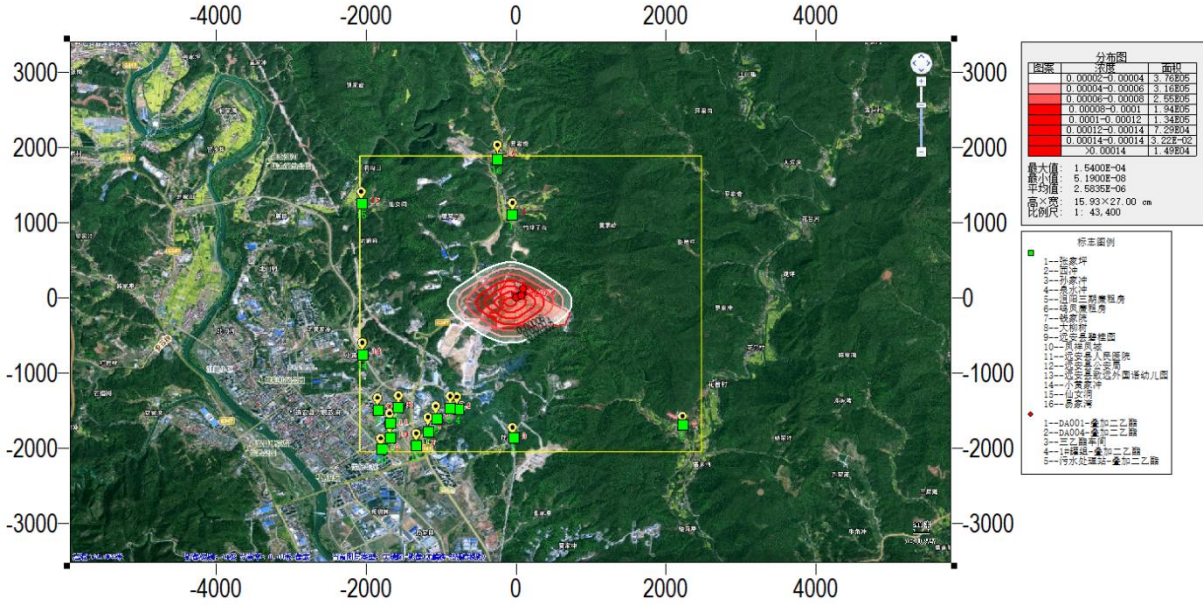
图 5.2-11 TSP 年平均浓度最大贡献值浓度分布图（单位：mg/m³）
