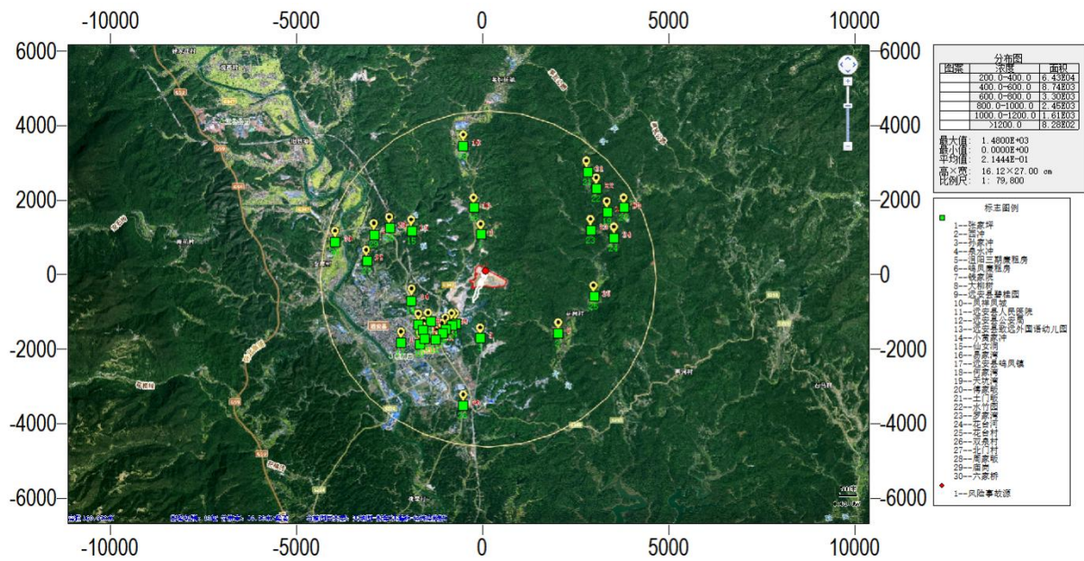
图 6.5-6 最不利气象条件下各网格点氯化氢浓度分布图 (mg/m³)
