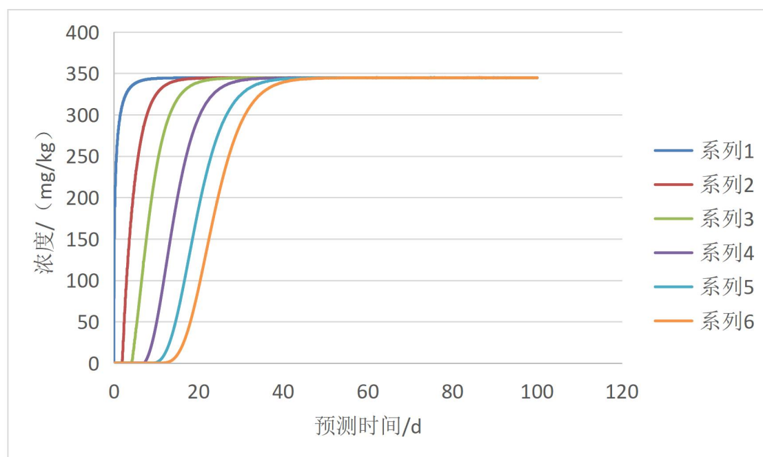
图 5.2-36 石油烃泄漏随时间在土壤中的迁移情况
