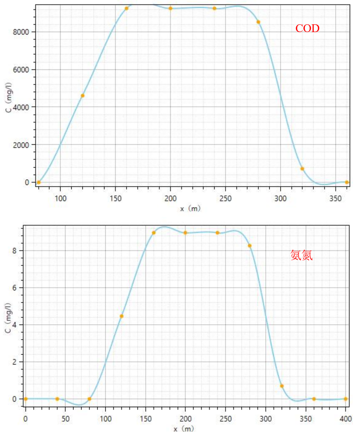
图 5.2-30 COD、氨氮 100d 随距离的预测结果变化趋势图
