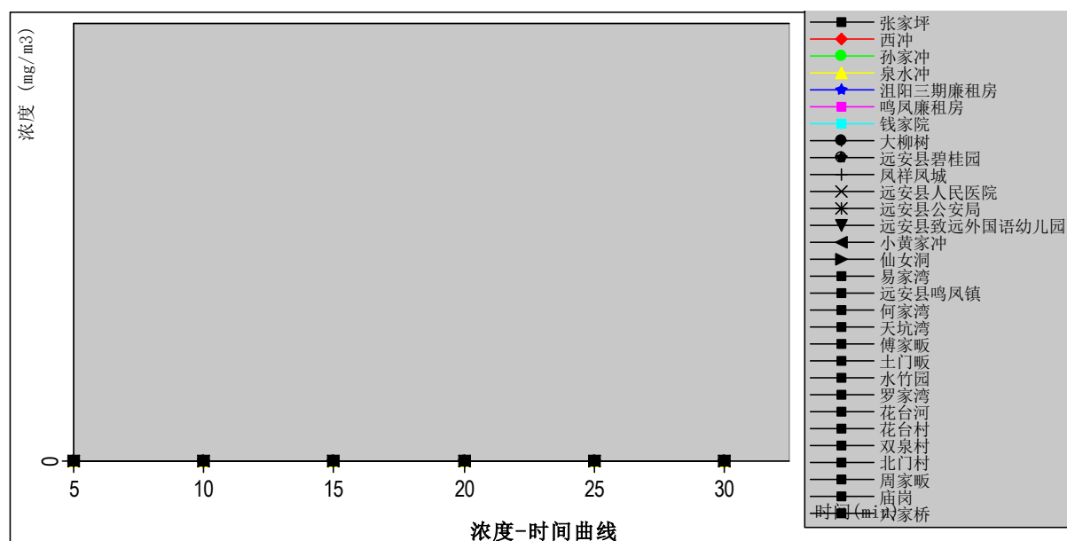
图 6.5-5 最不利气象条件下各关心点的氯化氢浓度随时间的变化图 ( \text{mg}/\text{m}^3 )
