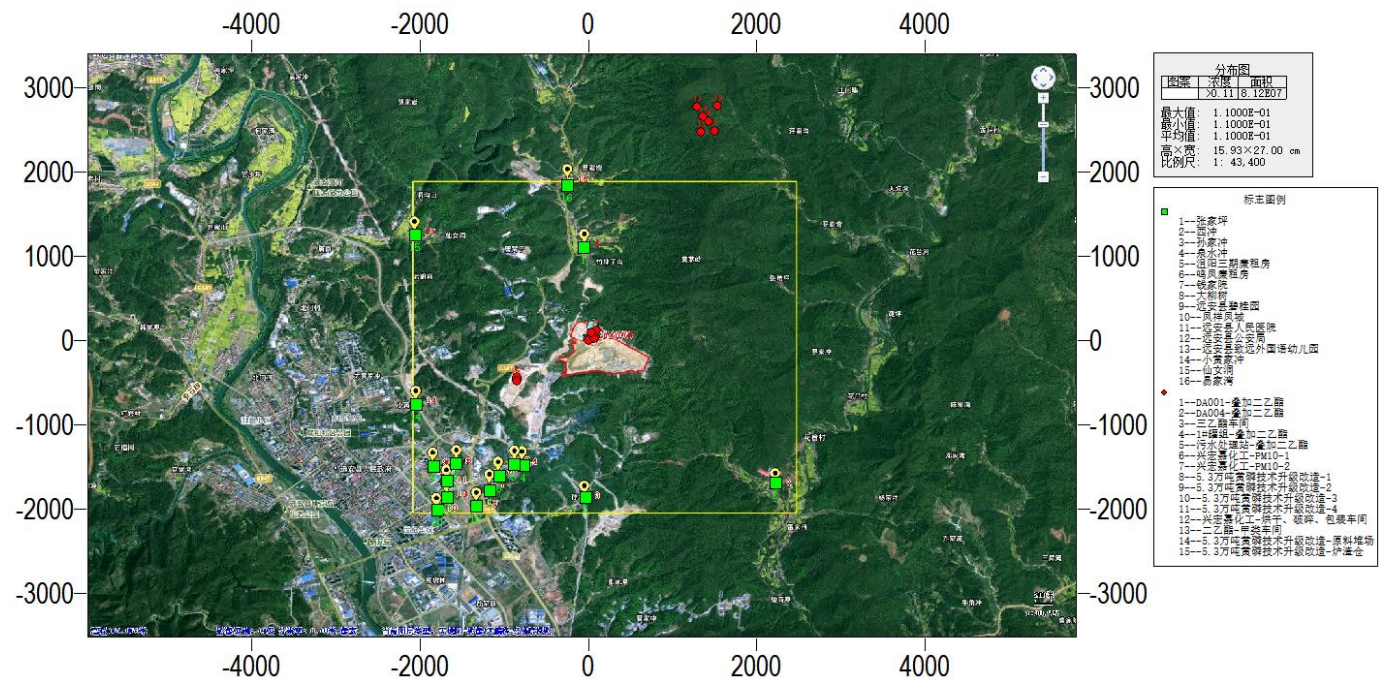
图 5.2-15 PM 10 叠加后日平均浓度分布图（单位：mg/m 3 ）
