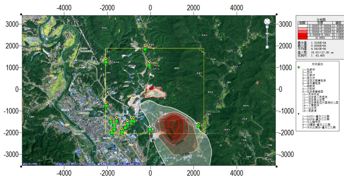
图 5.2-12 TVOC 小时平均浓度最大贡献值浓度分布图 (单位: \text{mg}/\text{m}^3 )
