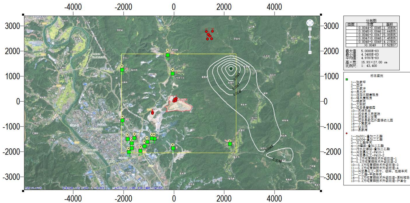
图 5.2-21 硫化氢叠加后小时平均浓度分布图（单位：mg/m³）
