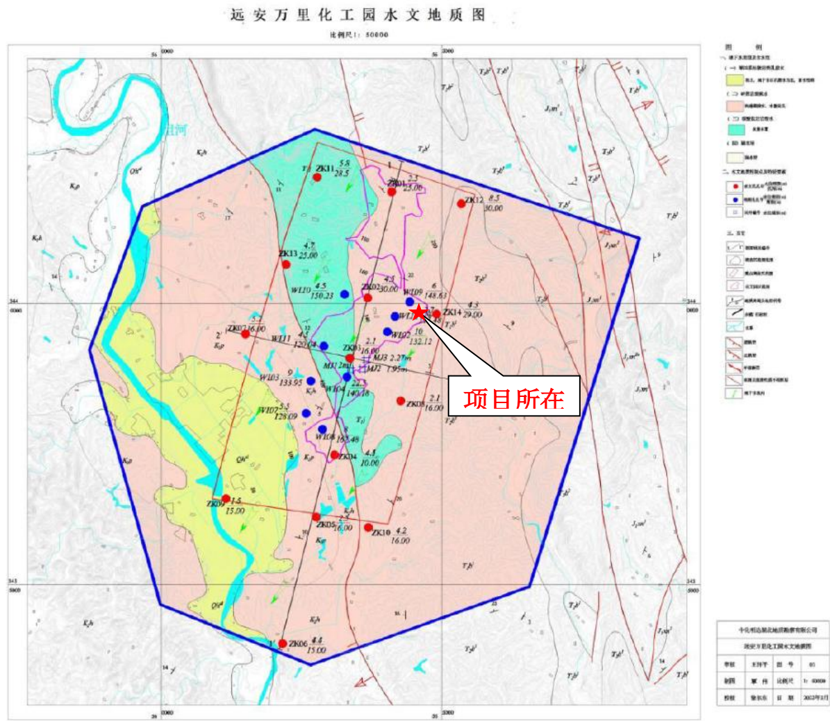
图 5.2-26 万里化工园水文地质图
