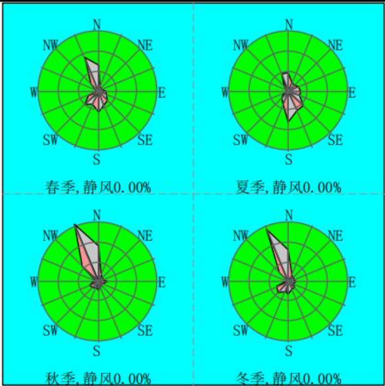
图 5.2-4 荆门地区 2022 年各季风频玫瑰图
