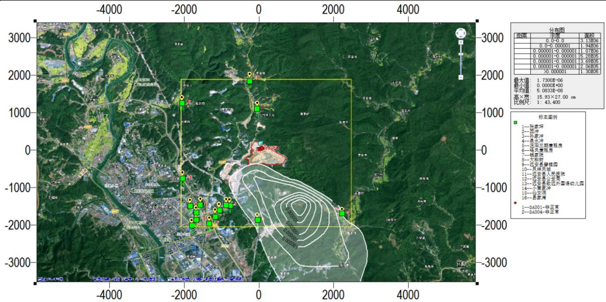
图 5.2-24 氨非正常排放小时平均最大贡献值浓度分布图（单位：mg/m³）
