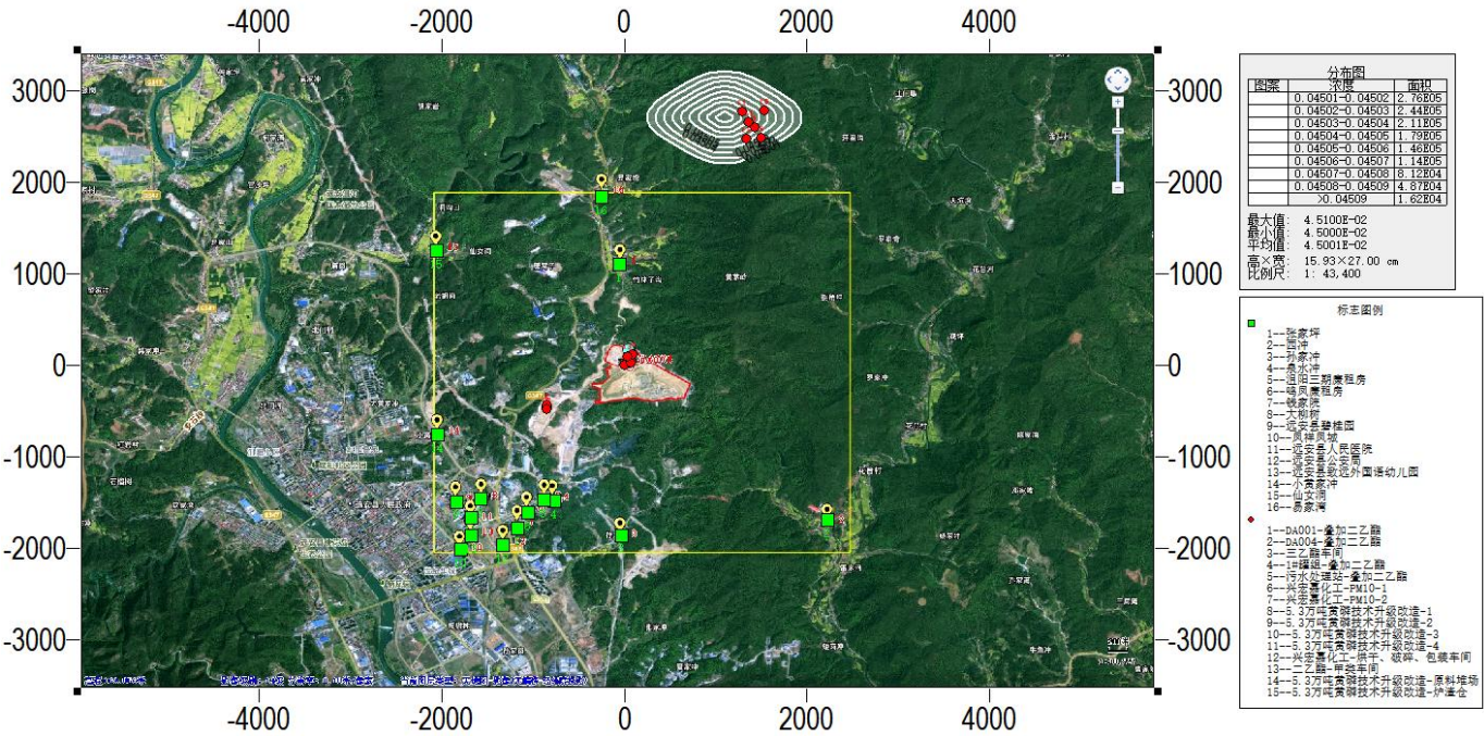
图 5.2-17 TSP 叠加后日平均浓度分布图 (单位: \text{mg}/\text{m}^3 )
