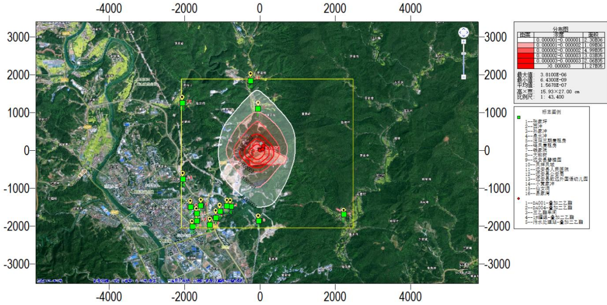
图 5.2-9 PM 10 年平均浓度最大贡献值浓度分布图（单位：mg/m 3 ）
