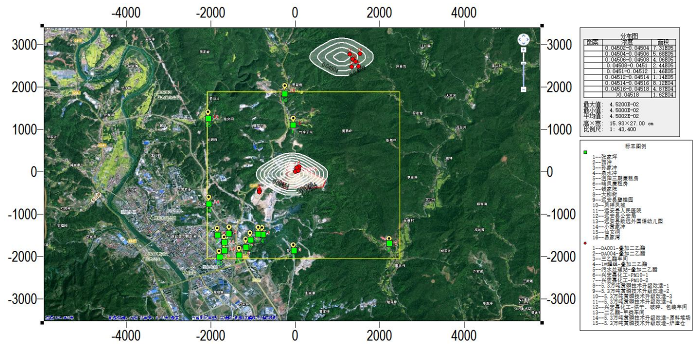
图 5.2-18 TSP 叠加后年平均浓度分布图
