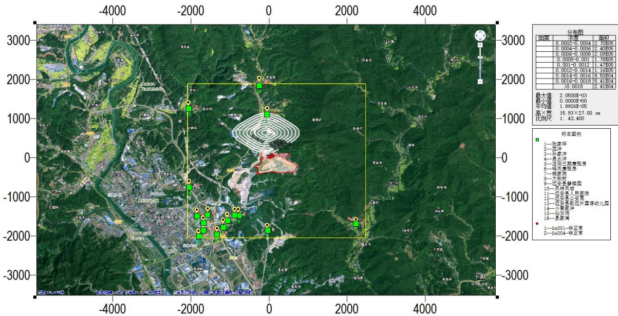
图 5.2-22 PM_{10} 非正常排放小时平均最大贡献值浓度分布图（单位： mg/m^3 ）
