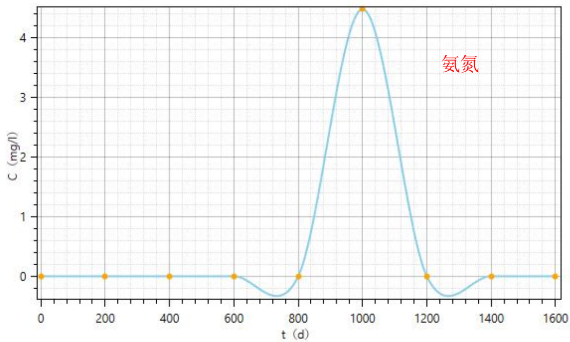
图 5.2-33 COD、氨氮 3000m 处不同时间的预测结果变化趋势
