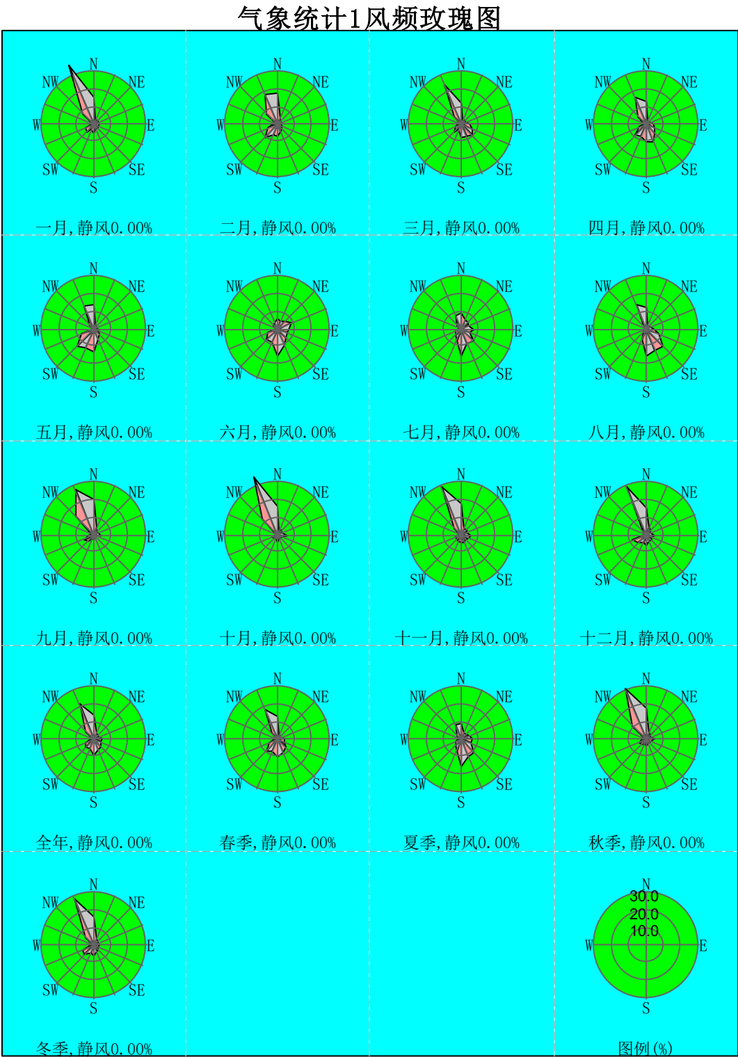
图 5.2-5 荆门地区 2022 年全年风频玫瑰图
