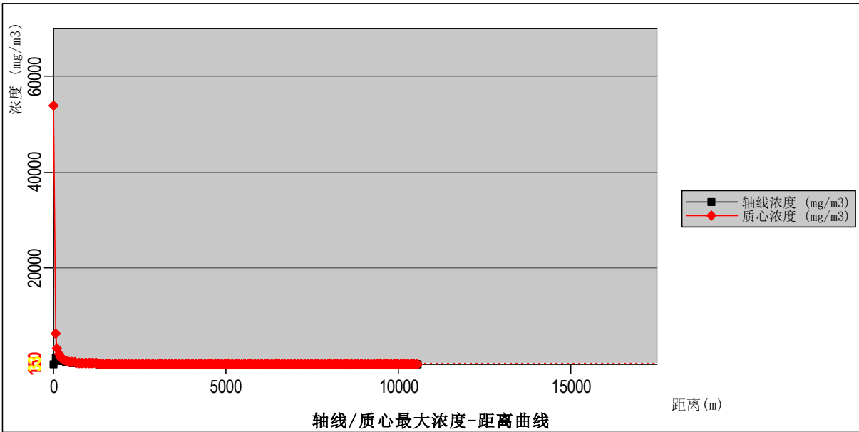
图 6.5-3 HCl 轴线/质心最大浓度图
