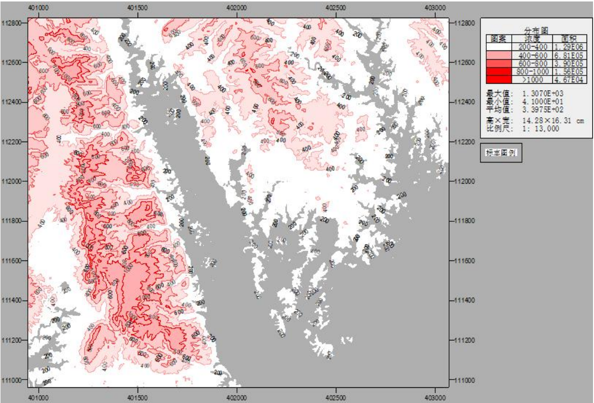
图 5.2-6 项目所在区域地形等高线示意图
