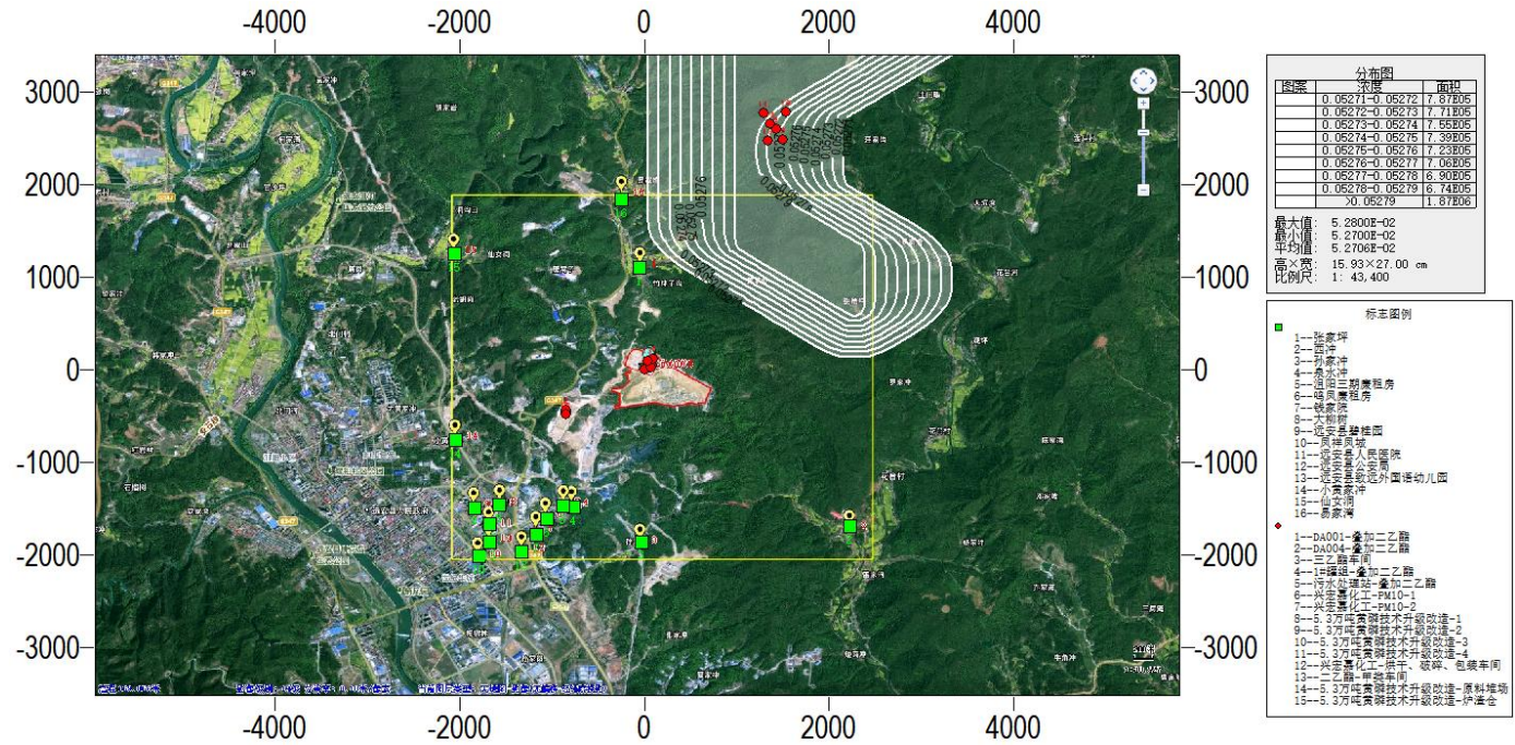
图 5.2-16 PM 10 叠加后年平均浓度分布图
