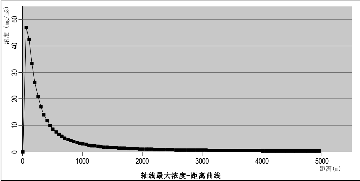
图 6.5-2 CO 预测轴线最大浓度图
