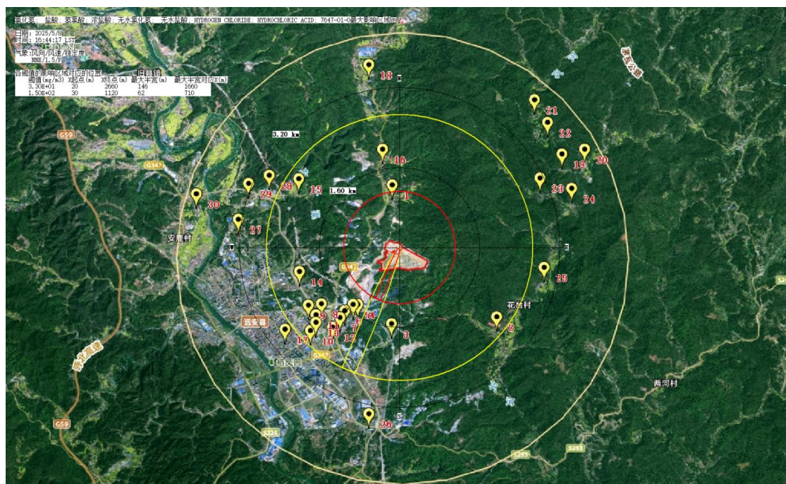
图 6.5-4 HCl 最大影响区域图
