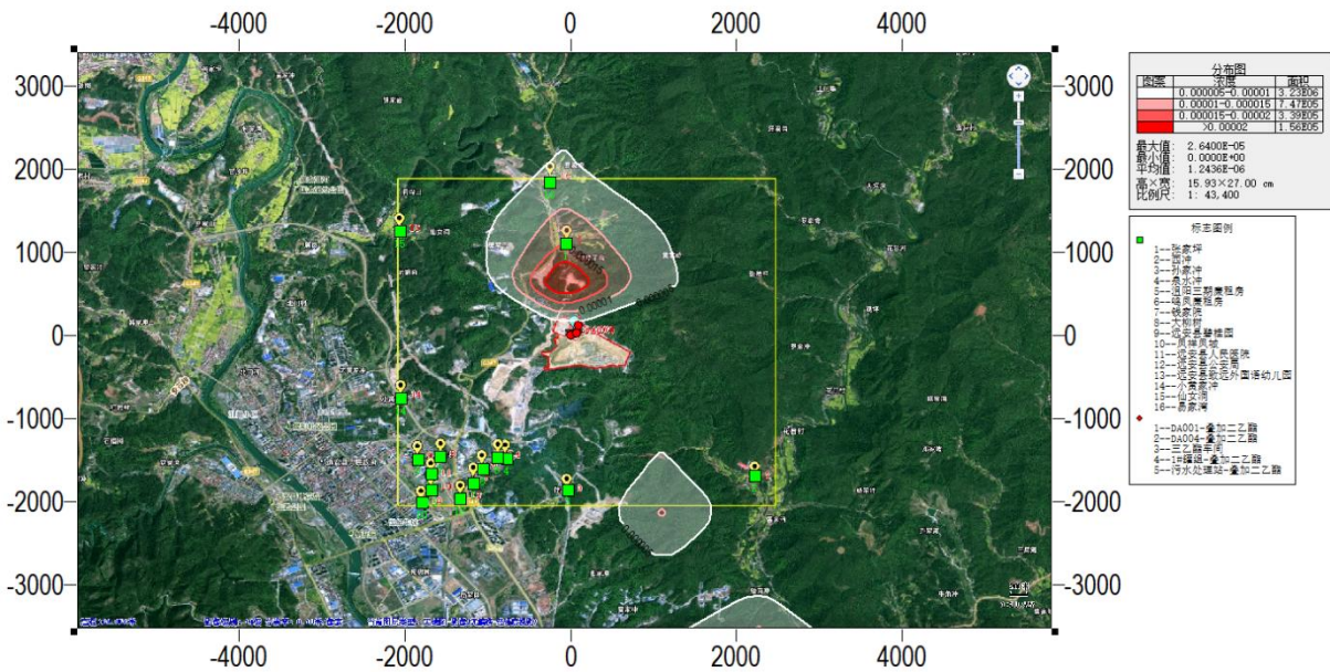
图 5.2-10 TSP 日平均浓度最大贡献值浓度分布图（单位：mg/m³）
