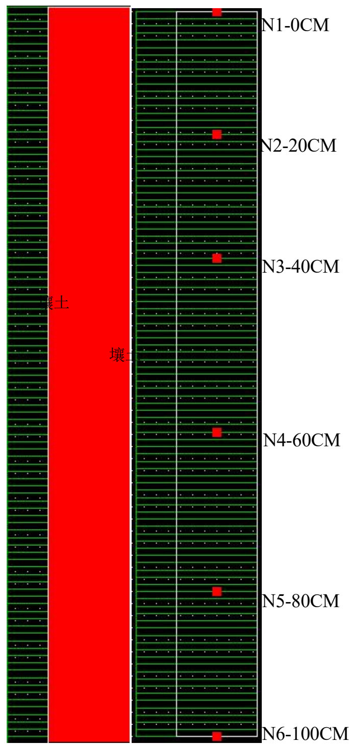
图 5.2-35 土壤结构模拟、观测点设置图
