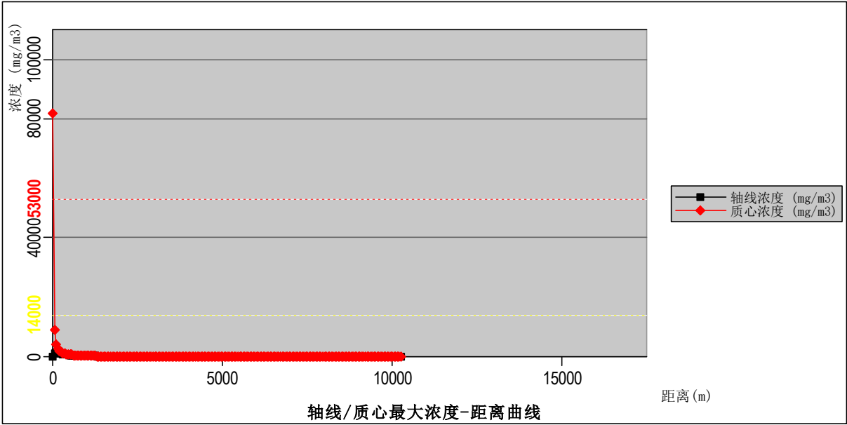
图 6.5-1 轴线/质心最大浓度图
