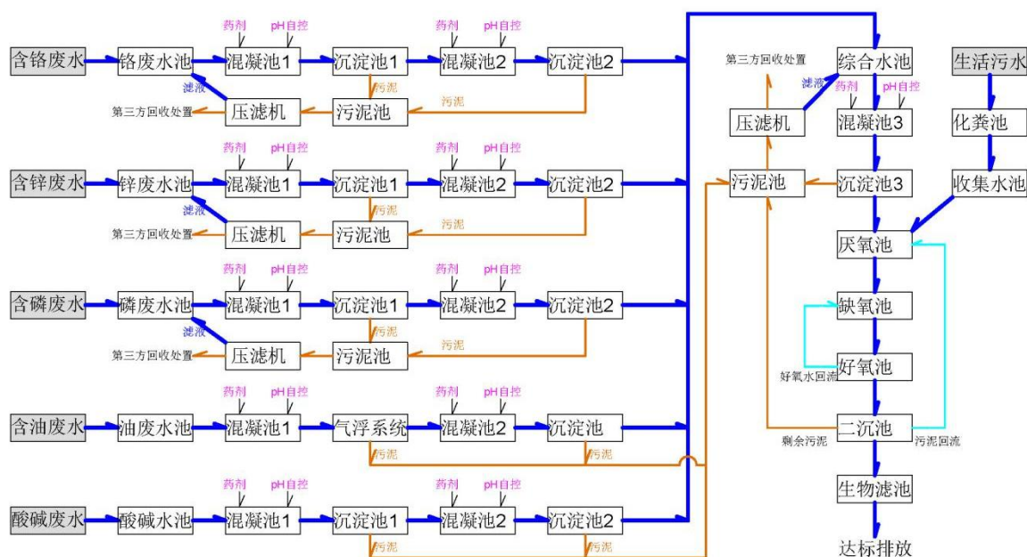
图 7.2-1 废水处理工艺流程图（含废水走向图）
