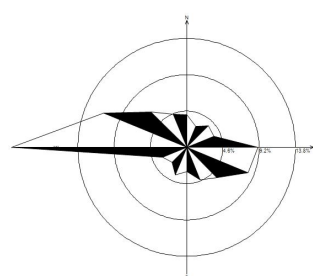
四月静风 0.56%
