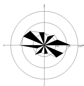
三月静风 0.94%
