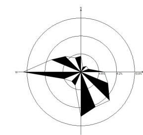
八月静风 1.21%
