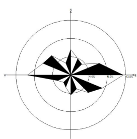
二月静风 2.44%
