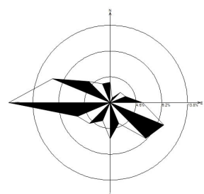
五月静风 0.94%
