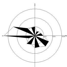
六月静风 2.78%
