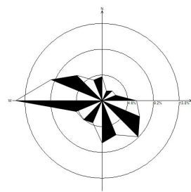
夏季静风 2.26%
