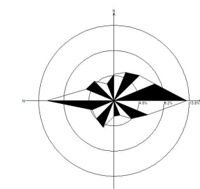
十二月静风 0.67%
