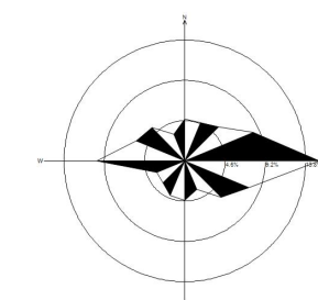
冬季静风 3.11%
