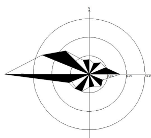
秋季静风 2.56%
