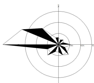
九月静风 1.81%
