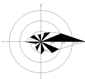
一月静风 2.55%
