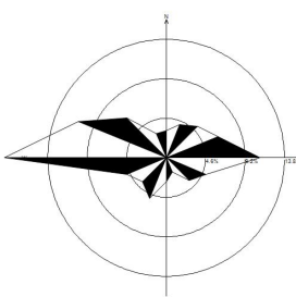
十一月静风 3.06%
