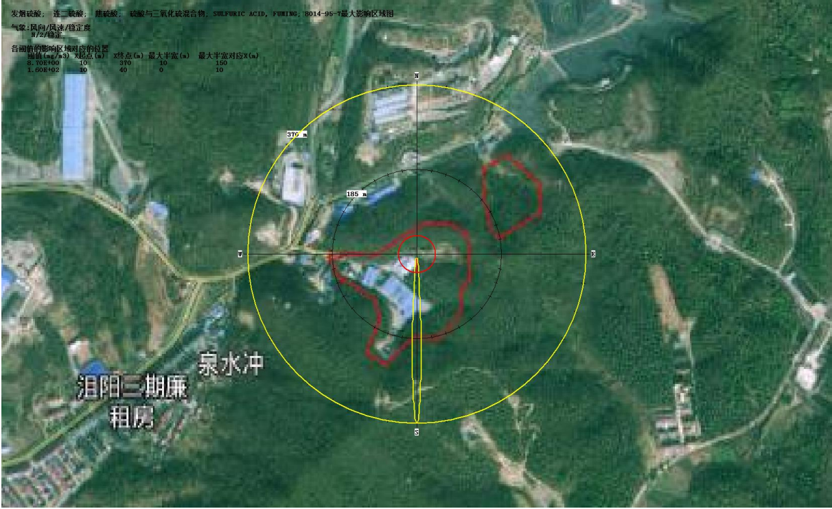
图 8.6.1.6.1-1 硫酸储罐泄漏扩散环境风险预测结果图
