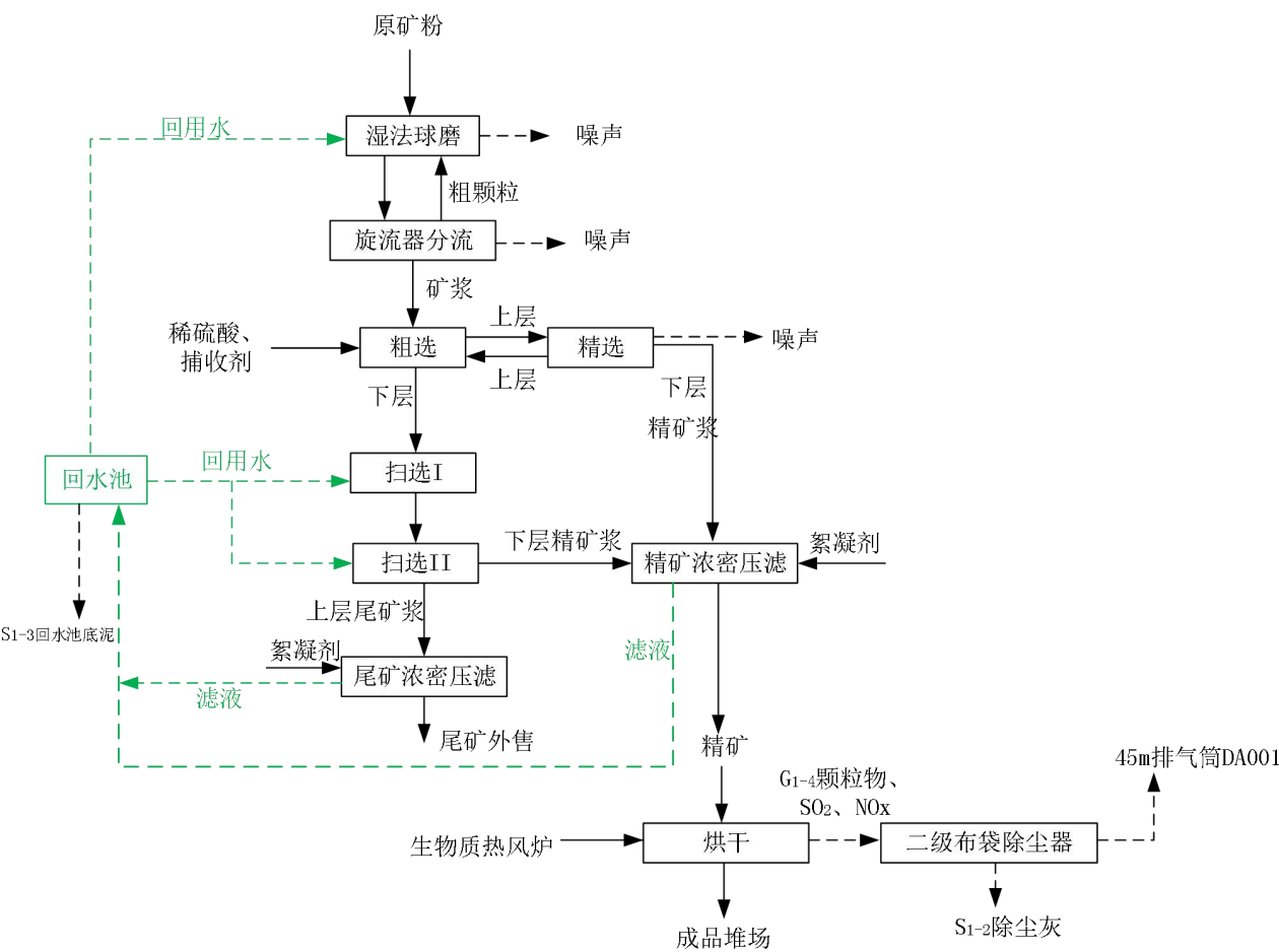
图 3.6-1 选矿工艺流程及产污环节图
