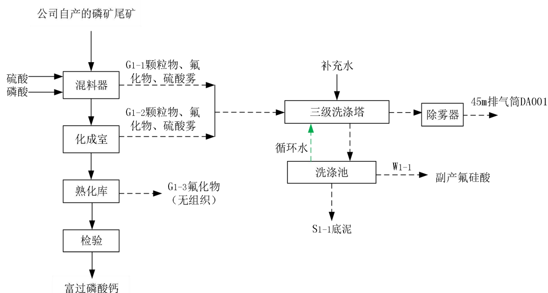
图 3.5-1 富钙工艺流程及产污示意图
