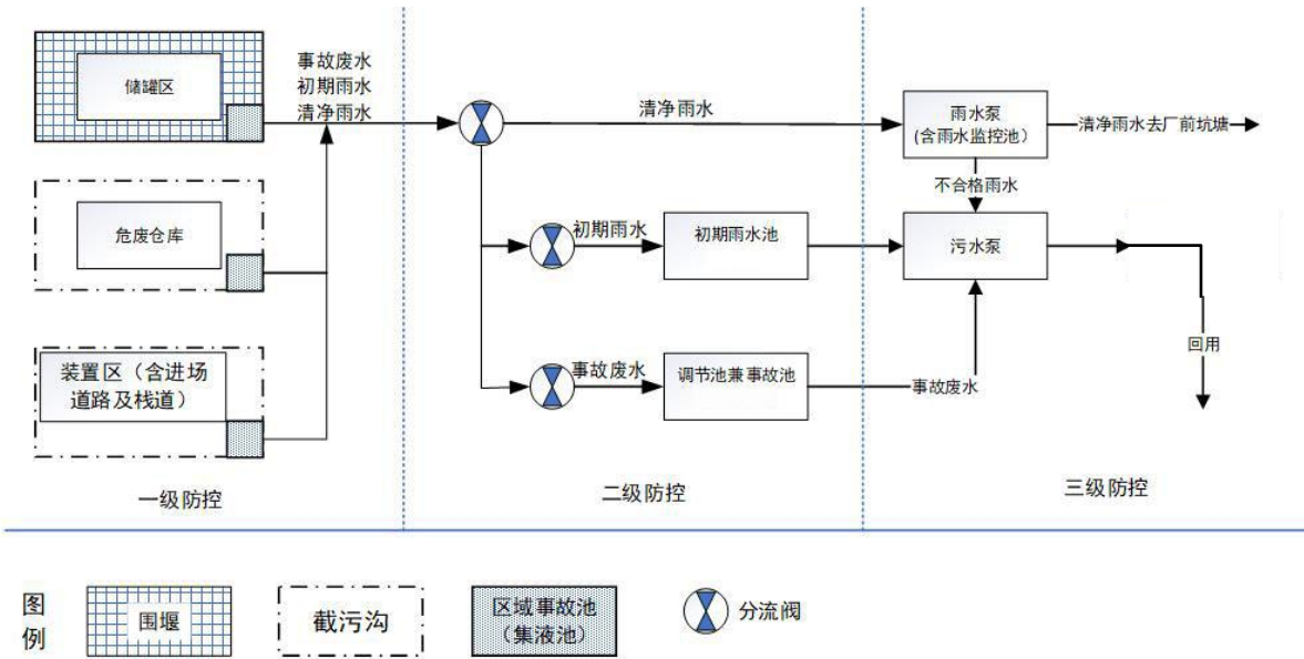
图 8.7.4-1 事故废水三级防控设施示意图
