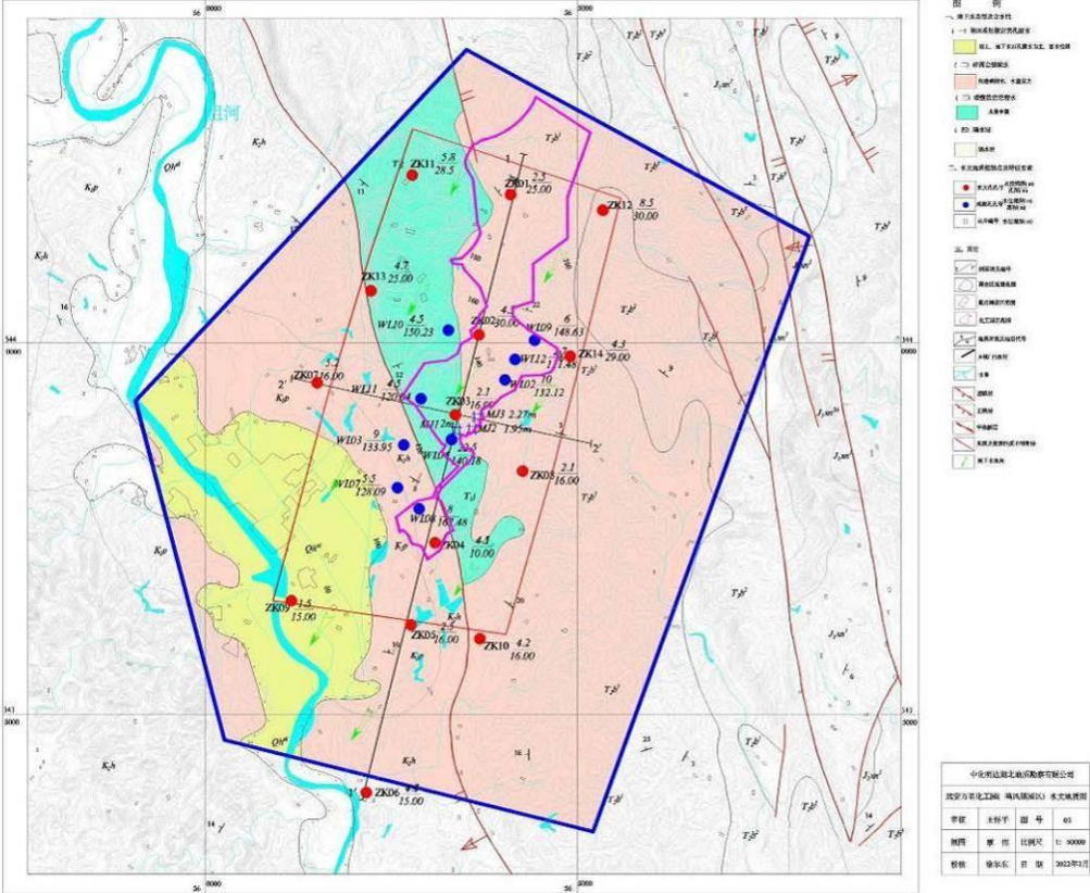
图 6.1.6.4-1 远安化工园（万里片区）水文地质图
