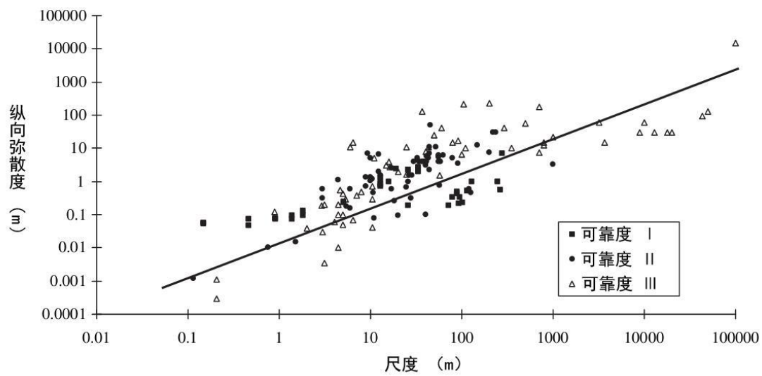
图 7.2.5.3.2-1 松散沉积物的弥散度确定
