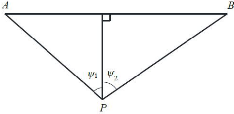
图 7.2.3.2-1 有限路段的修正函数，A--B 为路段，P 为预测点
