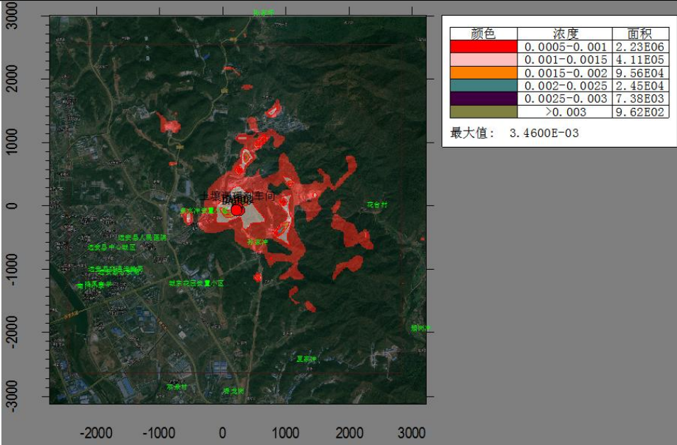
图 7.2.1.11-7 正常工况项目废气对敏感目标及网格浓度预测结果等值线图（PM 10 日均值）
