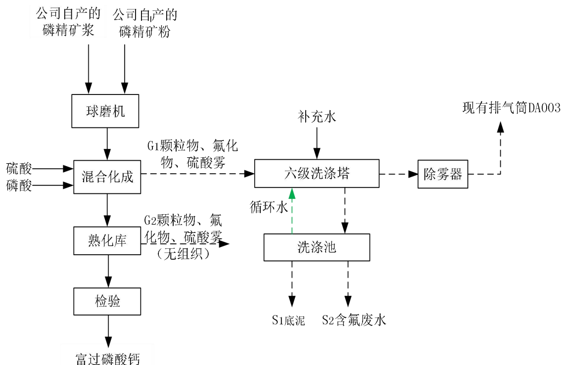
图 5.1-1 富钙工艺流程及产污示意图
