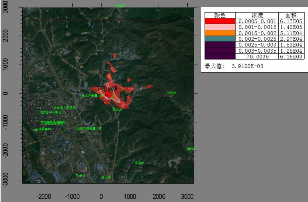
图 7.2.1.11-11 正常工况项目废气对敏感目标及网格浓度预测结果等值线图（硫酸雾小时均值）
