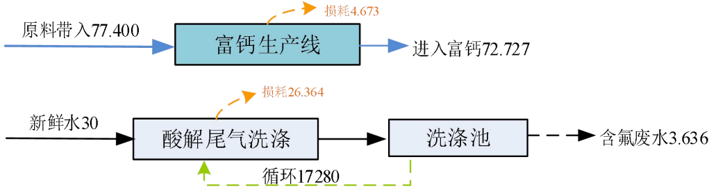
图 5.2.2-4 项目水平衡图 ( \text{m}^3/\text{d} )
