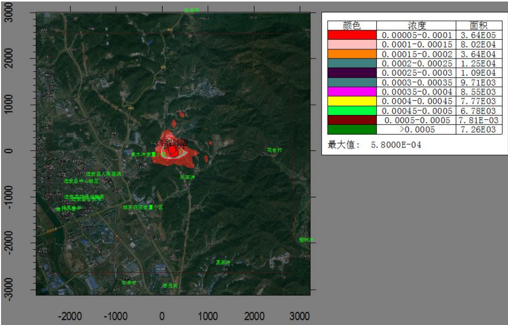
图 7.2.1.11-12 正常工况项目废气对敏感目标及网格浓度预测结果等值线图（硫酸雾日均值）
