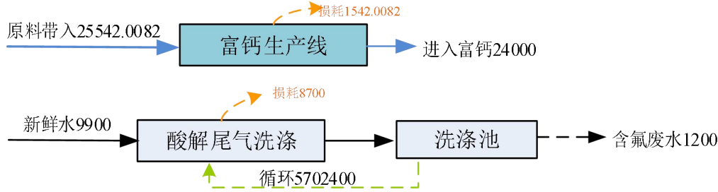
图 5.2.2-5 项目水平衡图 ( \text{m}^3/\text{a} )
