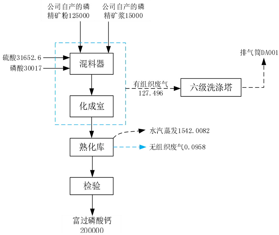
图 5.2.1-1 富钙物料平衡图
