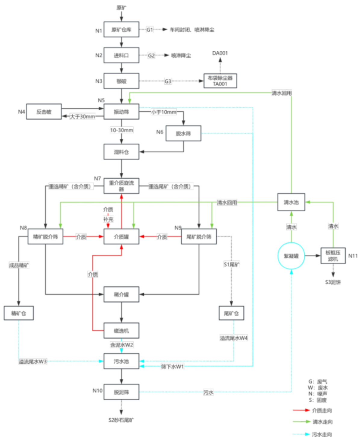
图 4.3-2 生产工艺图
