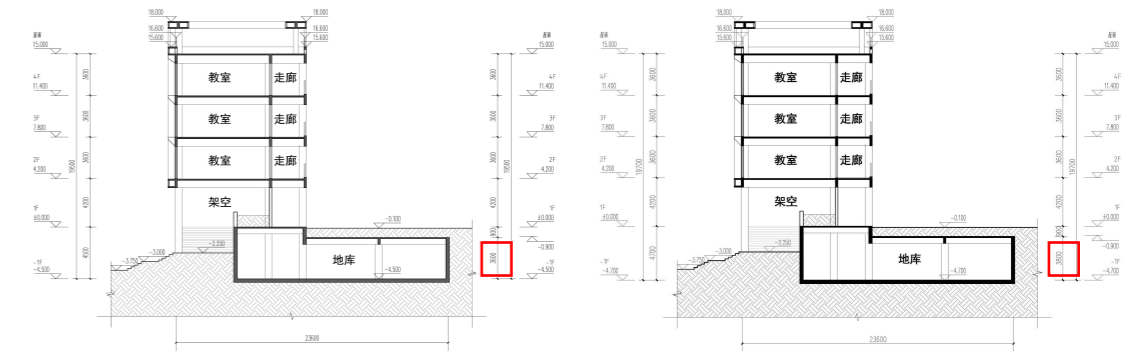
地下室变更前剖面图
