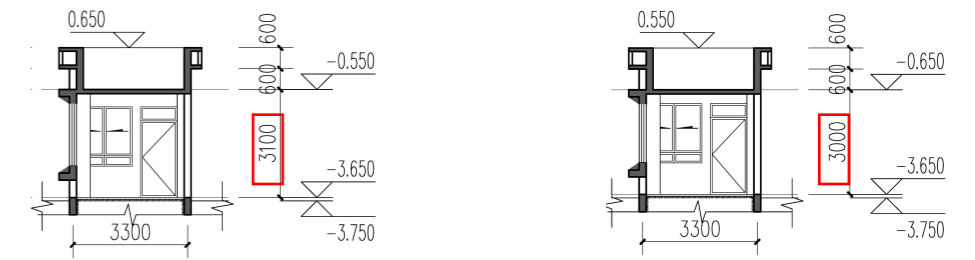
门房变更前剖面图
